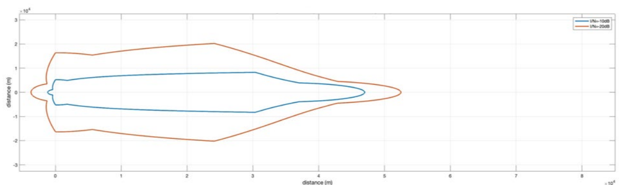
参考図 6.3-20 Pattern2-1 (電波法関係審査基準, VLP, 25mW, Outdoor, Body Loss なし)
