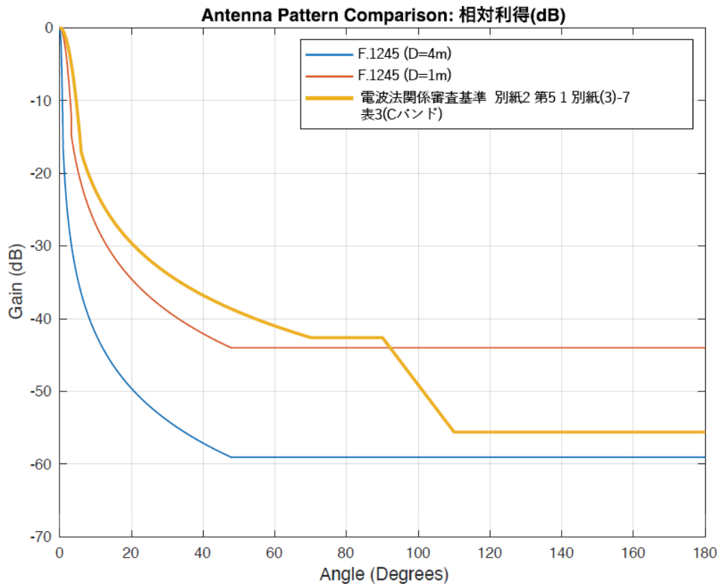
図 6.3-70 アンテナパターンの比較
