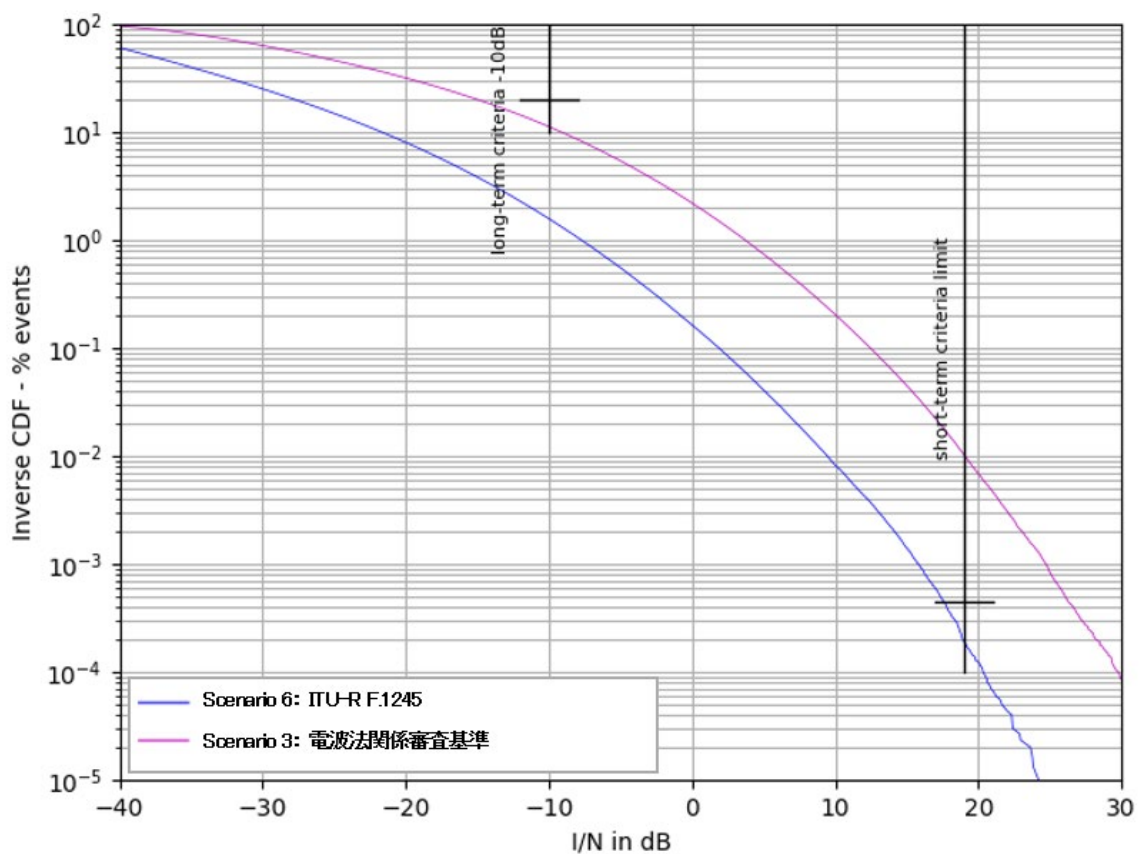
図 6.3-36 被干渉アンテナ地上高 20m の場合の結果（シナリオ 3, 6）
