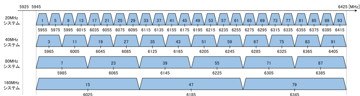
図 7.1-1 6GHz帯無線LANシステムの周波数チャネル配置
