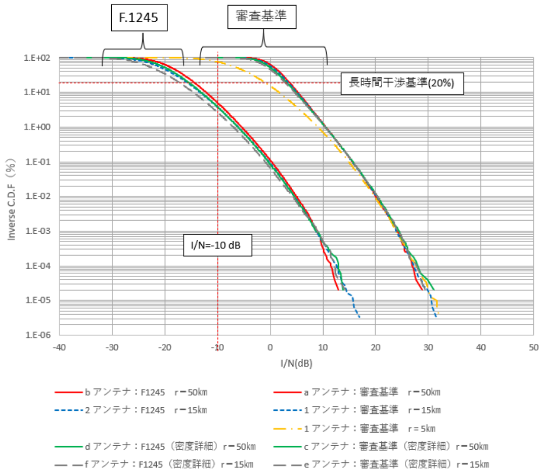
図 6. 3-72 電波法関係審査基準及び Rec. ITU-R F. 1245 の計算半径比較
