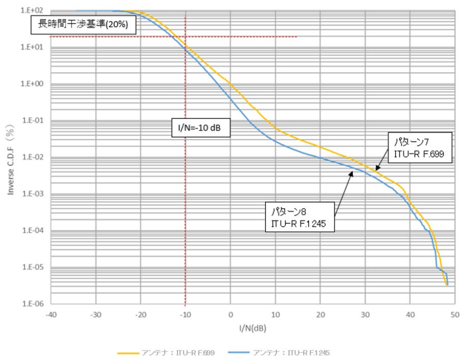
図 6.3-69 FPU パターン 7、8
