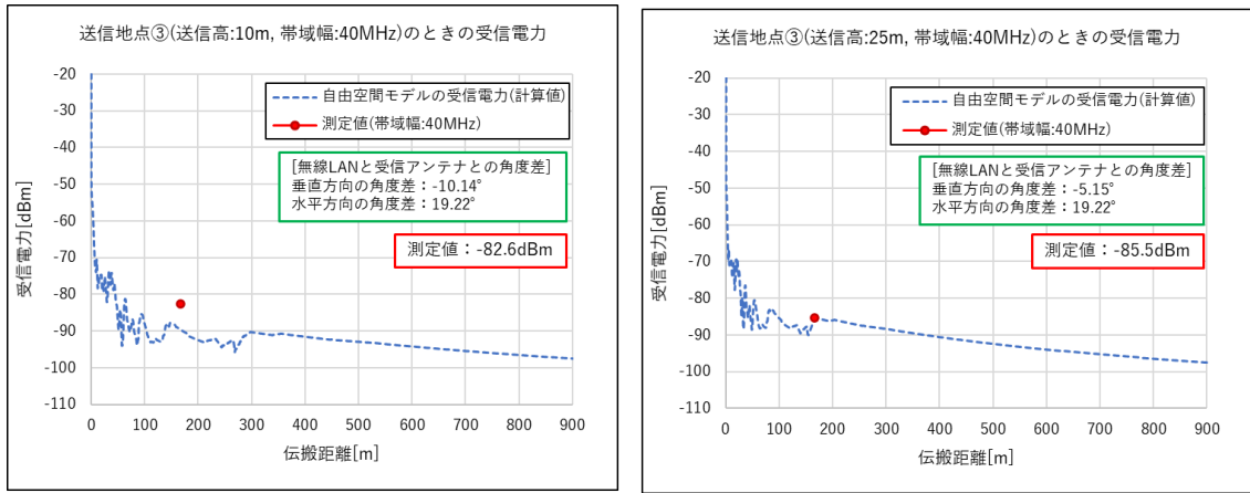
図 6.3-87 測定結果と理論値との比較 送信地点③(カテゴリ C)
