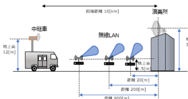
図 6.3-52 映像 FPU(固定)：中継車→演奏所の条件と所要改善量
