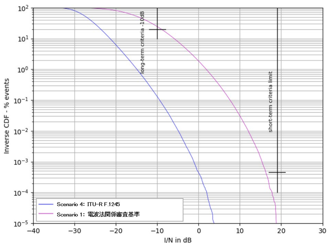
図 6.3-14 被干渉アンテナ地上高 110m の場合の結果 (シナリオ 1, 4)
