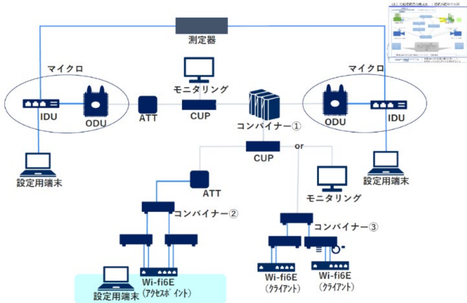
図 6.3-39 屋内実証試験の構成
