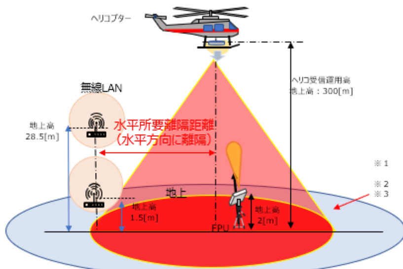
図 6.3-55 映像 FPU(移動) : 地上→ヘリコプター(rural)の条件
