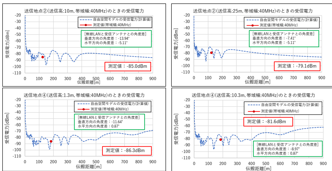
図 6.3-86 測定結果と理論値との比較 送信地点②④(カテゴリ B)
