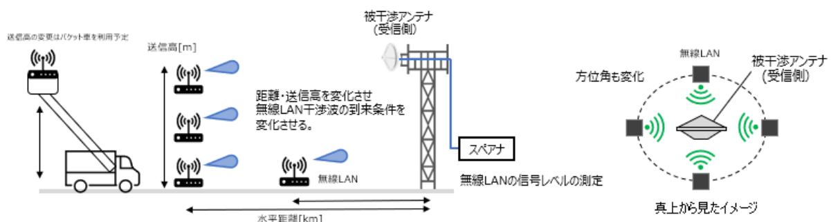
図 6.3-83 試験システムイメージ
