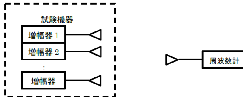
図 7.2-1 占有周波数帯幅測定系統図（空中線端子なしの場合）
