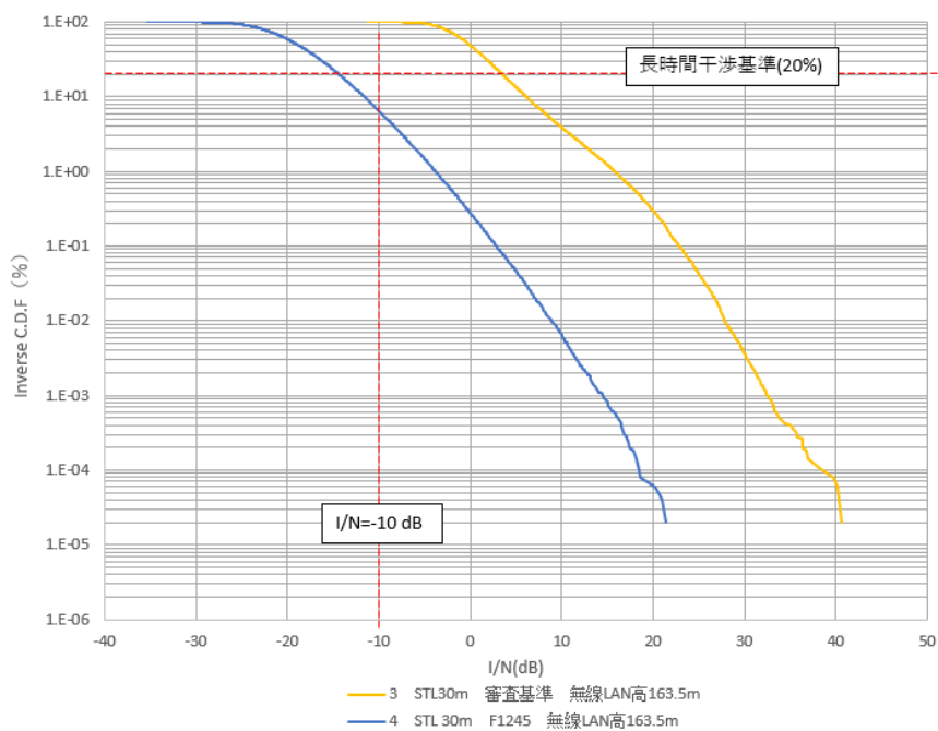
(2) 映像STLのシミュレーション結果（受信高30m）
