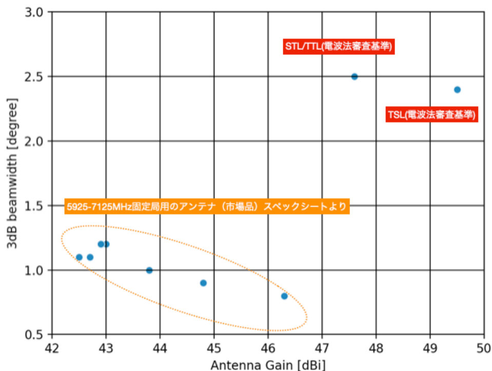
図 6.3-71 アンテナ最大利得と半値角の比較
