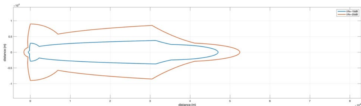
参考図 6.3-29 Pattern2-1（電波法関係審査基準, VLP, 25mW, Outdoor, Body Loss なし）
