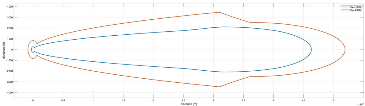
参考図 6.3-8 Pattern2-1 (電波法関係審査基準, VLP, 25mW, Outdoor, Body Loss なし)
