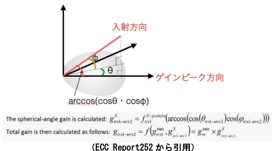
図 6.3-2 アンテナ利得の算出
