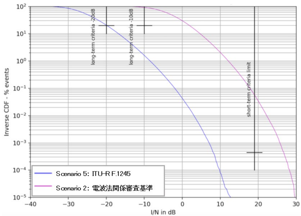
参考図 6.3-26 被干渉アンテナ地上高 55m の場合の結果（シナリオ 2, 5）
