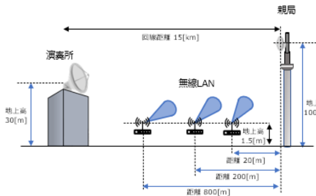
図 6.3-50 映像 STL：演奏所→親局の条件と所要改善量
