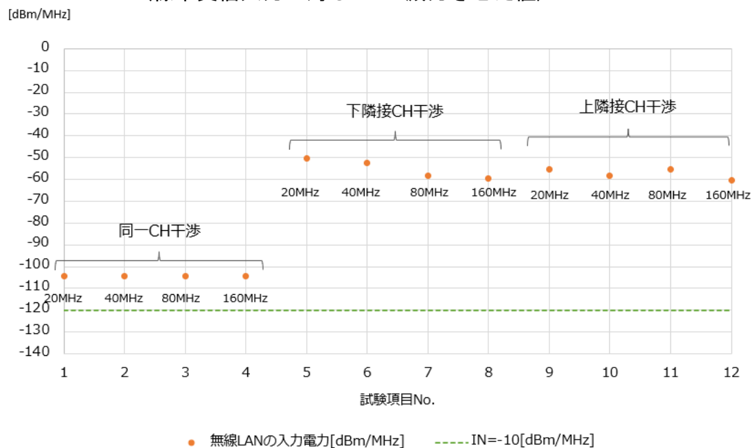
図 6.3-77 -70dBm 試験の結果
