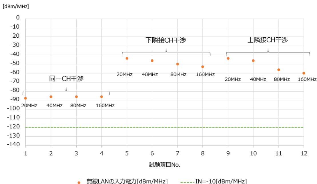
図 6.3-79 -65.5dBm(標準受信入力)試験の結果
