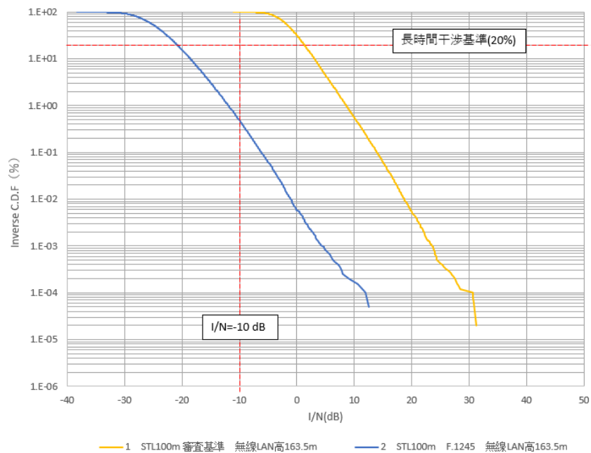
(1) 映像STLのシミュレーション結果（受信高100m）
