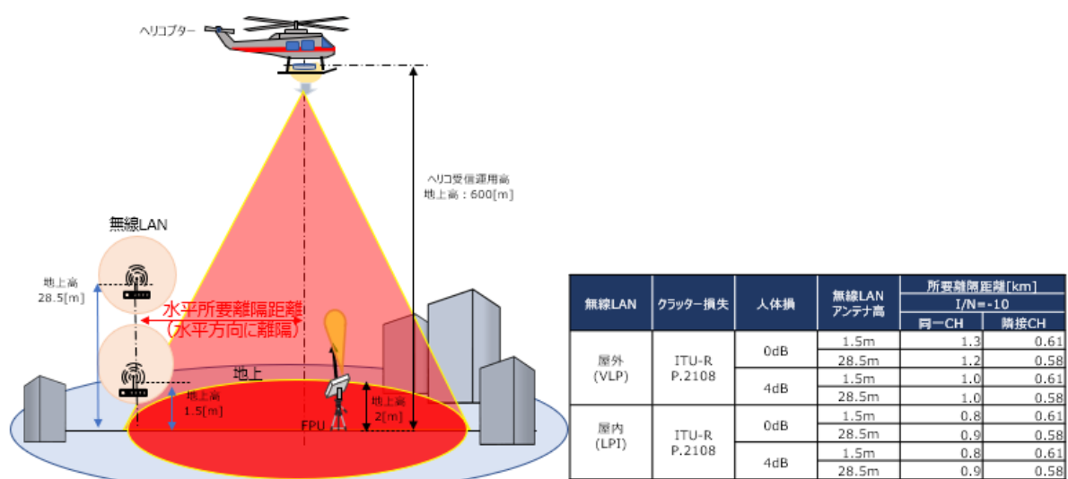
図 6.3-57 映像 FPU(移動) : 地上→ヘリコプター (urban) の条件と所要離隔距離
