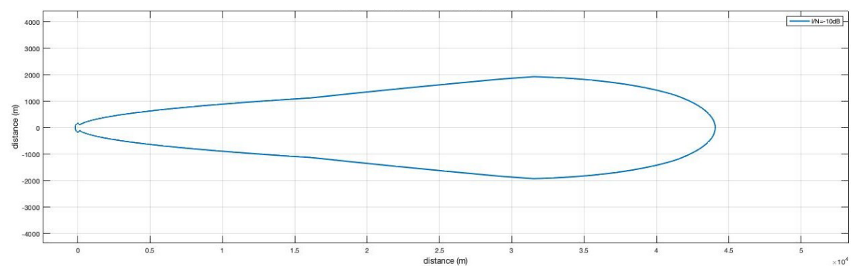
図 6.3-9 Pattern3-1 (電波法関係審査基準, VLP, 25mW, Outdoor, Body Loss あり)
