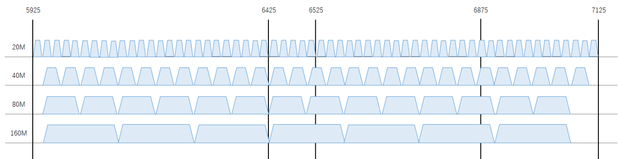
図 5.1-1 6GHz 帯無線 LAN システムのチャネル配置
