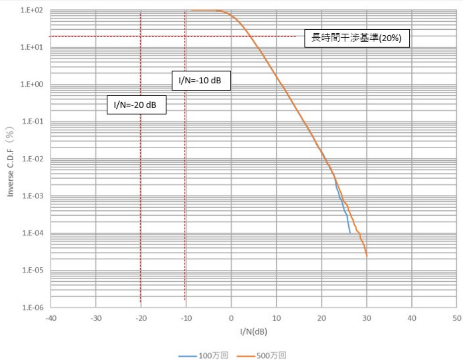
参考図 6.3-67 映像 TSL パターン 5
