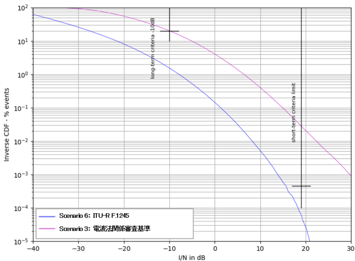
図 6.3-27 被干渉アンテナ地上高 25m の場合の結果（シナリオ 3, 6）
