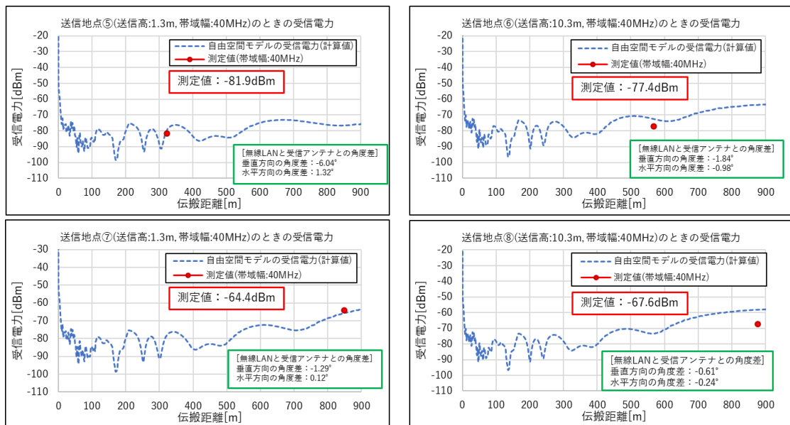
図 6.3-88 測定結果と理論値との比較 送信地点⑤⑥⑦⑧(カテゴリ D)
