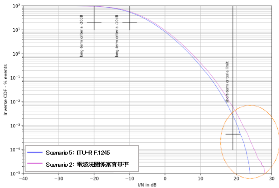
参考図 6.3-17 与干渉アンテナ地上高分布の変化に伴う結果の比較
