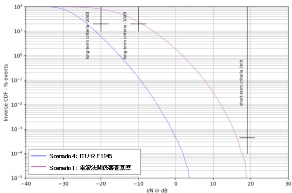
参考図 6.3-14 被干渉アンテナ地上高 110m の場合の結果（シナリオ 1, 4）
