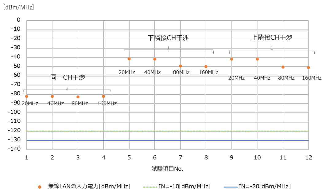
参考図 6.3-78 -54.5dBm(標準受信入力)試験の結果
