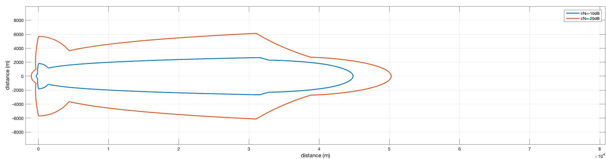
参考図 6.3-30 Pattern3-1 (電波法関係審査基準, VLP, 25mW, Outdoor, Body Loss あり)
