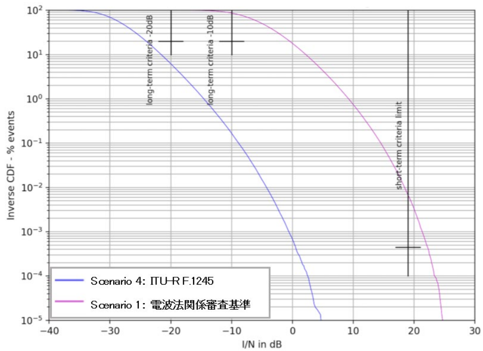
参考図 6.3-25 被干渉アンテナ地上高 110m の場合の結果（シナリオ 1, 4）
