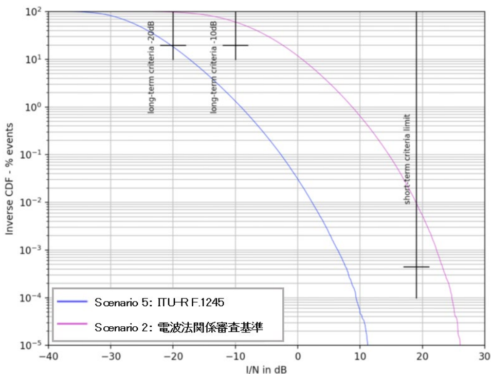
参考図 6.3-35 被干渉アンテナ地上高 55m の場合の結果 (シナリオ 2, 5)
