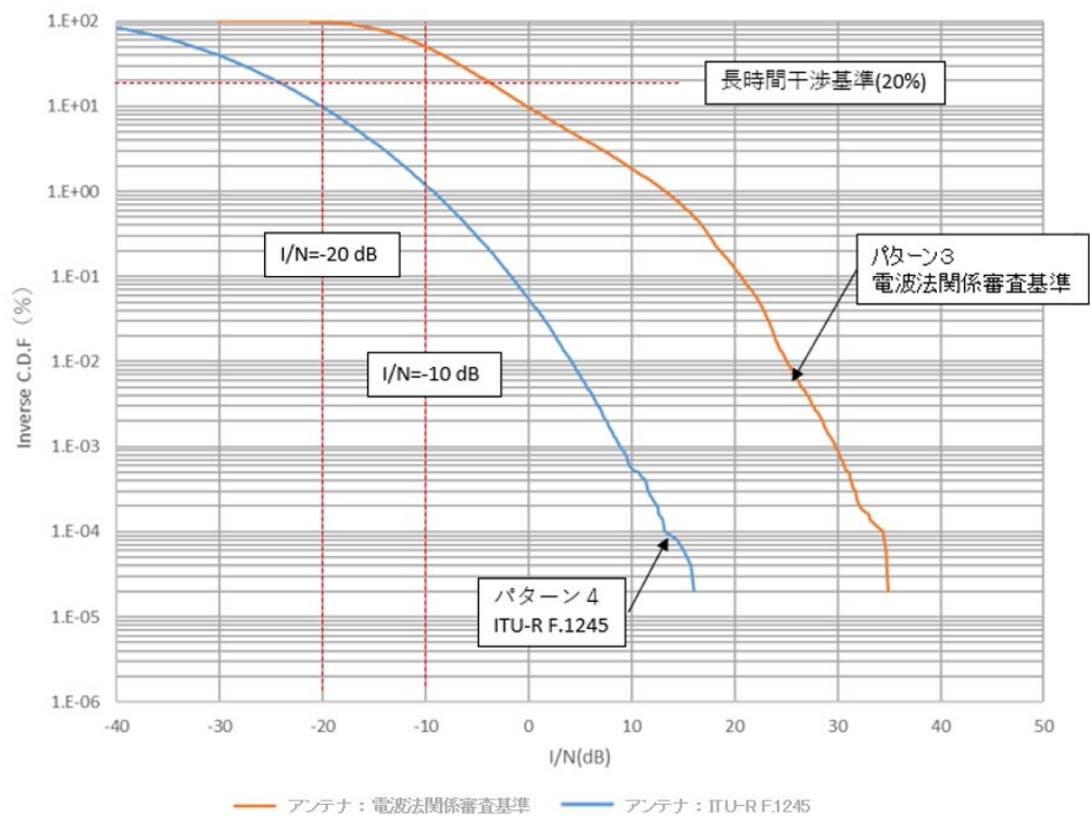
参考図 6.3-66 映像 STL パターン 3、4
