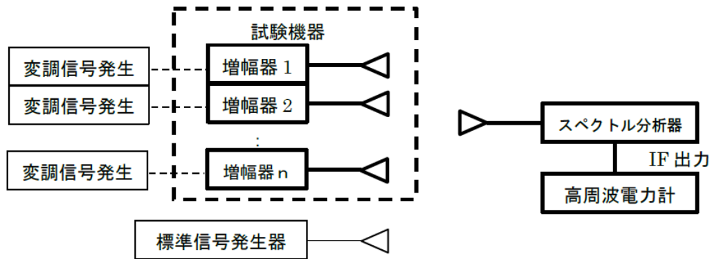
図 7.2-3 空中線電力測定系統図（空中線端子なしの場合）
