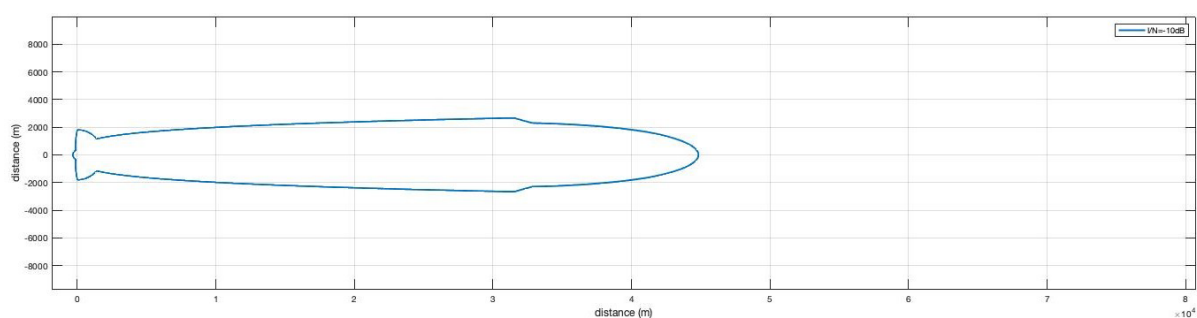
図 6.3-30 Pattern3-1 (電波法関係審査基準, VLP, 25mW, Outdoor, Body Loss あり)
