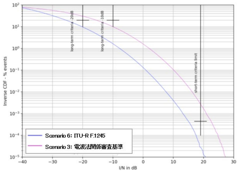
参考図 6.3-16 被干渉アンテナ地上高 25m の場合の結果（シナリオ 3, 6）
