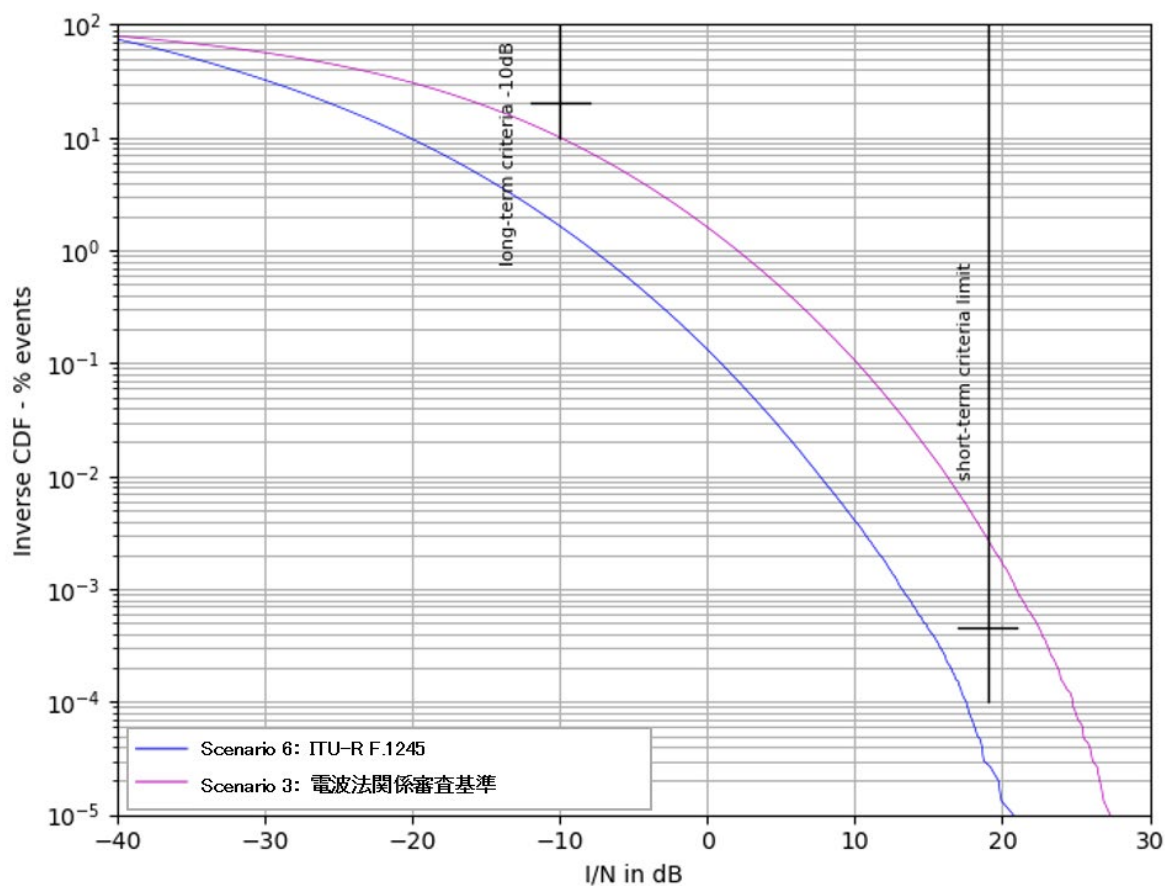
図 6.3-16 被干渉アンテナ地上高 25m の場合の結果 (シナリオ 3, 6)
