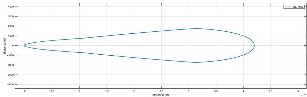
図 6.3-7 Pattern1-1 (電波法関係審査基準, LPI, 200mW, Indoor)
