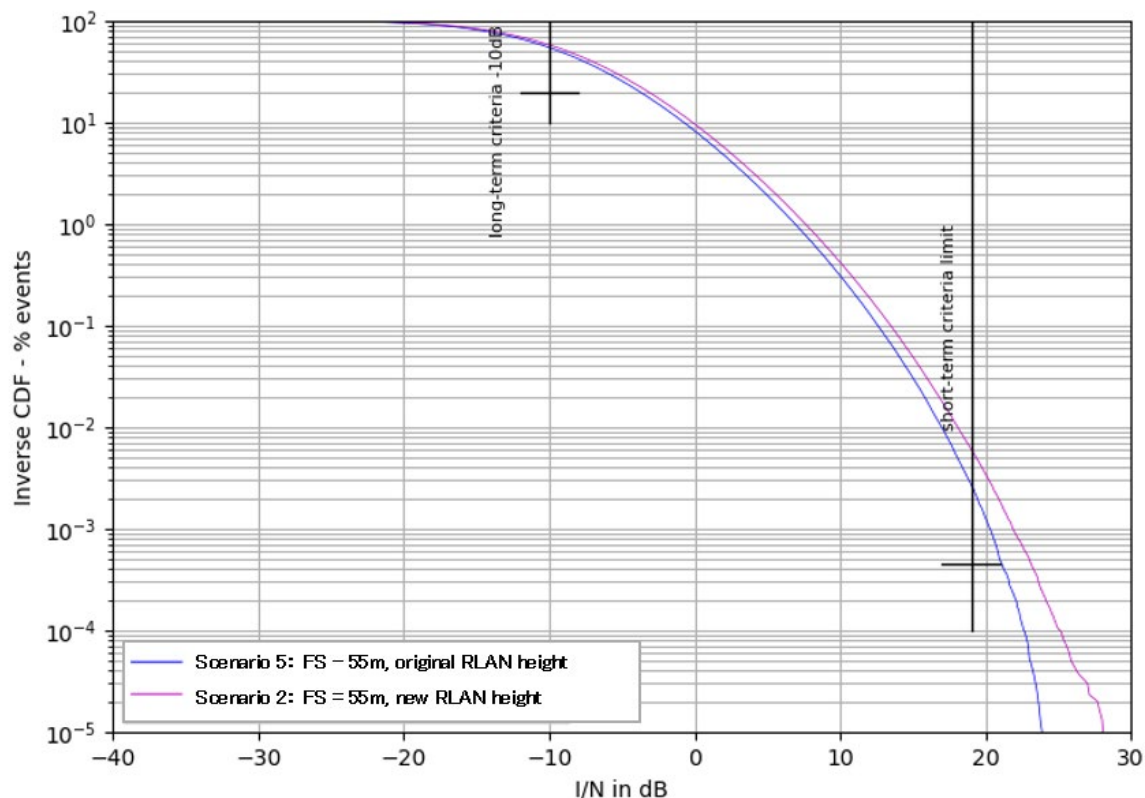
図 6.3-17 与干渉アンテナ地上高分布の変化に伴う結果の比較
