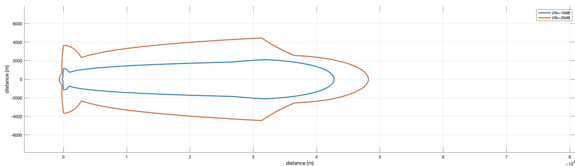
参考図 6.3-28 Pattern1-1（電波法関係審査基準, LPI, 200mW, Indoor）
