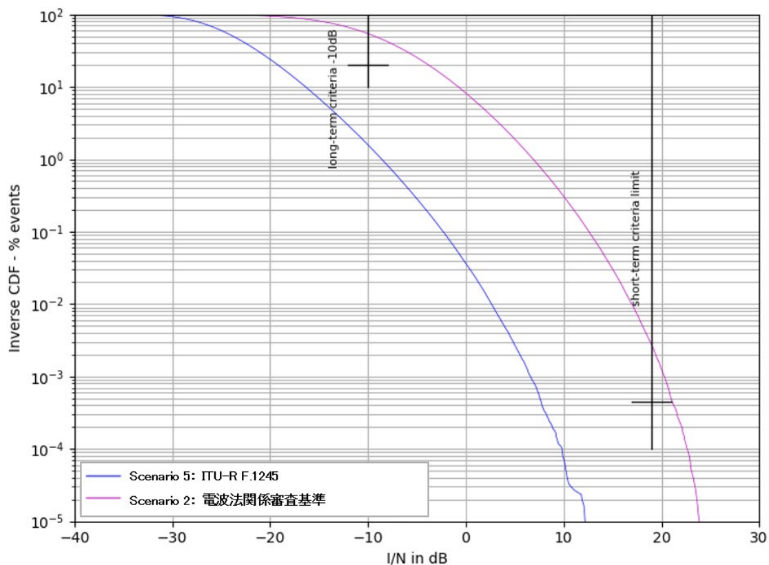
図 6.3-15 被干渉アンテナ地上高 55m の場合の結果 (シナリオ 2, 5)
