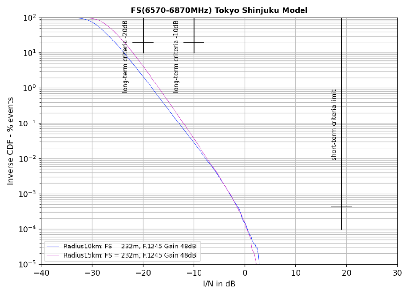
参考図 6.3-38 人口密集地での結果
