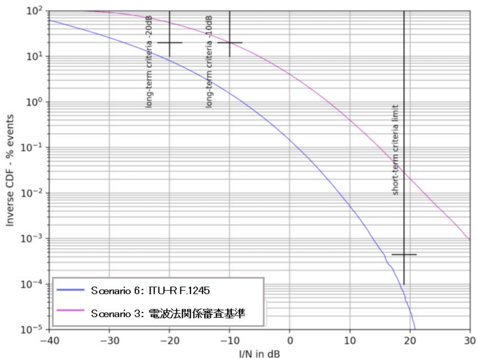
参考図 6.3-27 被干渉アンテナ地上高 25m の場合の結果（シナリオ 3, 6）
