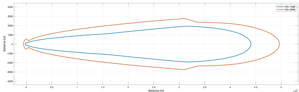
参考図 6.3-9 Pattern3-1 (電波法関係審査基準, VLP, 25mW, Outdoor, Body Loss あり)
