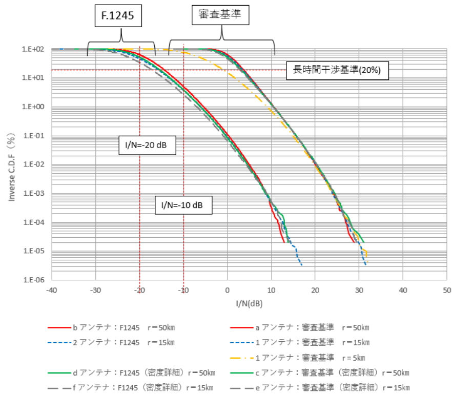
参考図 6.3-72 電波法関係審査基準及び Rec. ITU-R F.1245 の計算半径比較
