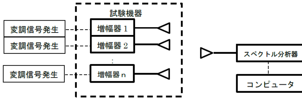
図 7.2-2 占有周波数帯幅測定系統図（空中線端子なしの場合）
