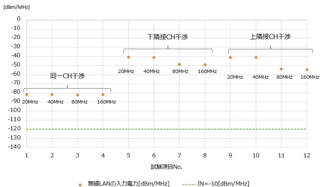
図 6.3-78 -54.5dBm(標準受信入力)試験の結果
