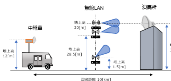
図 6.3-51 映像 FPU(固定)：中継車→演奏所の条件と所要離隔距離
