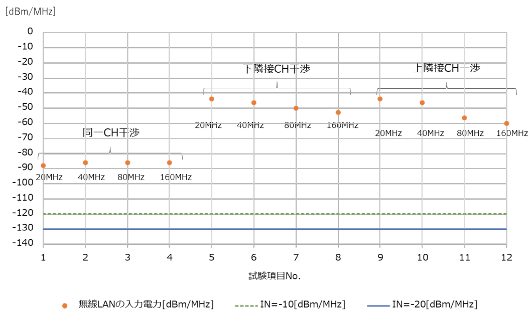
参考図 6.3-79 -65.5dBm(標準受信入力)試験の結果
