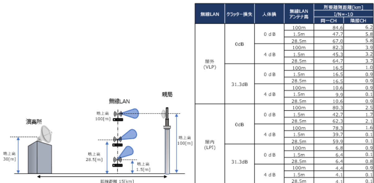
図 6.3-49 映像 STL：演奏所→親局の条件と所要離隔距離
