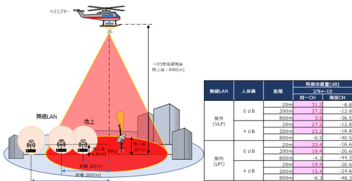
図 6.3-58 映像 FPU(移動) : 地上→ヘリコプター (urban) の条件と所要改善量
