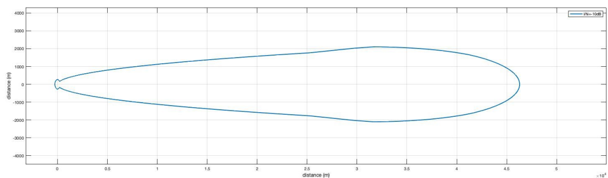
図 6.3-8 Pattern2-1 (電波法関係審査基準, VLP, 25mW, Outdoor, Body Loss なし)
