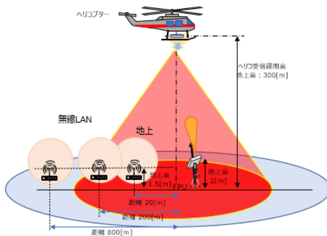
図 6.3-56 映像 FPU(移動)：地上→ヘリコプター(rural)の条件と所要改善量
