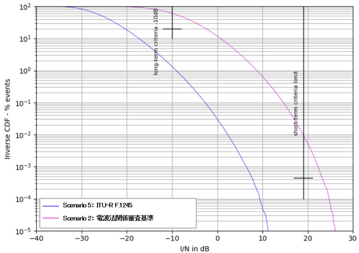
図 6.3-35 被干渉アンテナ地上高 55m の場合の結果（シナリオ 2, 5）
