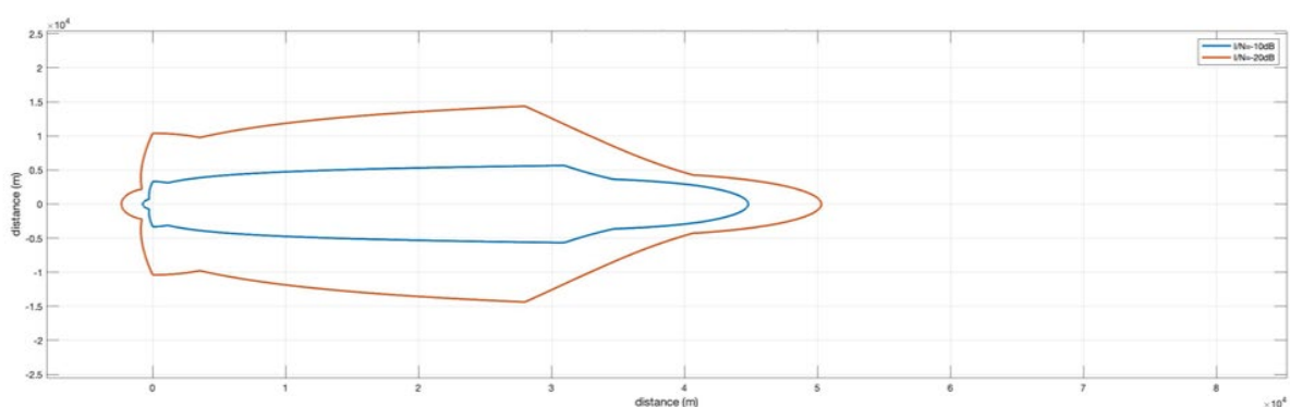
参考図 6.3-21 Pattern3-1 (電波法関係審査基準, VLP, 25mW, Outdoor, Body Loss あり)
