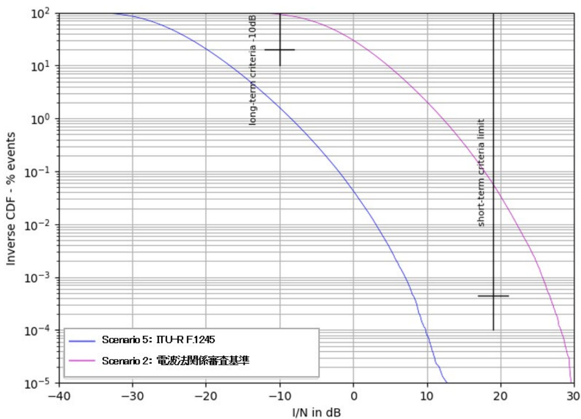
図 6.3-26 被干渉アンテナ地上高 55m の場合の結果（シナリオ 2, 5）
