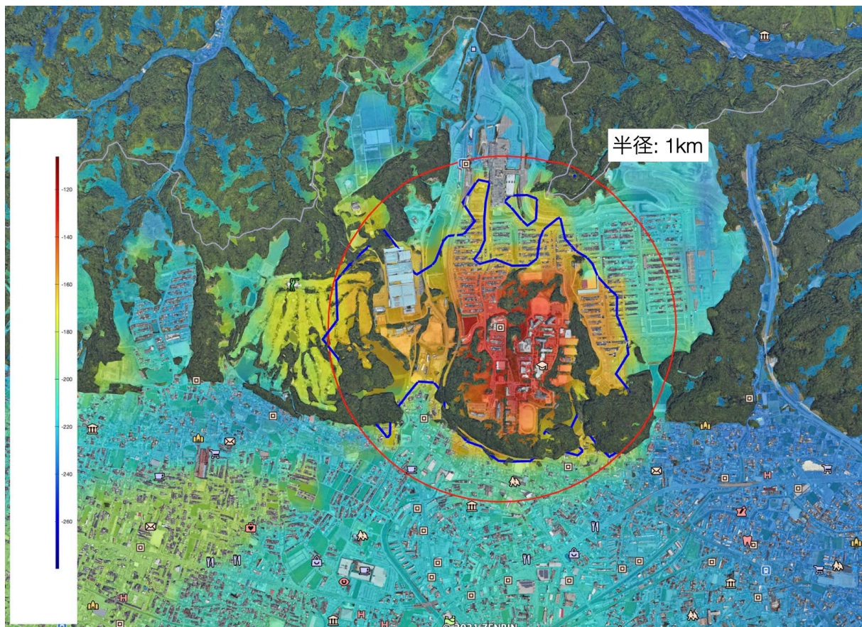
図 6.3-89 和歌山局周辺の地形データを考慮したシングルエントリーの結果
