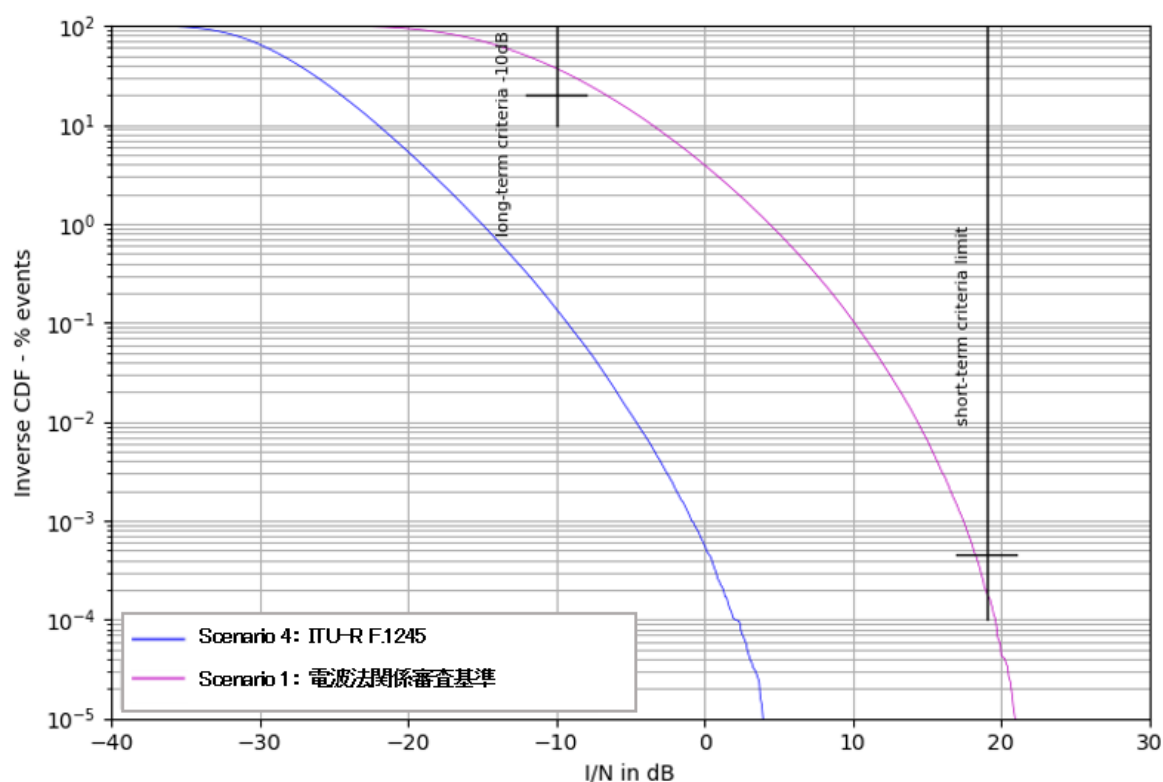
図 6.3-34 被干渉アンテナ地上高 110m の場合の結果 (シナリオ 1, 4)
