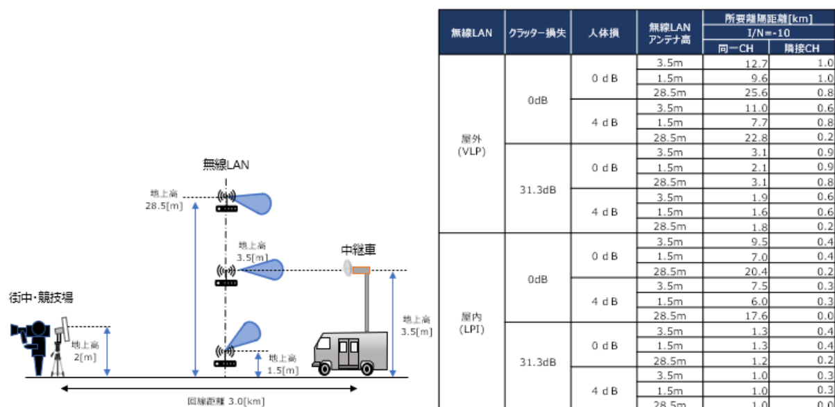
図 6.3-53 映像 FPU(移動) : 街中・競技場→中継車の条件と所要離隔距離
