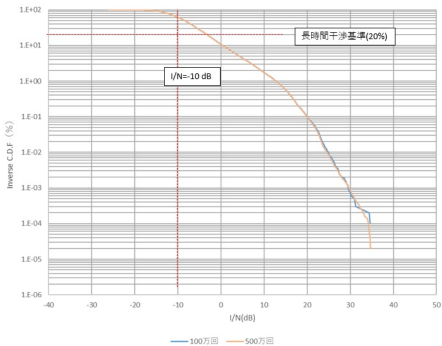
図 6.3-68 映像 TSL パターン 6
