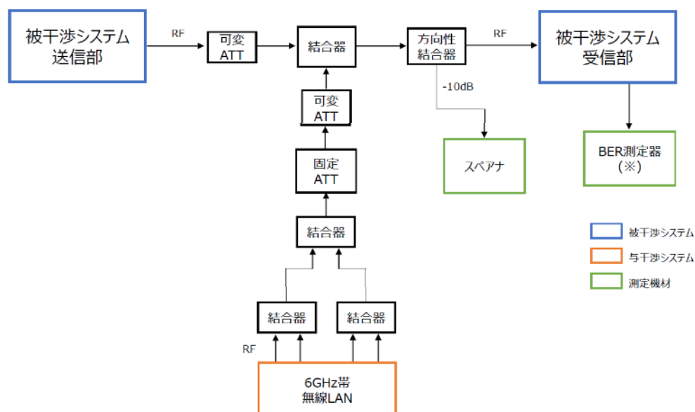
図 6.3-75 試験システム系統
