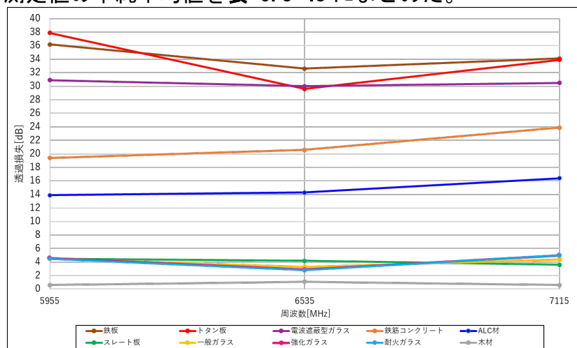
図 6.3-82 各建物建材の透過損失
