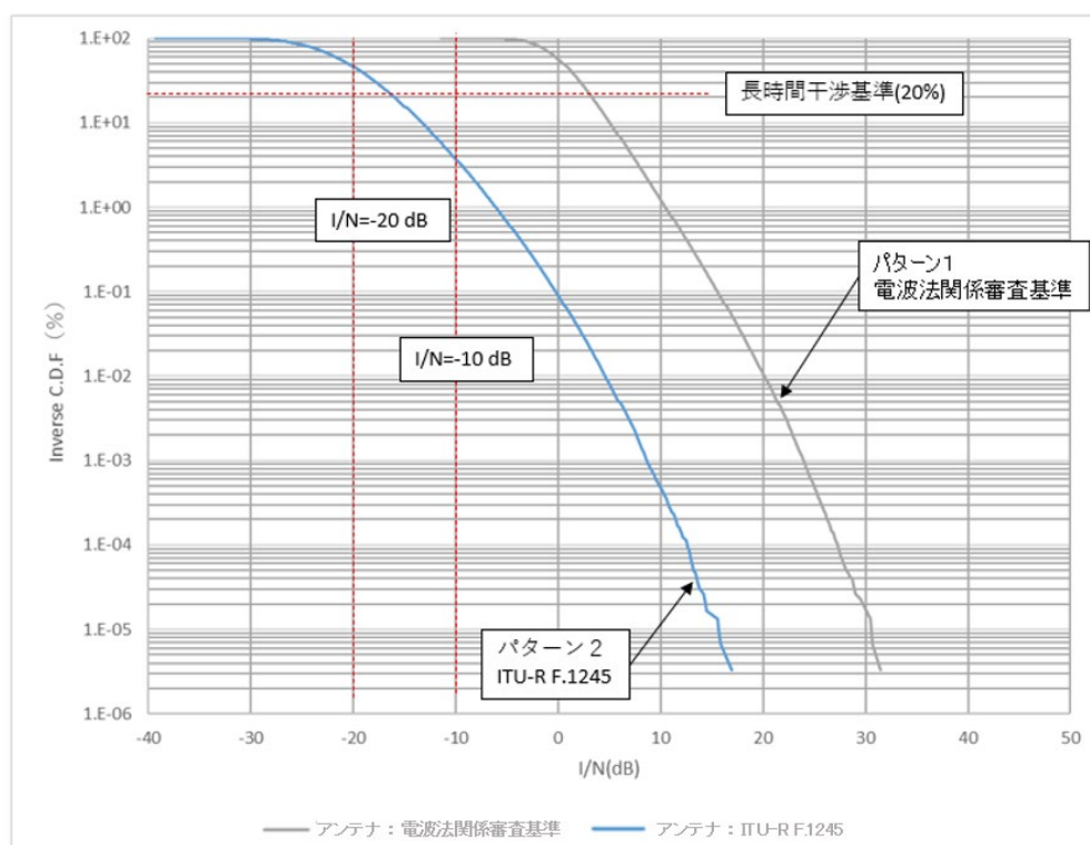
参考図 6.3-65 映像 STL パターン1、2
