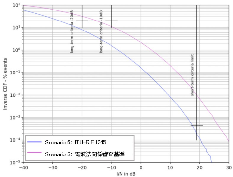
参考図 6.3-36 被干渉アンテナ地上高 20m の場合の結果（シナリオ 3, 6）
