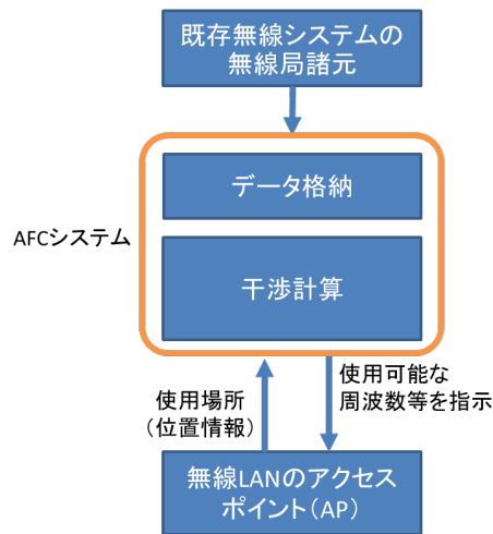
図 6.3-93 AFC システム構成図
