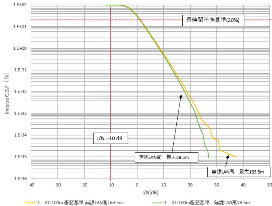
図 6.3-73 無線 LAN アンテナ地上高の比較
