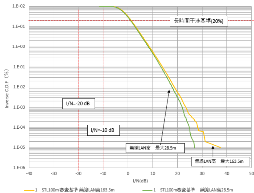
参考図 6.3-73 無線 LAN アンテナ地上高の比較
