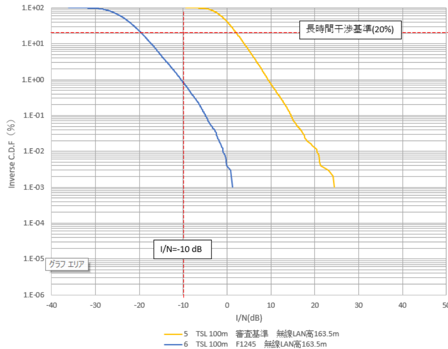
図 6.3-74 新しい無線 LAN アンテナ地上高分配によるシミュレーション結果
