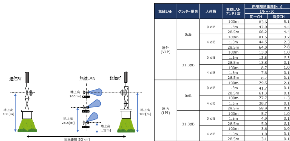
図 6.3-61 監視制御用固定回線 : 送信所→送信所の条件と所要離隔距離
