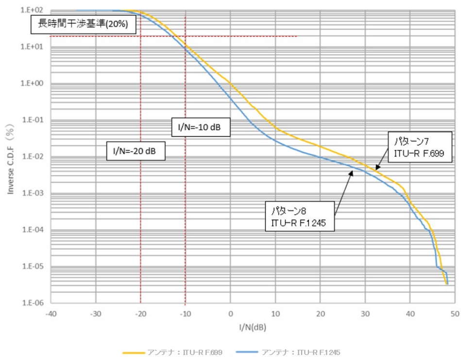
参考図 6.3-69 FPU パターン 7、8
