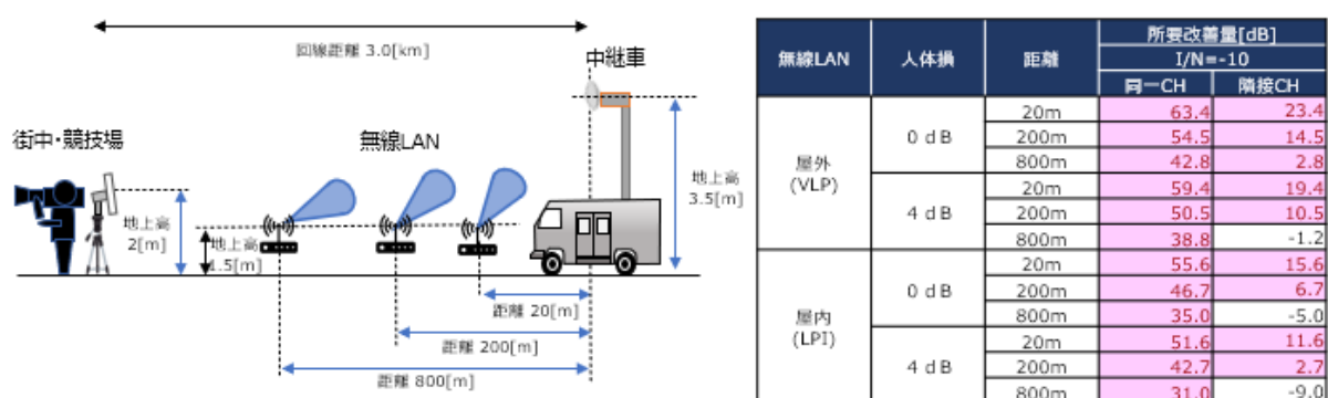
図 6.3-54 映像 FPU(移動) : 街中・競技場→中継車の条件と所要改善量
