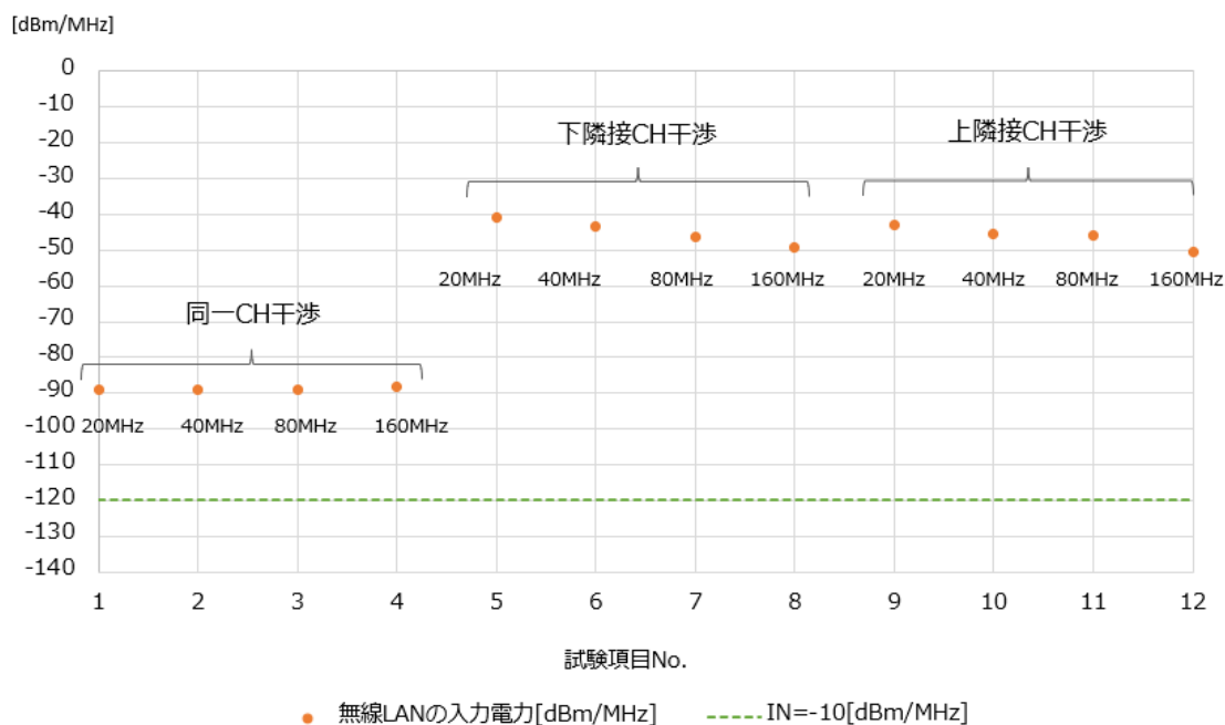
図 6.3-76 -55dBm (標準受信入力) 試験の結果
