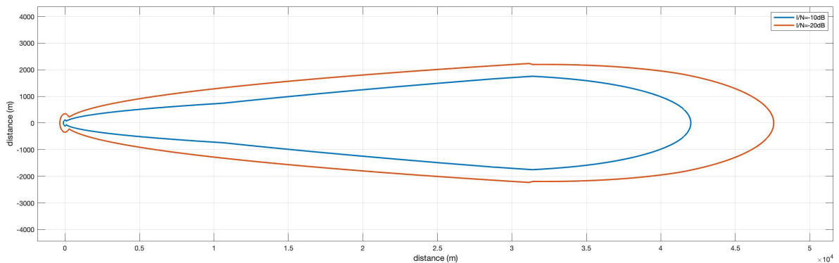
参考図 6.3-7 Pattern1-1 (電波法関係審査基準, LPI, 200mW, Indoor)
