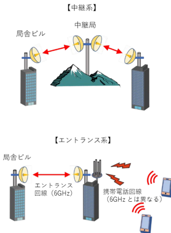
図 6.1-2 電気通信業務・公共業務・一般業務用固定局のサービス形態例
