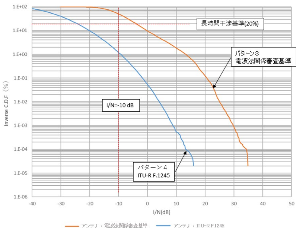
図 6.3-66 映像 STL パターン3、4
