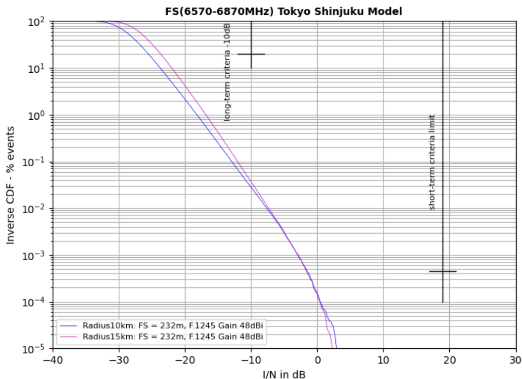
図 6.3-38 人口密集地での結果
