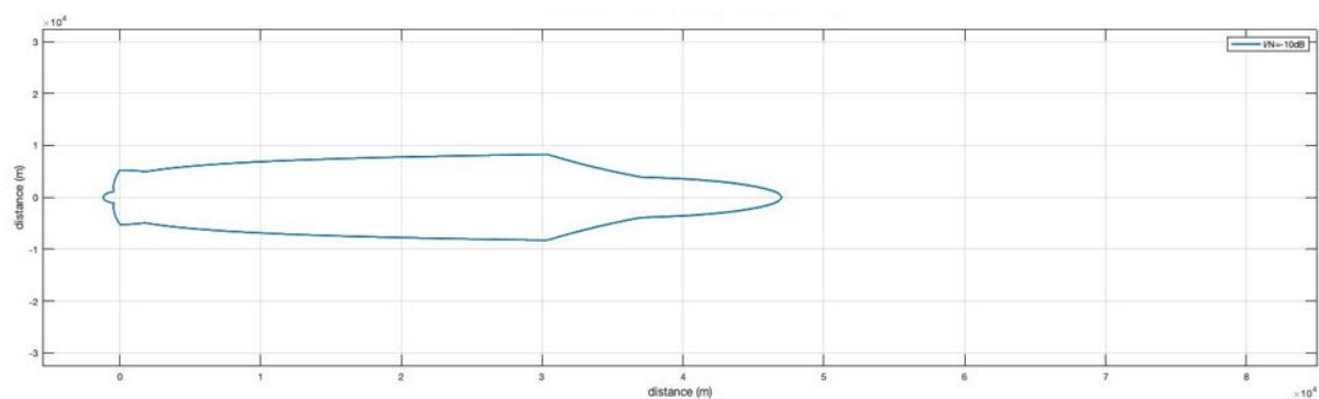
図 6.3-20 Pattern2-1 (電波法関係審査基準, VLP, 25mW, Outdoor, Body Loss なし)
