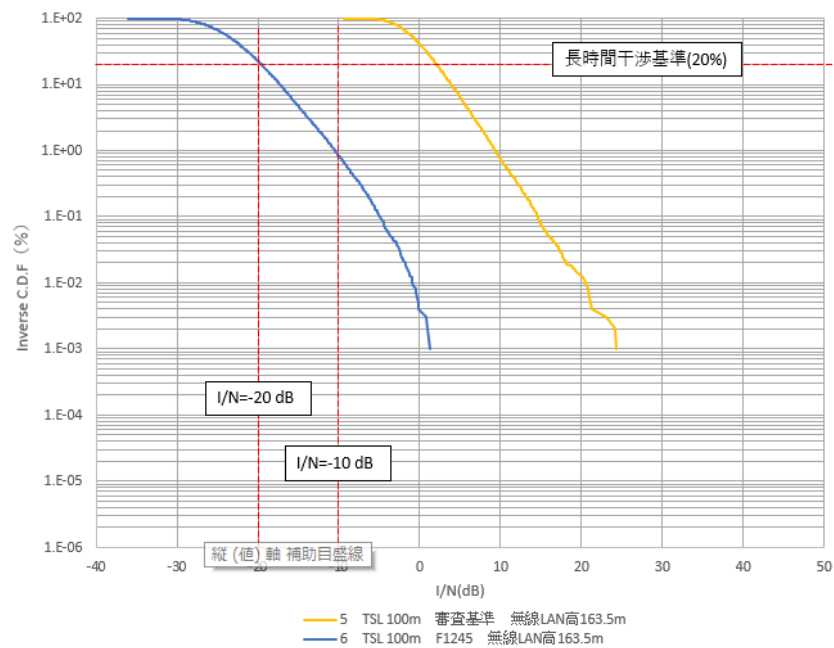
参考図 6.3-74 新しい無線 LAN アンテナ地上高分配によるシミュレーション結果
