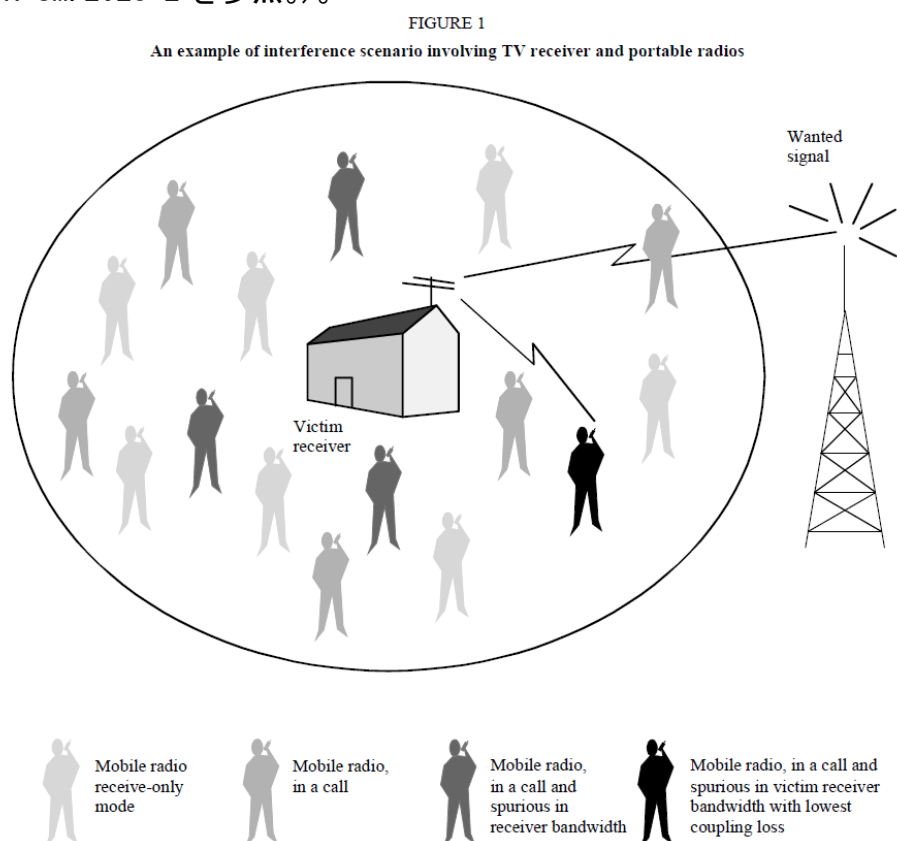
図 6.3-13 移動体通信機器から TV 受信機への干渉計算の例
