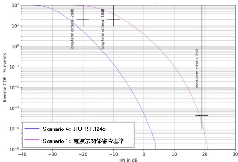
参考図 6.3-34 被干渉アンテナ地上高 110m の場合の結果 (シナリオ 1, 4)
