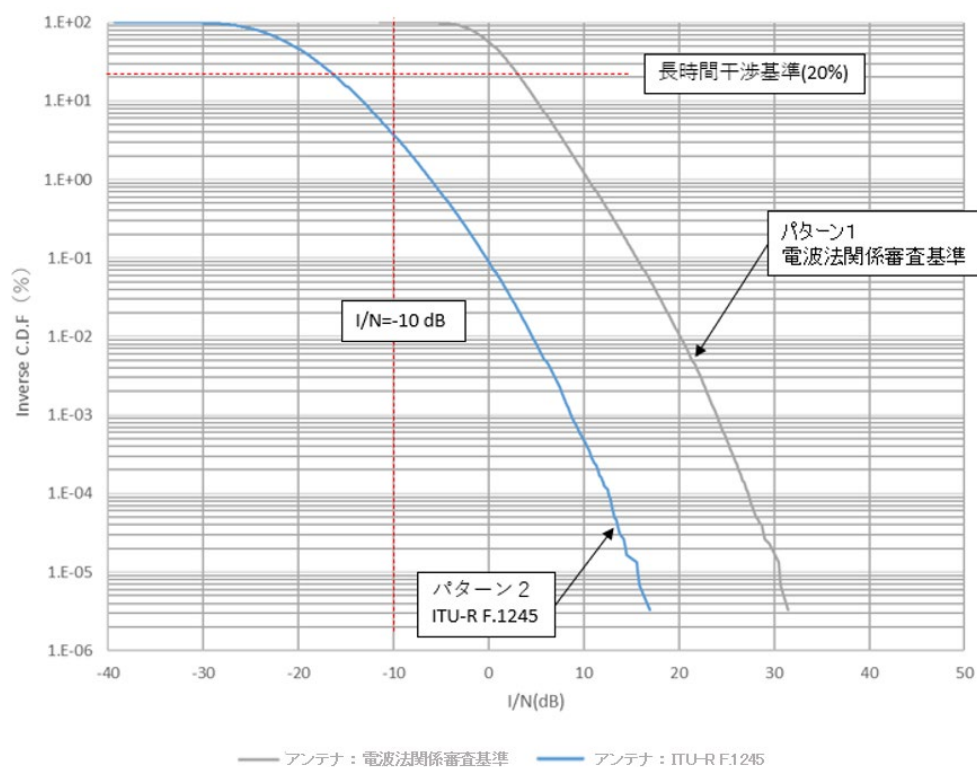
図 6.3-65 映像 STL パターン1、2
