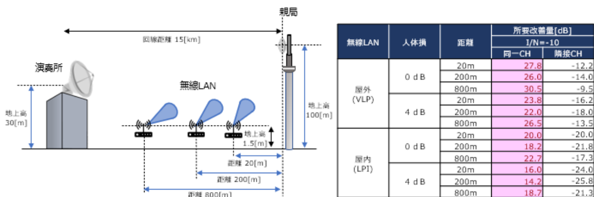
図 6.3-60 音声 STL : 演奏所→親局の条件と所要改善量
