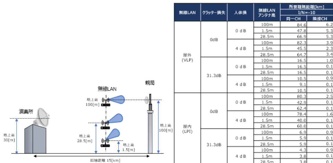
図 6.3-59 音声 STL : 演奏所→親局の条件と所要離隔距離
