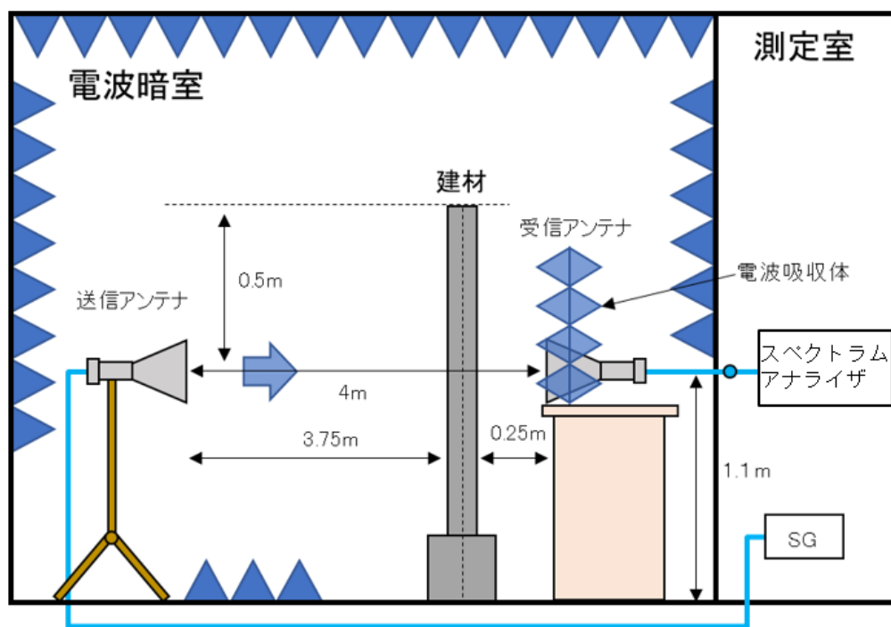
図 6.3-80 透過損失試験の試験系統
