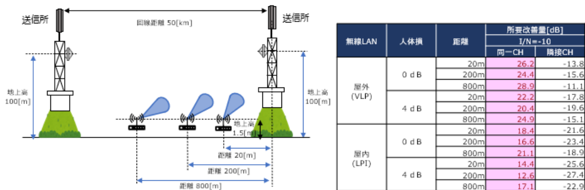
図 6.3-62 監視制御用固定回線：送信所→送信所の条件と所要改善量
