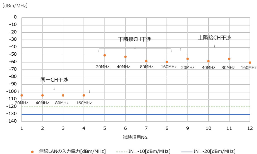
参考図 6.3-77 -70dBm 試験の結果
