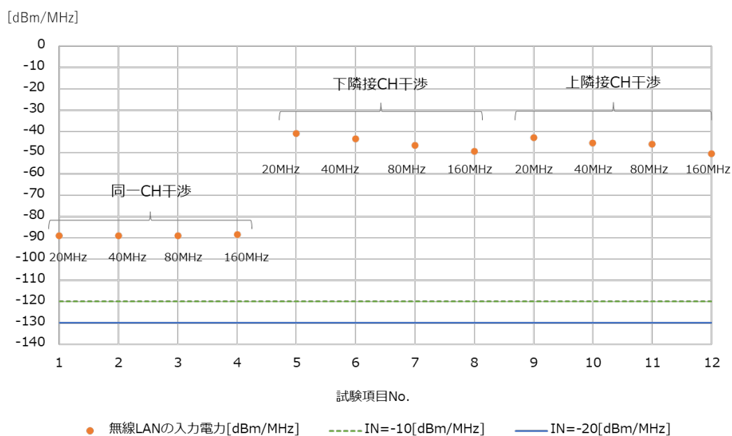
参考図 6.3-76 -55dBm(標準受信入力)試験の結果
