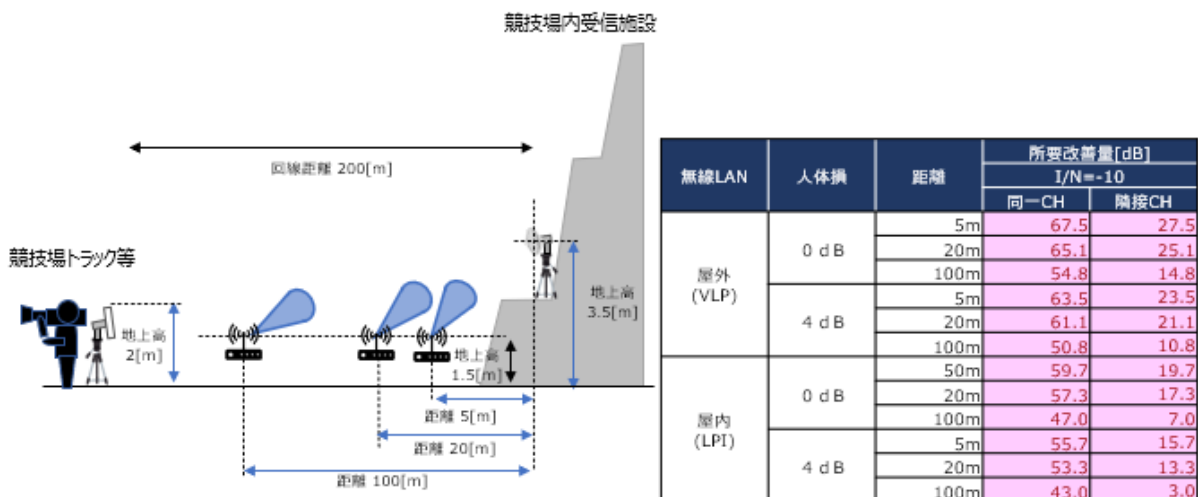
図 6.3-64 映像 FPU(移動)：競技場トラック等→競技場内受信施設の条件と所要改善量
