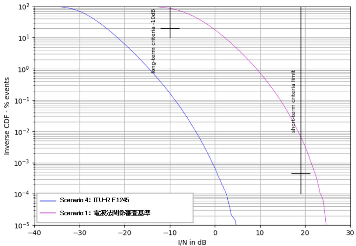
図 6.3-25 被干渉アンテナ地上高 110m の場合の結果 (シナリオ 1, 4)
