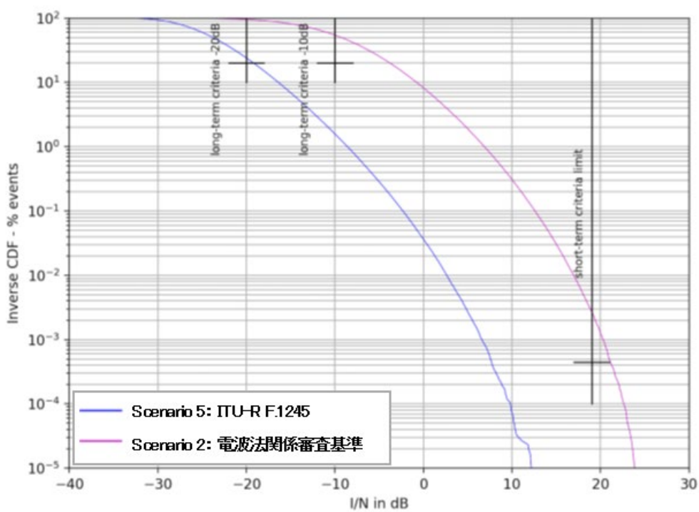
参考図 6.3-15 被干渉アンテナ地上高 55m の場合の結果（シナリオ 2, 5）
