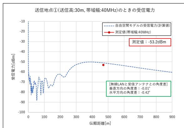
図 6.3-85 測定結果と理論値との比較 送信地点①(カテゴリ A)
