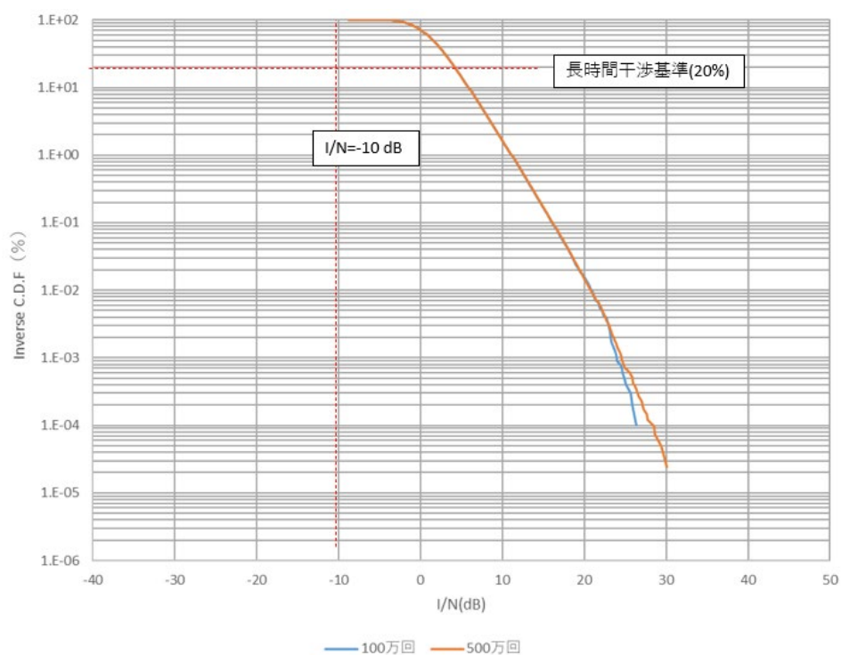
図 6.3-67 映像 TSL パターン 5
