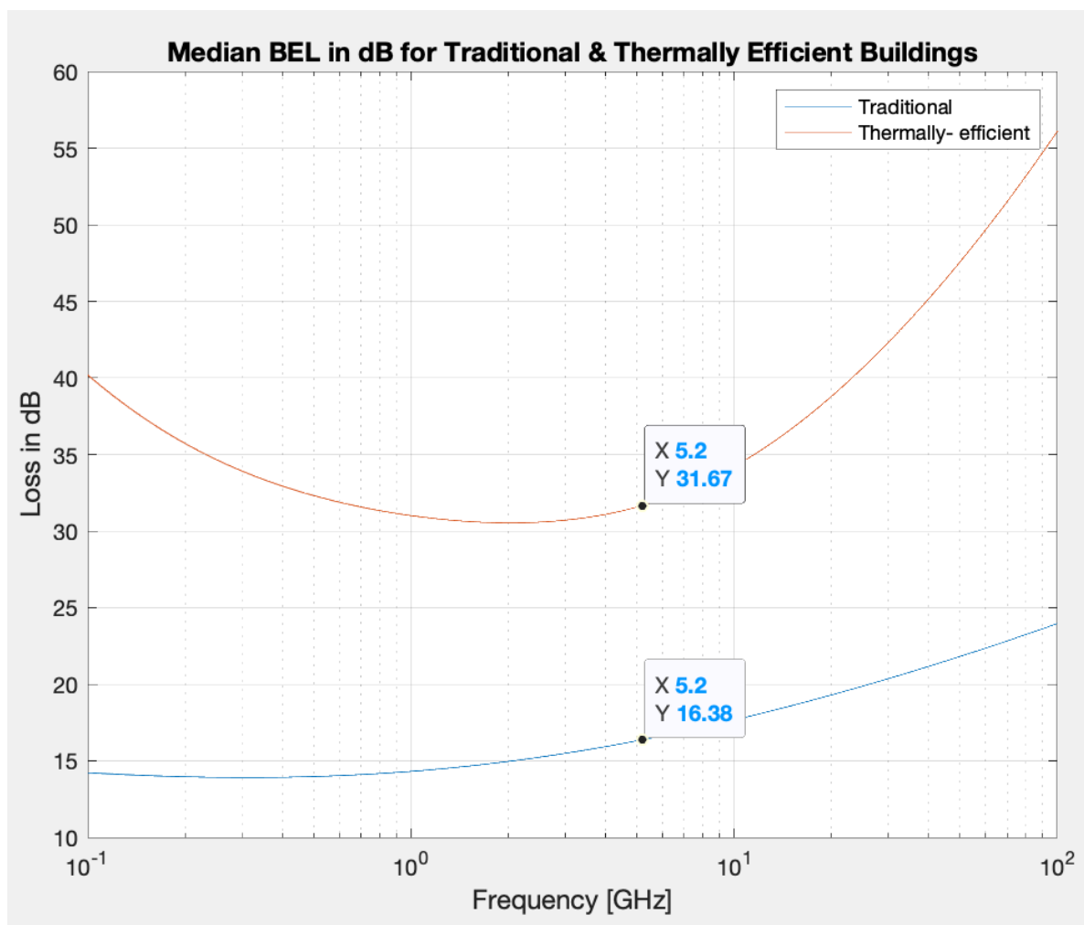
図 5-3-1 ITU-R 勧告 P. 2109 による建物遮蔽損失
