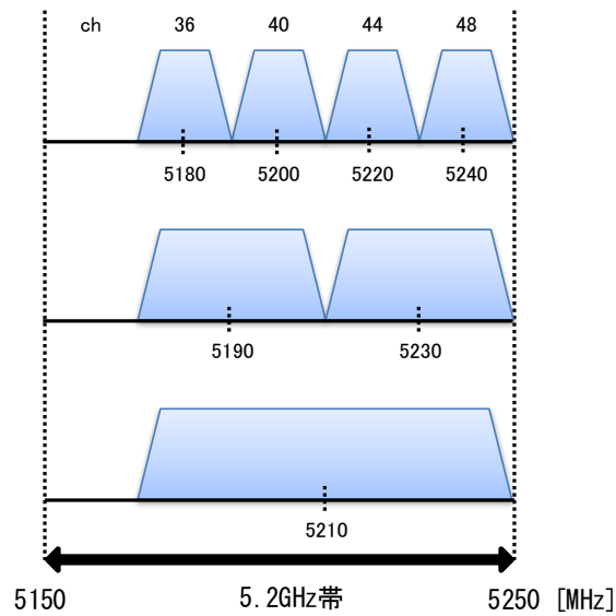
図 6-1-1 5.2GHz 帯自動車内無線 LAN システムの周波数チャネル配置図
