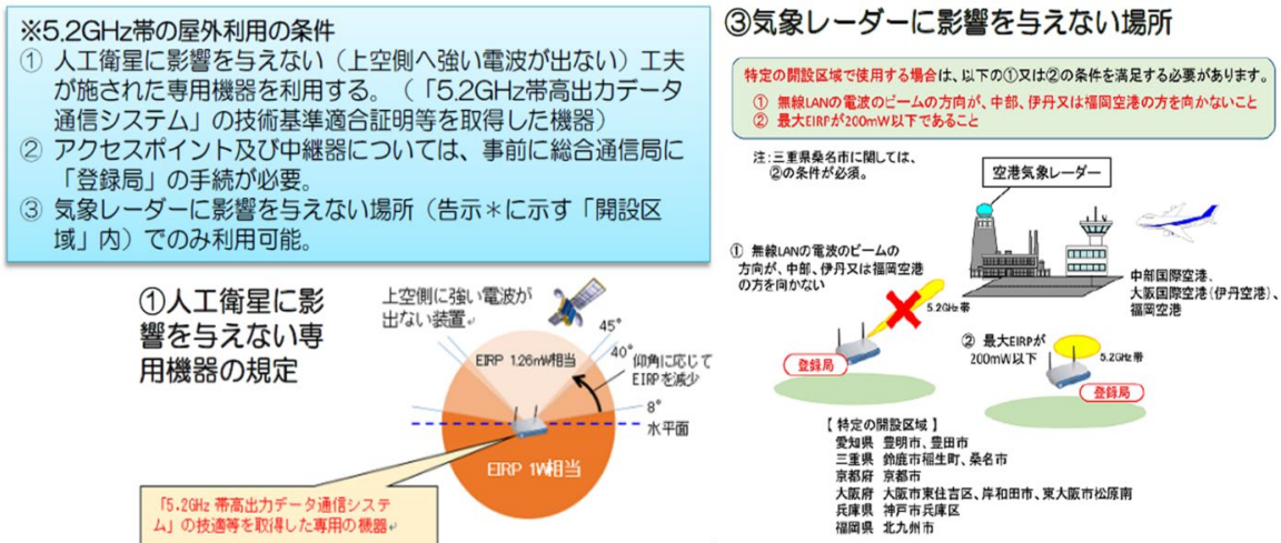
図 2-1-2 5.2GHz 帯高出力データ通信システムの屋外利用のための共用条件
