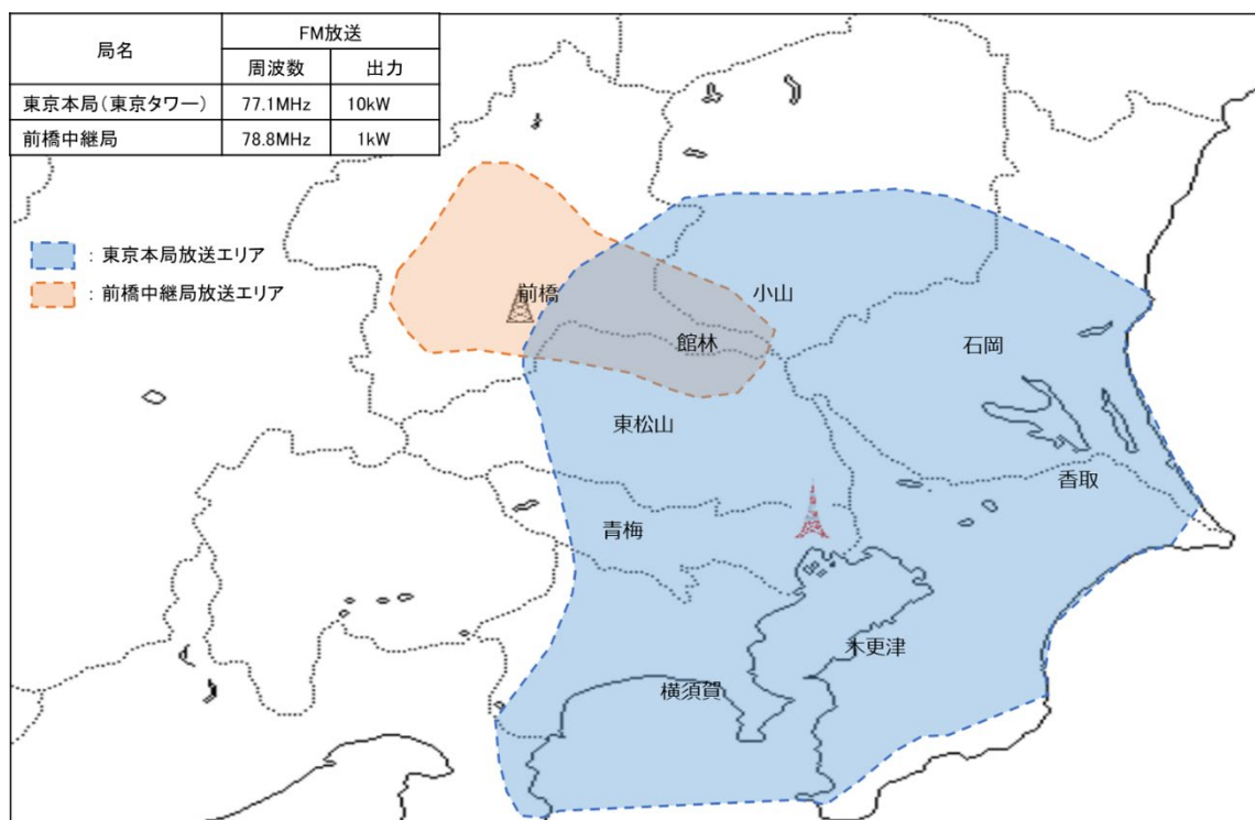
図5 放送大学の FM 放送跡地のエリア図
