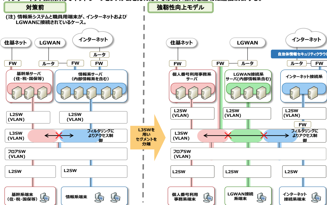
図表 16 強靱性向上モデルにおけるネットワーク再構成の一つのイメージ
