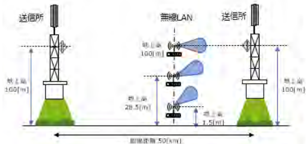
図 6.3-61 監視制御用固定回線 : 送信所→送信所の条件と所要離隔距離
