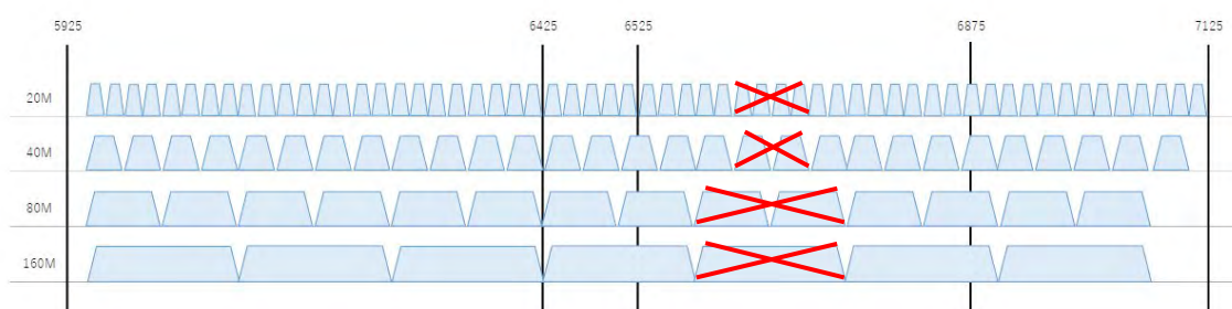
図 6.3-92 電波天文の保護のための使用禁止チャンネル
