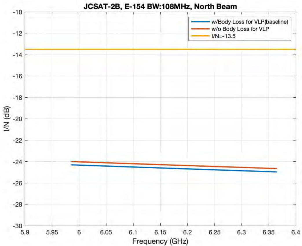
图 6.3-43 JCSAT-2B
