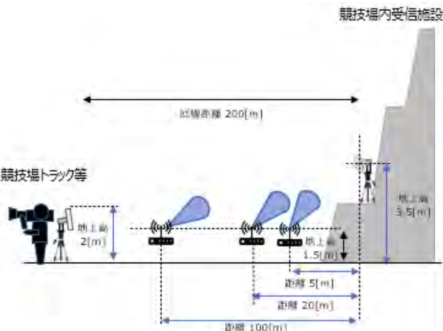
図 6.3-64 映像 FPU(移動)：競技場トラック等→競技場内受信施設の条件と所要改善量
