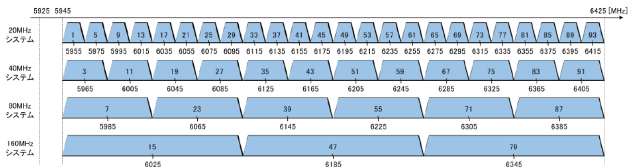
図 7.1-1 6GHz帯無線LANシステムの周波数チャンネル配置
