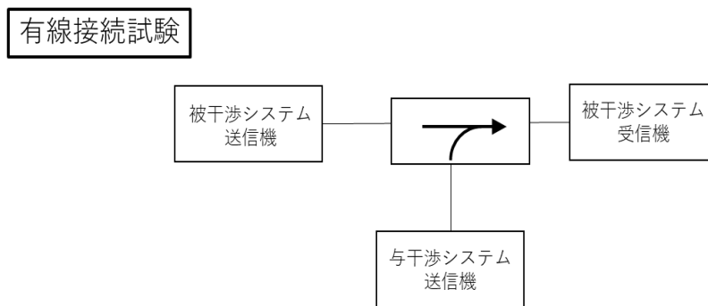
図 6.3-4 屋内実証実験
