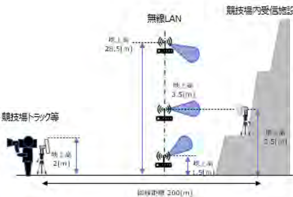
図 6.3-63 映像 FPU(移動)：競技場トラック等→競技場内受信施設の条件と所要離隔距離
