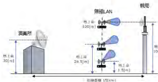
図 6.3-59 音声 STL : 演奏所→親局の条件と所要離隔距離
