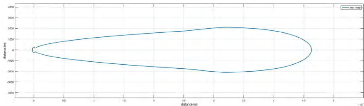
図 6.3-8 Pattern2-1 (電波法関係審査基準, VLP, 25mW, Outdoor, Body Loss なし)
