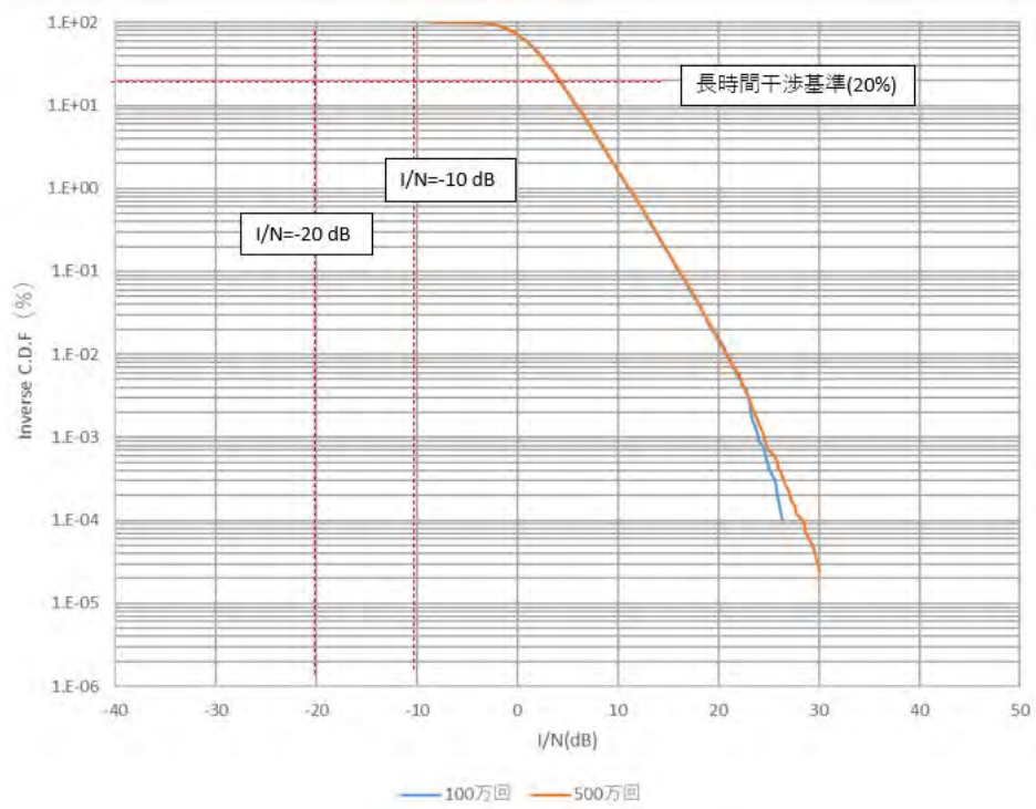
参考図 6.3-67 映像 TSL パターン 5
