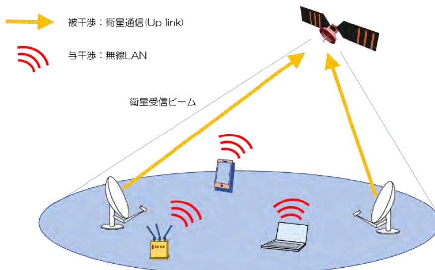
図 6.3-40 無線 LAN から静止衛星システム(Uplink)への与干渉
