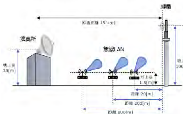
図 6.3-60 音声 STL : 演奏所→親局の条件と所要改善量
