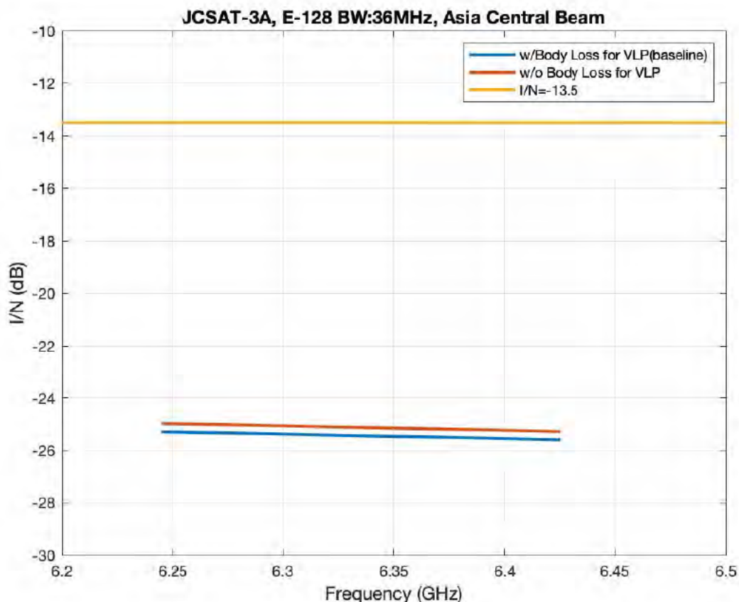
図 6.3-44 JCSAT-3A
