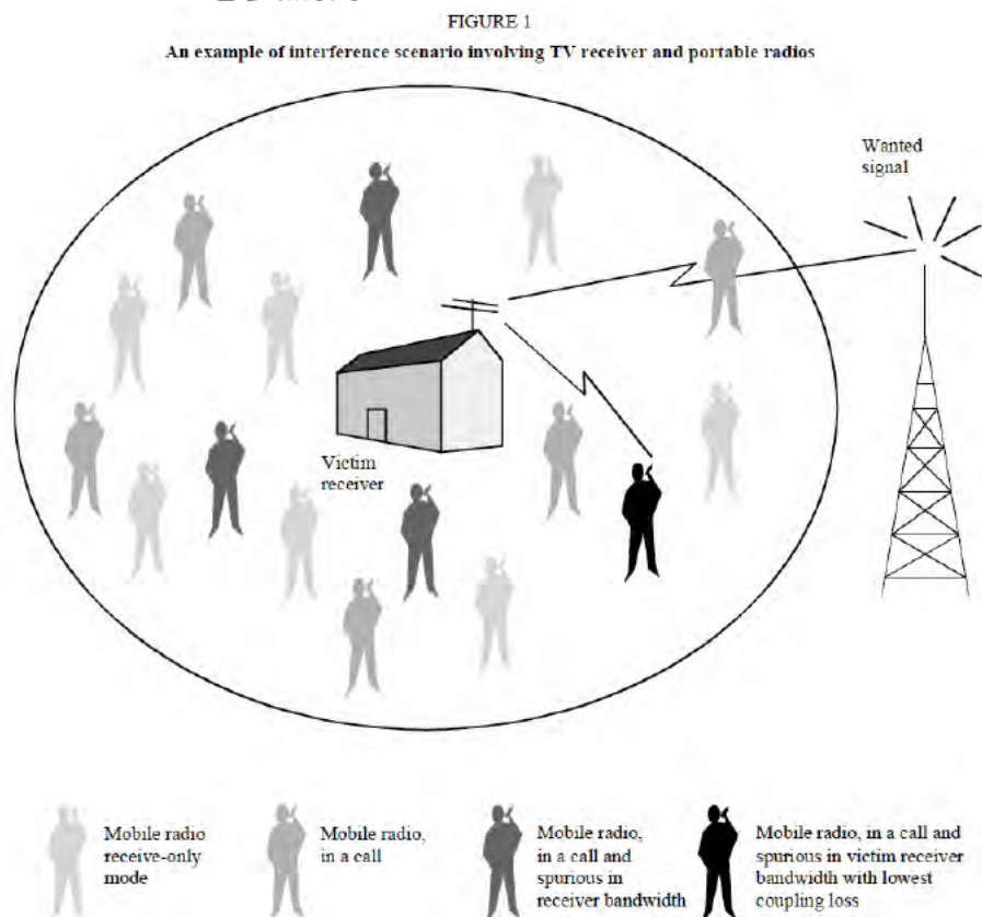
図 6.3-13 移動体通信機器から TV 受信機への干渉計算の例 (図は Rep. ITU-R SM. 2028-2 から引用)
