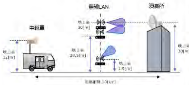
図 6.3-51 映像 FPU(固定) : 中継車→演奏所の条件と所要離隔距離
