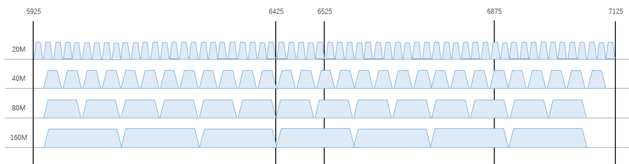
図 5.1-1 6GHz 帯無線 LAN システムのチャンネル配置
