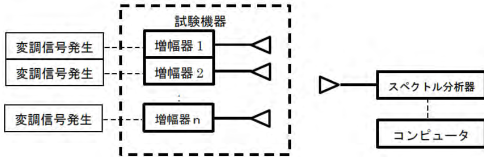
図 7.2-2 占有周波数帯幅測定系統図（空中線端子なしの場合）
