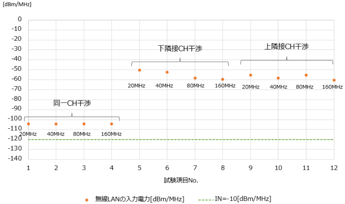
図 6.3-77 -70dBm 試験の結果
