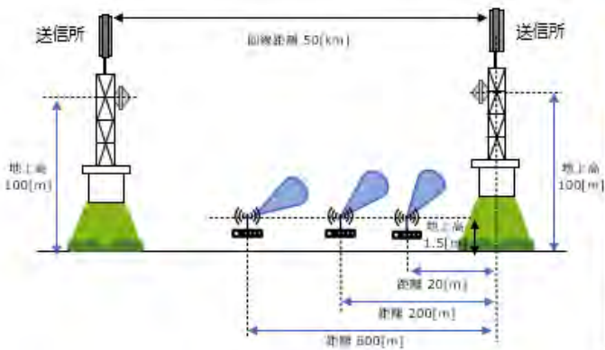
図 6.3-62 監視制御用固定回線：送信所→送信所の条件と所要改善量
