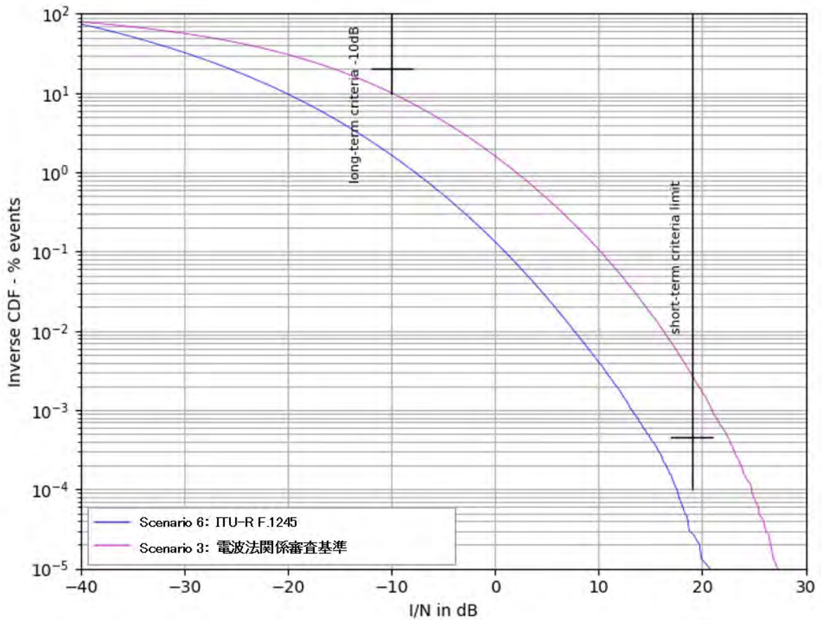
図 6.3-16 被干渉アンテナ地上高 25m の場合の結果 (シナリオ 3, 6)
