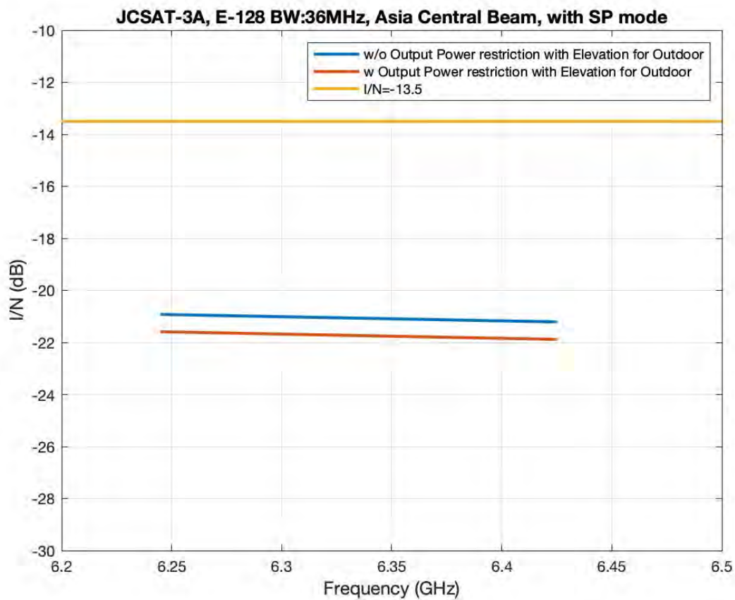
図 6.3-48 JCSAT-3A
