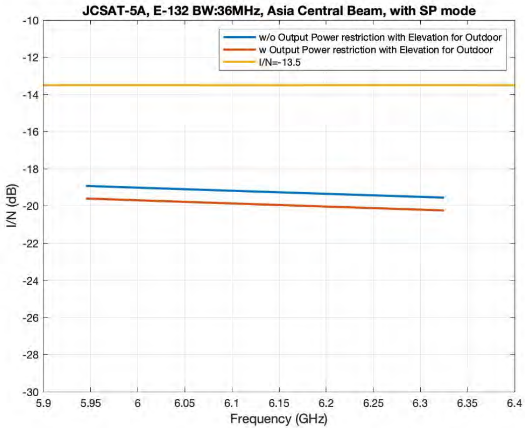
图 6.3-46 JCSAT-5A
