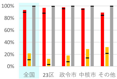
地域ごとの256QAM導入状況
