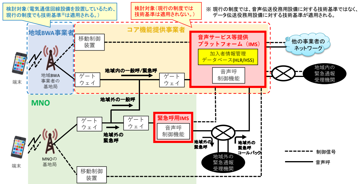
＜図 2-4＞コア機能提供事業者が音声伝送携帯電話番号の指定を受ける場合のネットワーク構成
