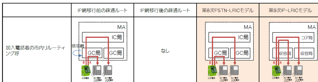
図3-12 加入電話着の市内リレーティング呼
