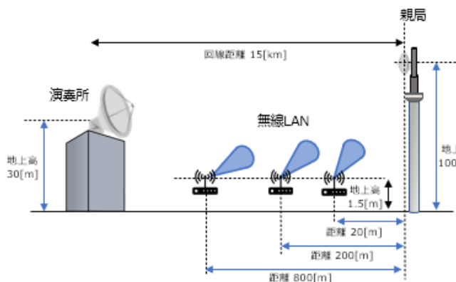
図 6.3-60 音声 STL : 演奏所→親局の条件と所要改善量
