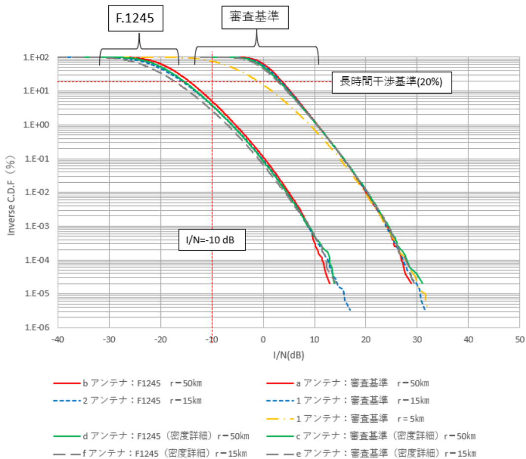
図 6.3-72 電波法関係審査基準および ITU-RF. 1245 の計算半径比較
