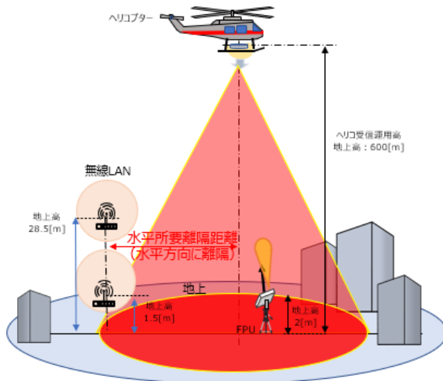
図 6.3-57 映像 FPU(移動) : 地上→ヘリコプター (urban) の条件と所要離隔距離
