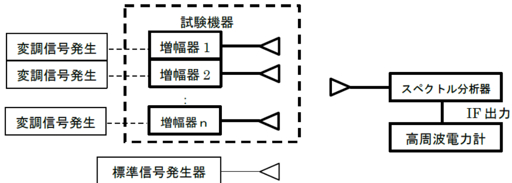
図 7.2-3 空中線電力測定系統図（空中線端子なしの場合）
