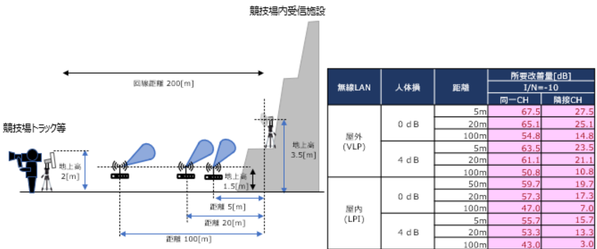
図 6.3-64 映像 FPU(移動) : 競技場トラック等→競技場内受信施設の条件と所要改善量
