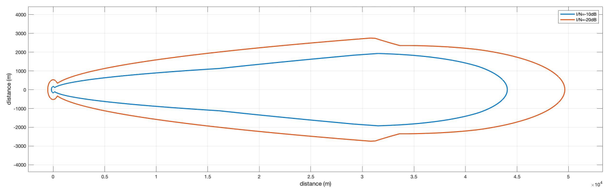
参考図 6.3-9 Pattern3-1 (電波法関係審査基準, VLP, 25mW, Outdoor, Body Loss あり)
