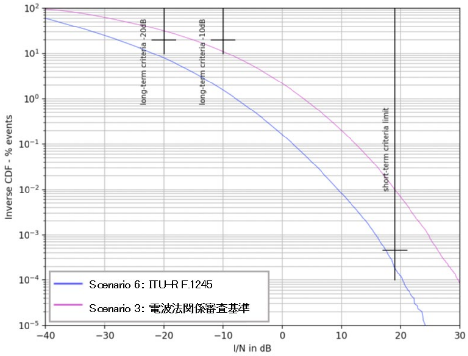
参考図 6.3-36 被干渉アンテナ地上高 20m の場合の結果 (シナリオ 3, 6)
