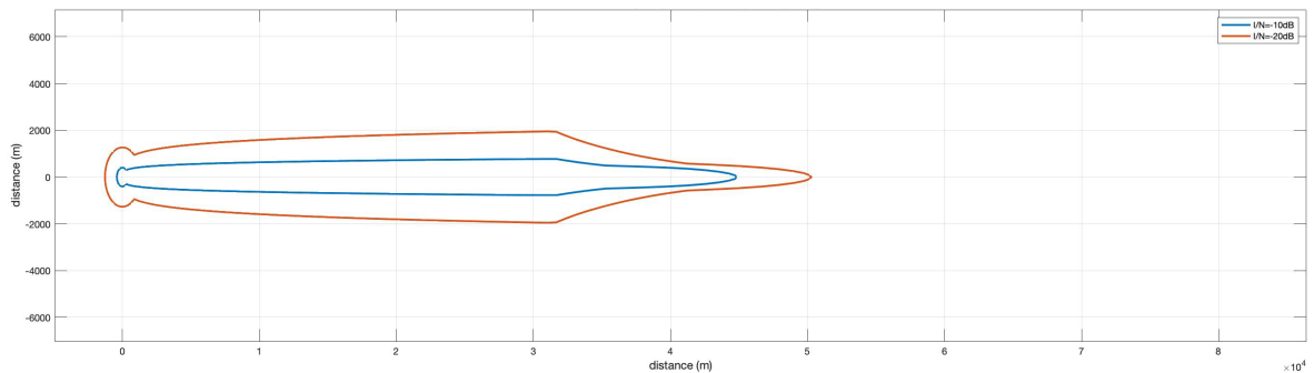
参考図 6.3-33 Pattern3-2 (ITU-R F.1245, VLP, 25mW, Outdoor, Body Loss あり)
