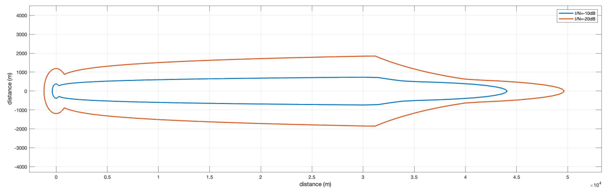
参考図 6.3-12 Pattern3-2 (ITU-R F.1245, VLP, 25mW, Outdoor, Body Loss あり)
