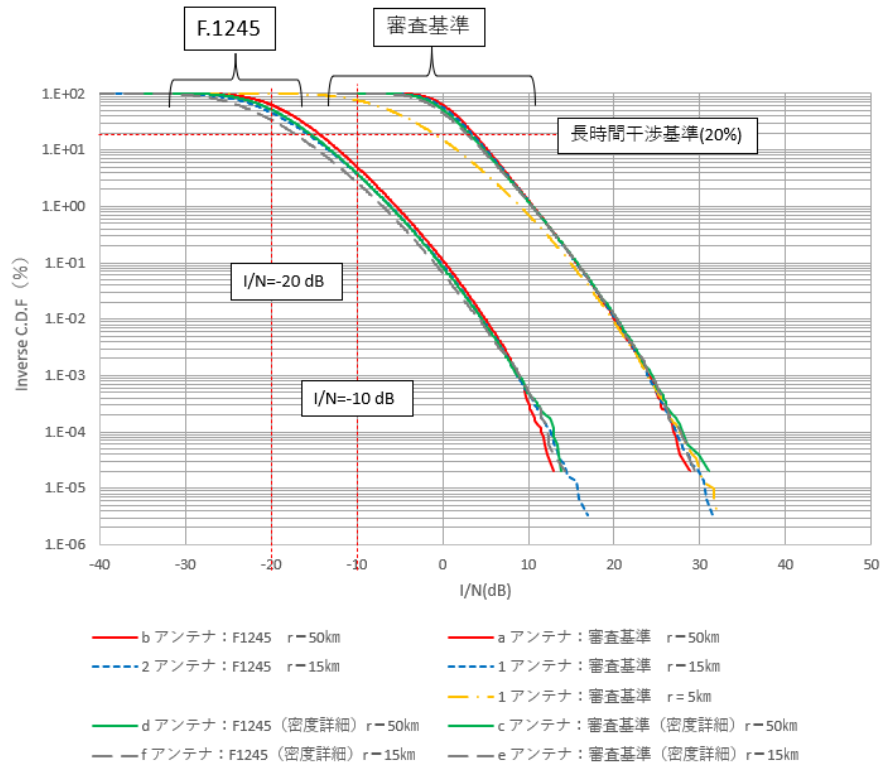
参考図 6.3-72 電波法関係審査基準および ITU-RF.1245 の計算半径比較
