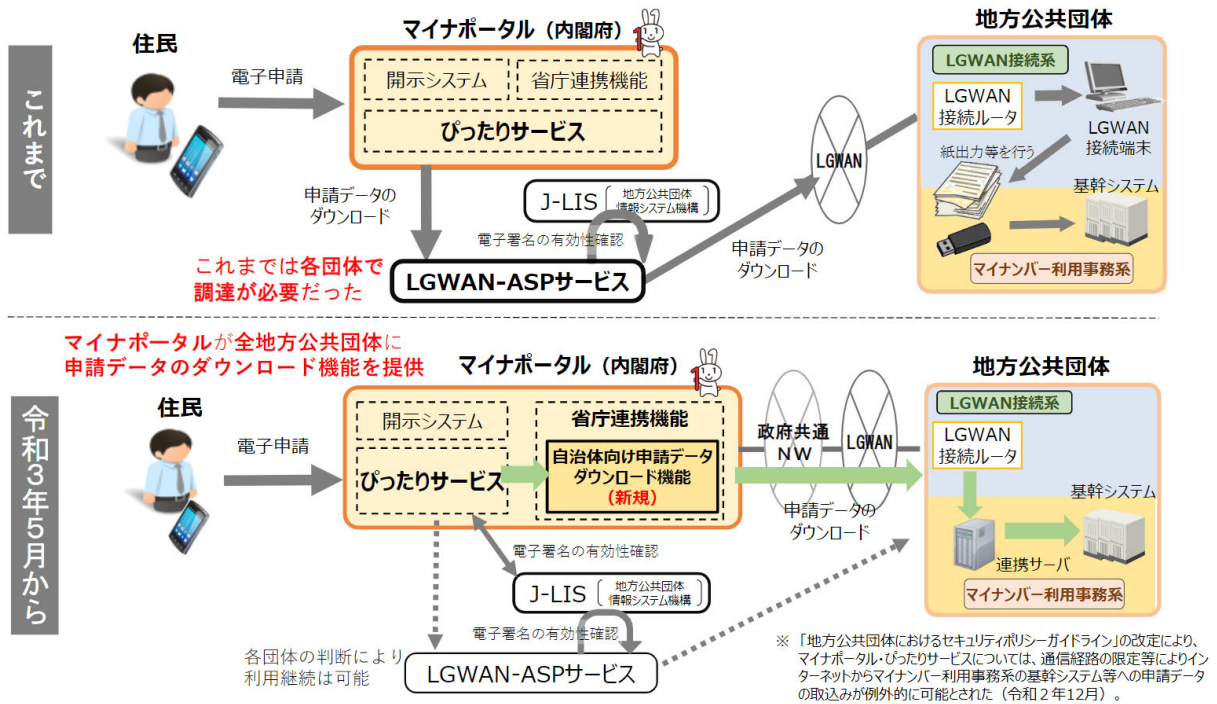
図表 3015 全自治体接続基盤の構築
