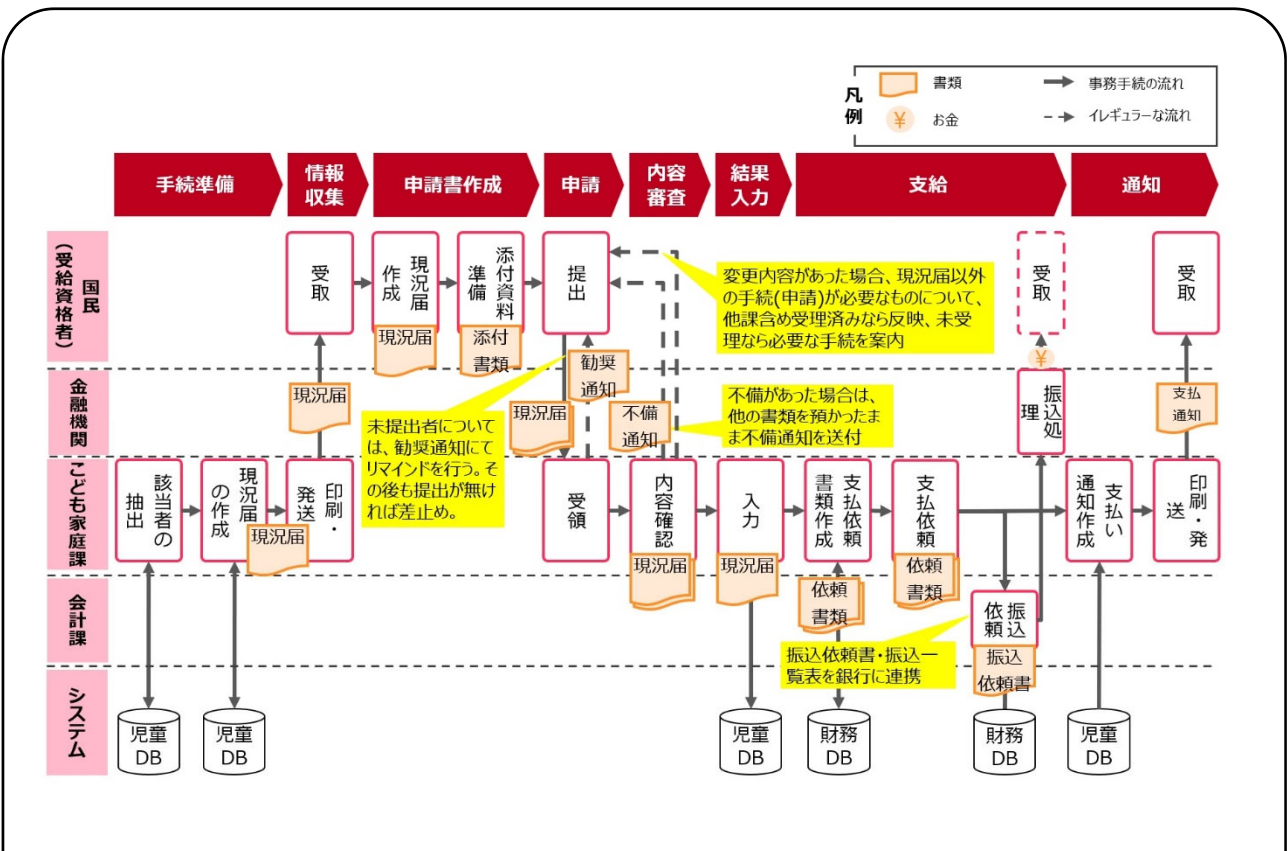
図表-8-12 児童手当の現況届の申請受付事務フロー例（オンライン化前）
