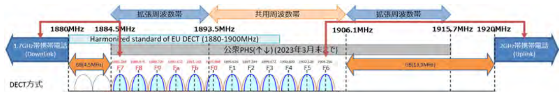
図 2. 2-7 DECT 方式と隣接する携帯電話との周波数位置関係
