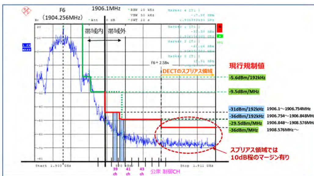
※引用：陸上無線通信委員会報告(平成29年3月31日) 図3. 1-5
