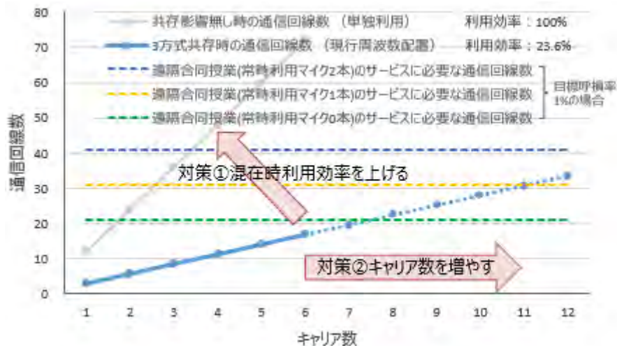
図1. 2-16 ワイヤレスマイク全教室導入に必要なキャリア数概算
