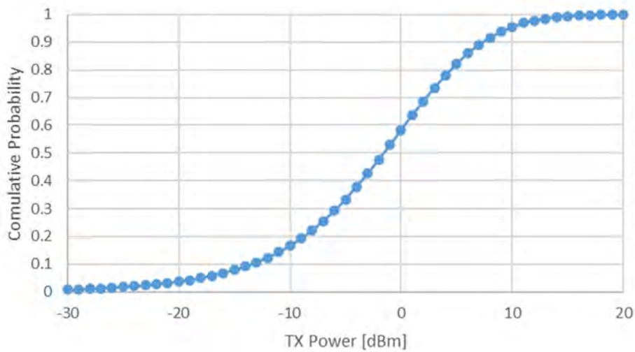
参図 2 - 9 TD-LTE 子機の送信電力分布
