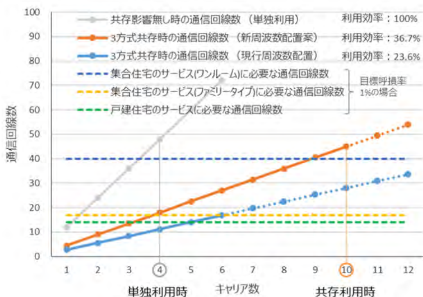
図2. 1-2 ワイヤレステレビドアホン全戸導入に必要なキャリア数概算
