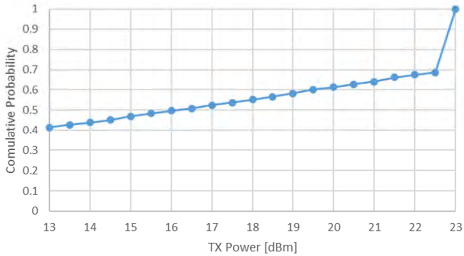
参図 2 - 8 TD-LTE 親機の送信電力分布
