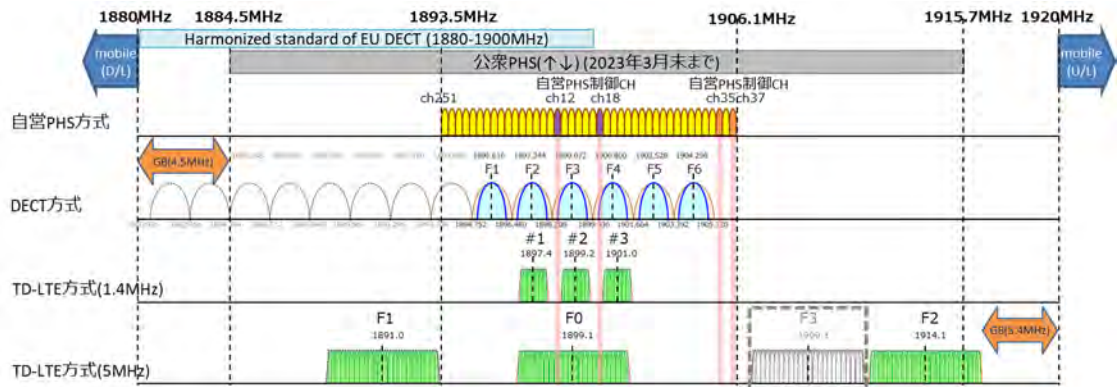
図 1. 2-15 現行周波数配置(DECT方式は6波、自営 PHS 制御チャンネル検出で4波に縮退)
