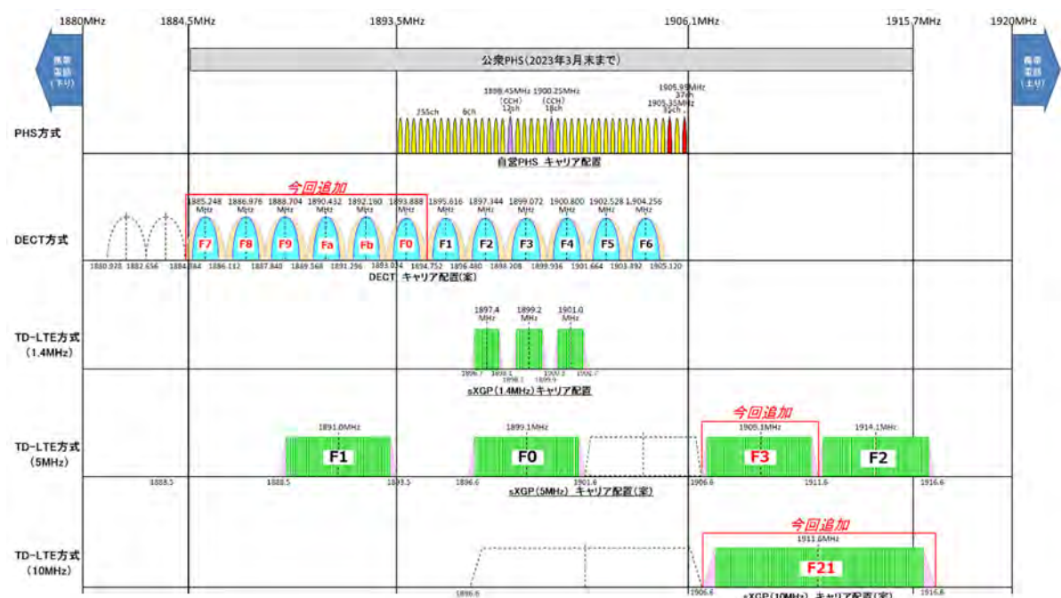
図 3. 1-1 TD-LTE 方式の周波数拡張案
