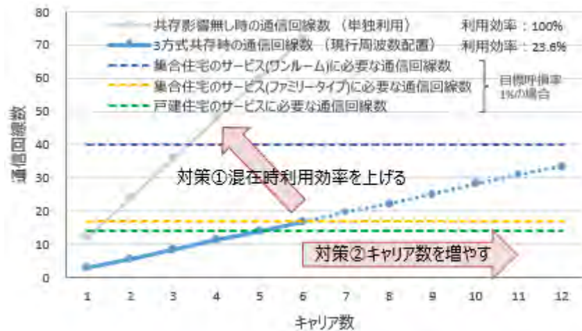
図 1. 2-14 ワイヤレステレビドアホン全戸導入に必要なキャリア数概算
