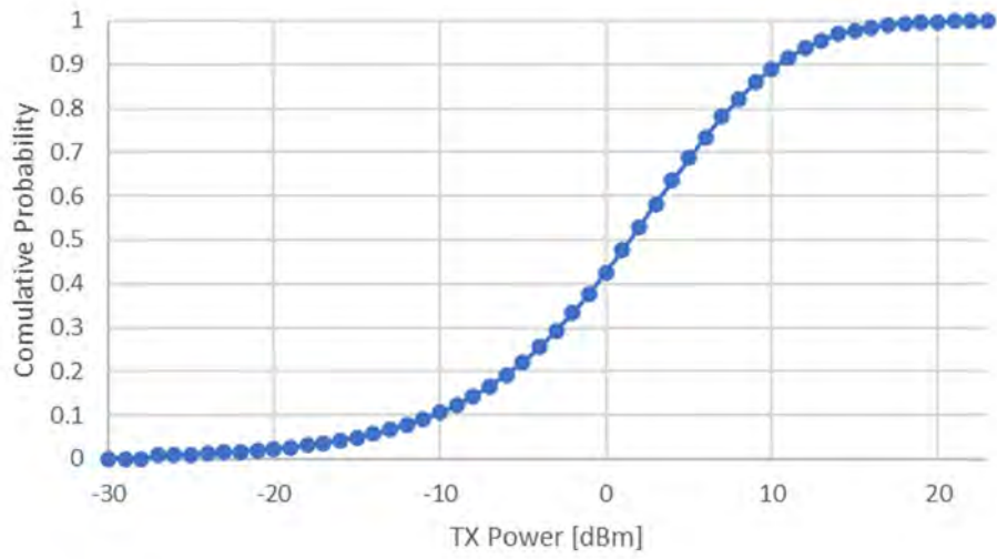
参図 2-20 携帯移動局の送信電力分布
