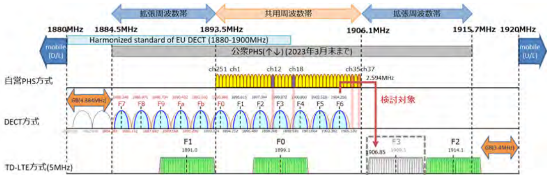
図 2. 2-5 DECT 方式の割当周波数と TD-LTE 方式の割当周波数との位置関係
