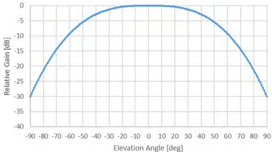
参図 2-7 TD-LTE 親機のアンテナ垂直指向特性 (送受信)
