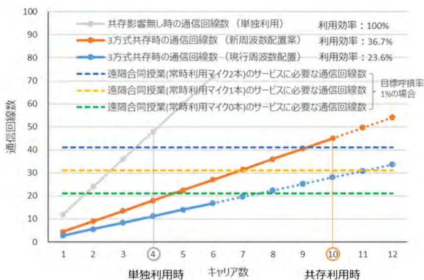
図2. 1-3 ワイヤレスマイクを全教室導入に必要なキャリア数概算
