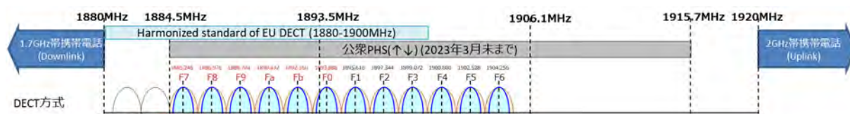
図4. 2-1 DECT方式のキャリア周波数
