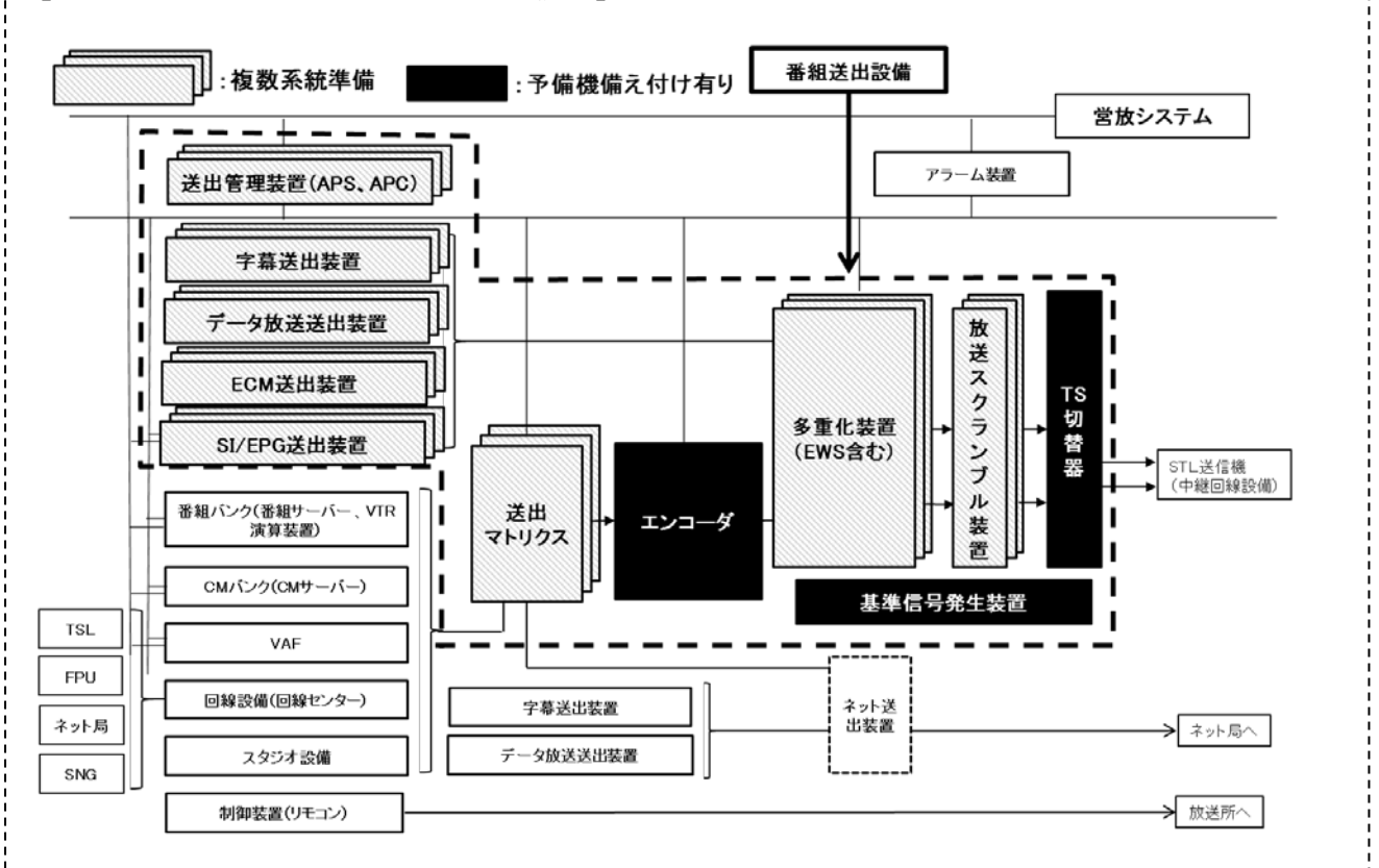
【番組送出設備に関する系統図の記載例】
