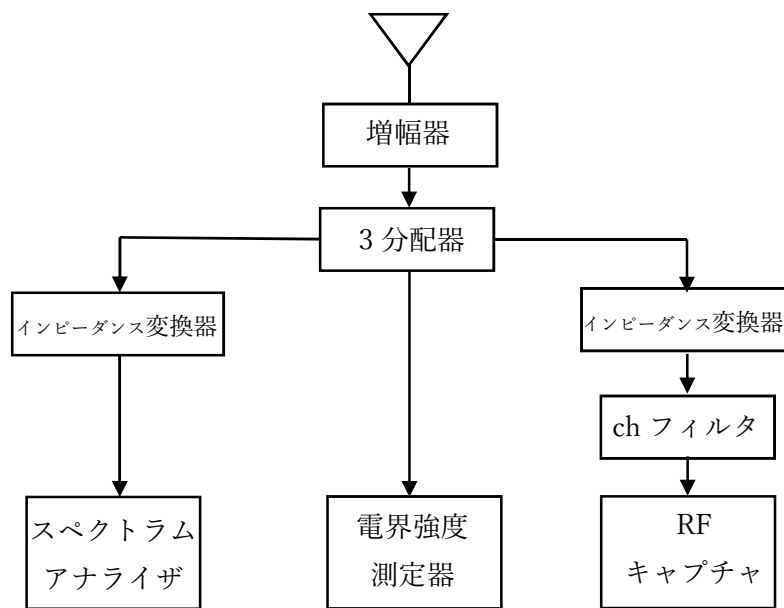
図 4.1-2 受信系統図
