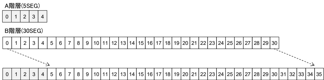
図 3.2.1.6.2.6-1 階層合成の信号処理手順
