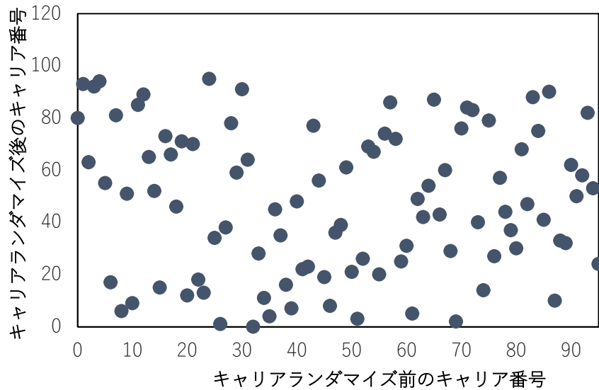
図 3.2.2.3.10.2-2 キャリア ランダム化前後のキャリア配列例
