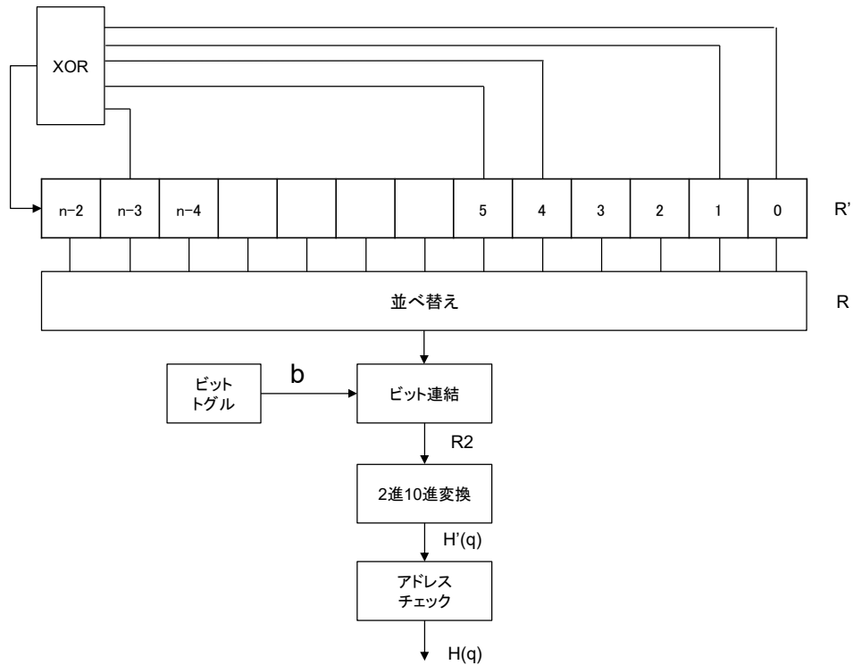
図 3.2.1.6.2.9.4.2-1 アドレス生成回路
