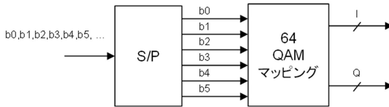
(d) 64QAM
