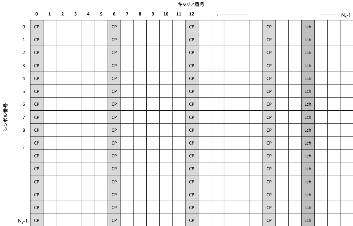
図 3.2.1.5.10-1 TMCC 区間の OFDM セグメント構成例
