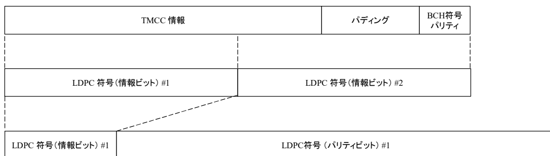
図 3.2.1.5.2-1 伝送制御情報の誤り訂正符号化
