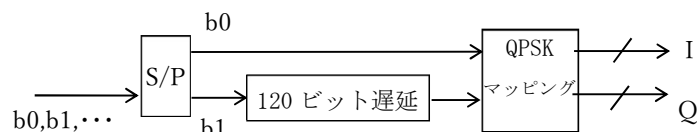
図3.2.2.3.7.3.1-1 QPSK変調系統図
