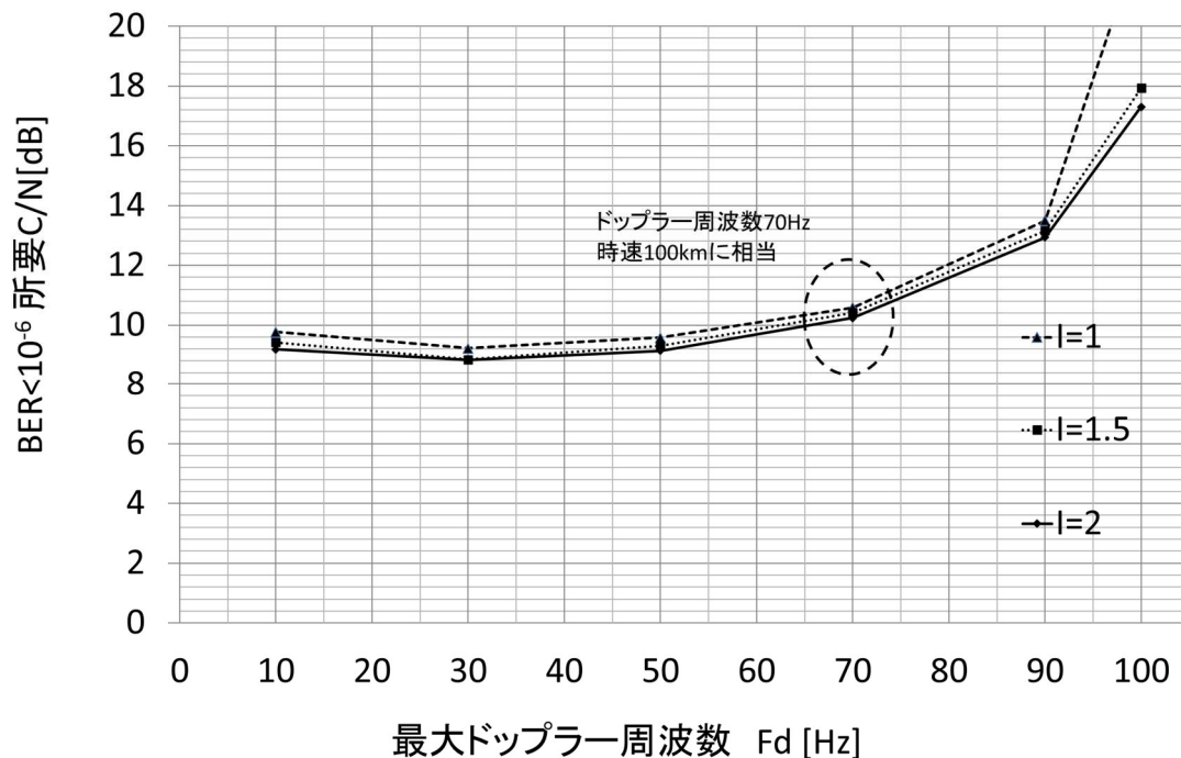
図 2-1 最大ドップラー周波数に対する所要 C/N(シミュレーション(TU6))
