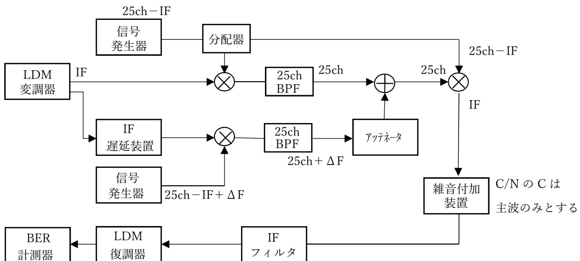
図 3-1 試験系統
