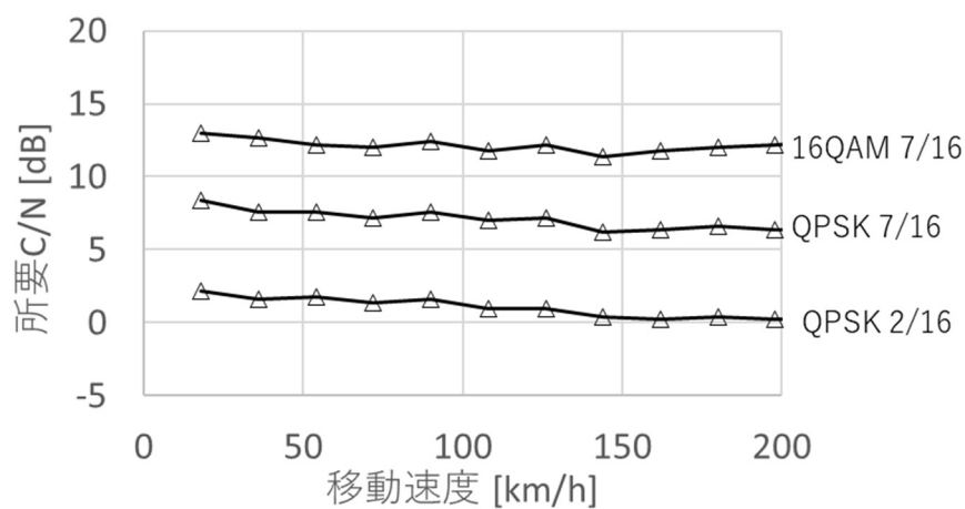
図 3-4 計算機シミュレーションにおける速度耐性の結果
