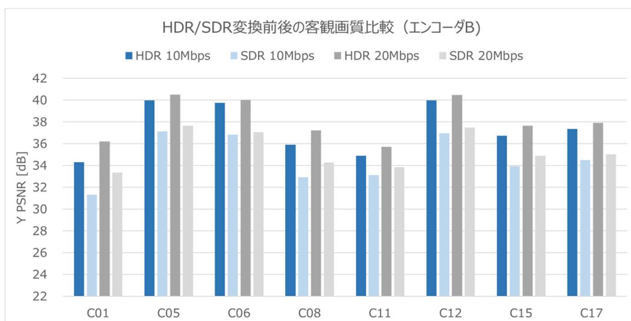
図 3-8 エンコーダ B における 2160/60/P, HDR 映像を SDR 変換した場合の客観画質の違い
