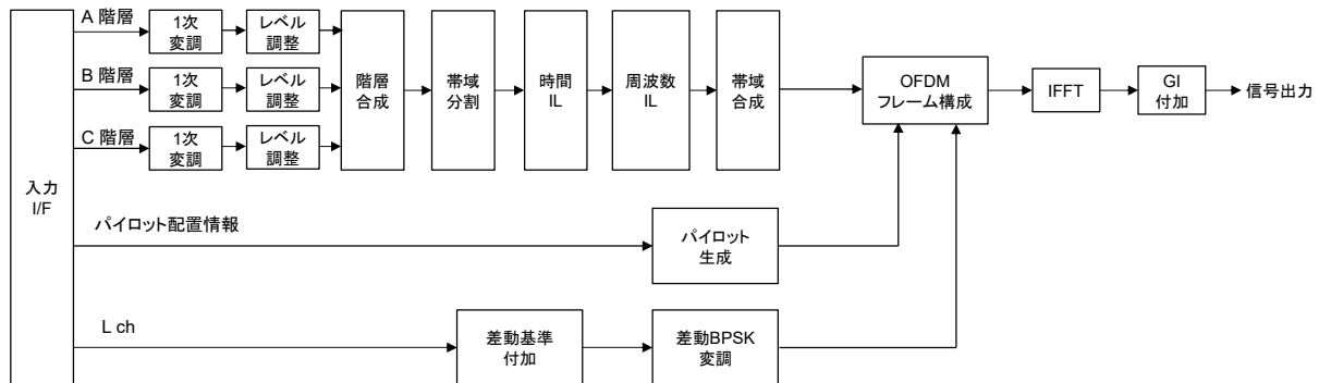
図 3.2.1.2.1-1 OFDM 変調部の構成
