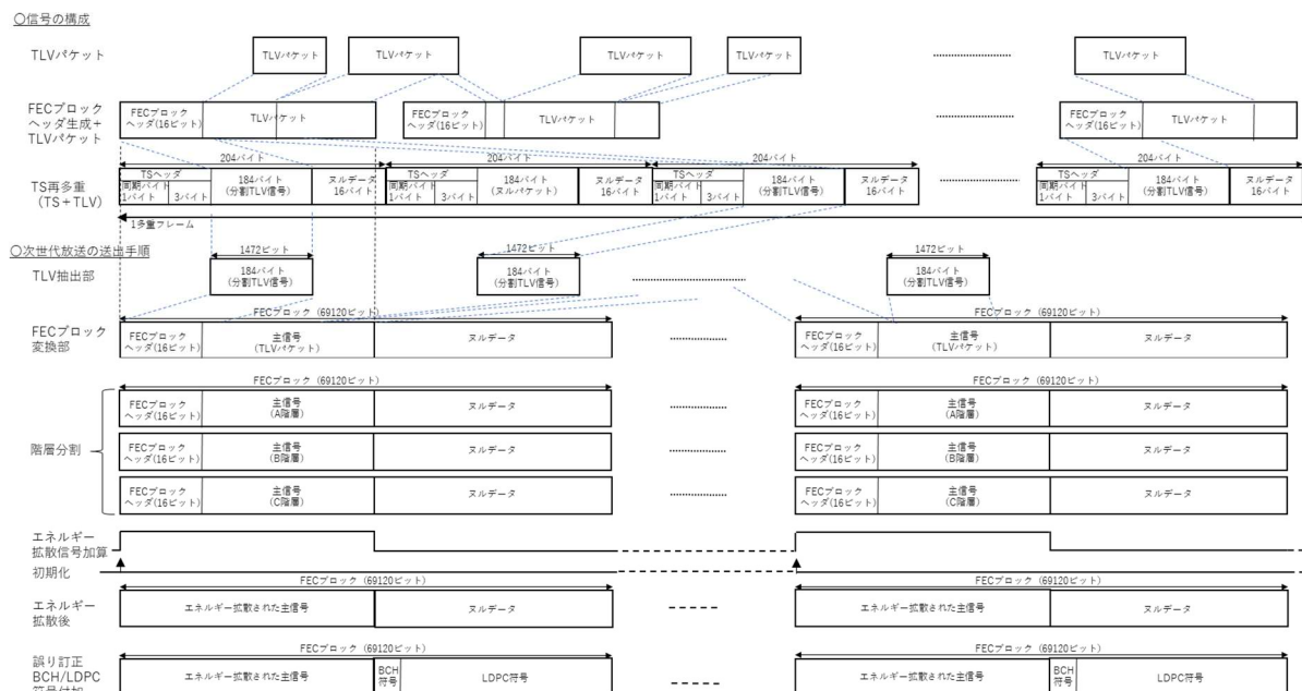
図 3.2.2.4-2 伝送主信号の構成及び送出手順（次世代放送時）
