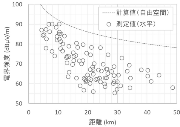
図 1-4 測定点の電界強度の測定結果 (水平偏波)
