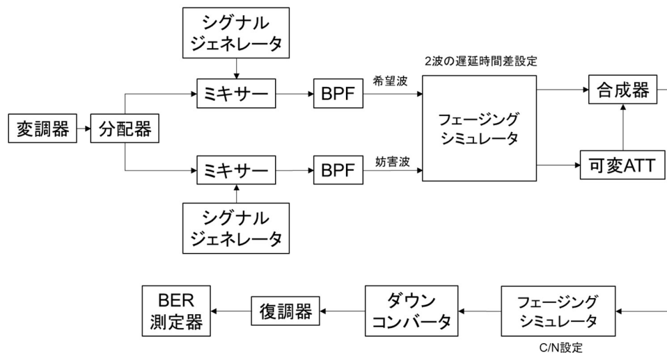
図 3-1 実験系統図
