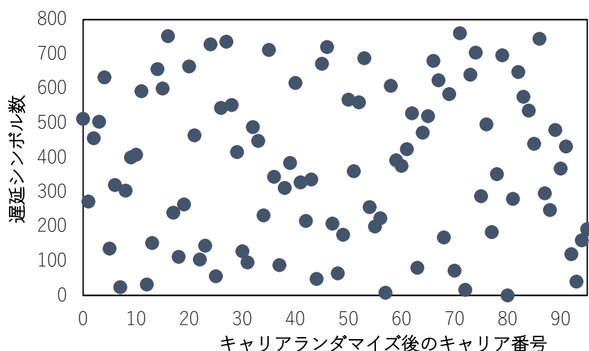
図 3.2.2.3.10.2-3 時間インターリーブ、キャリア ランダムイズ後の配列例
