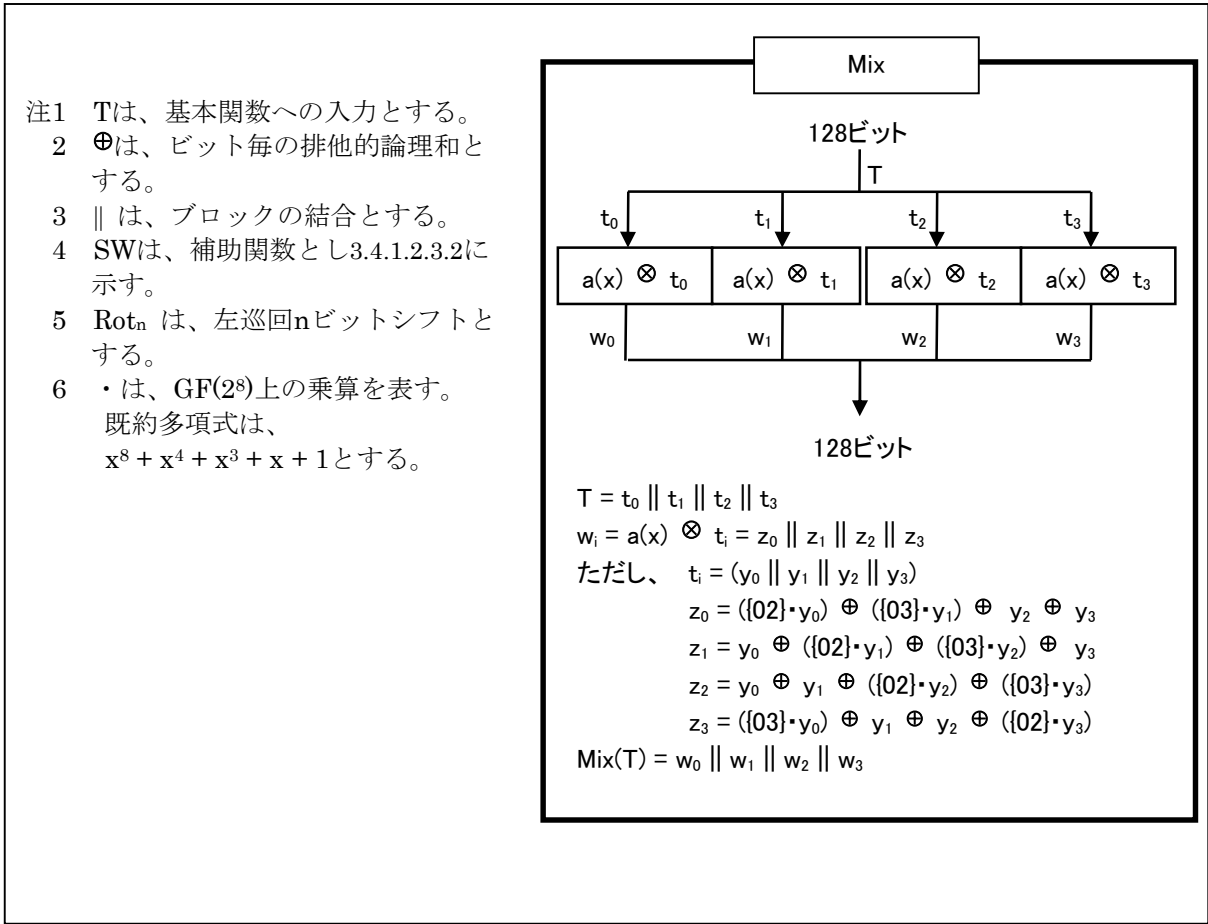
図 3. 4. 1. 2. 3. 1-2 AES 暗号の基本関数 (鍵長 256 ビットの場合)
