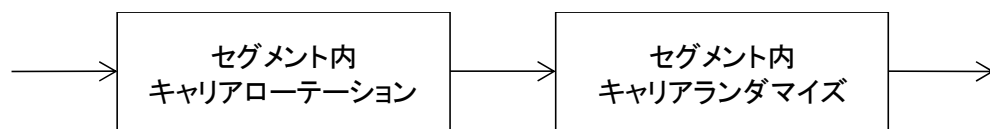
図 3.2.1.6.2.9.4-1 セグメント内インターリーブ
