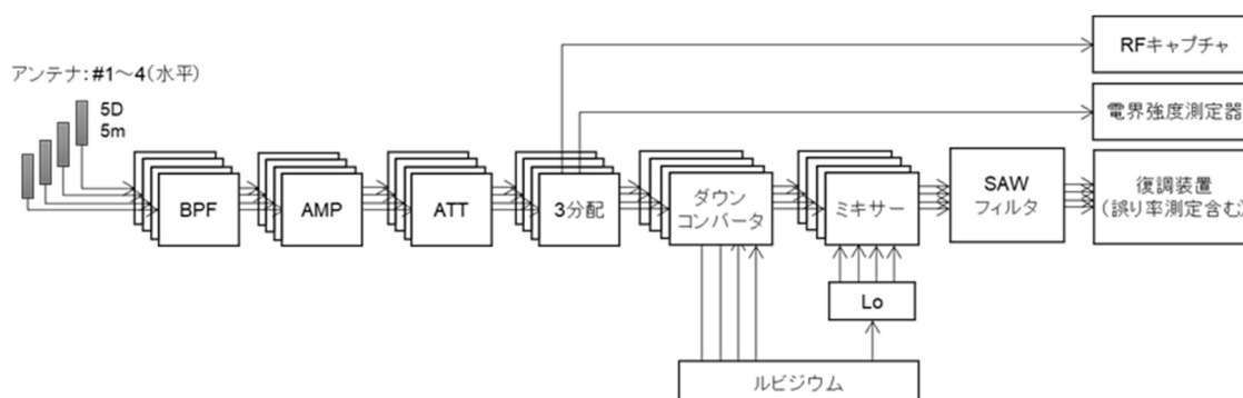
図 5-1 受信系統図
