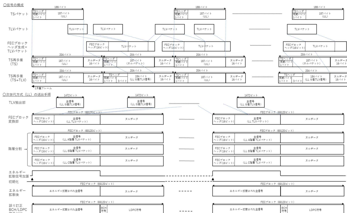
図 3.2.2.4-1 伝送主信号の構成及び送出手順 (LDM 放送時の LL)
