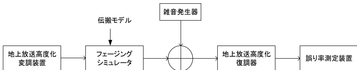
図 1-1 伝搬モデルを用いる場合の測定系
