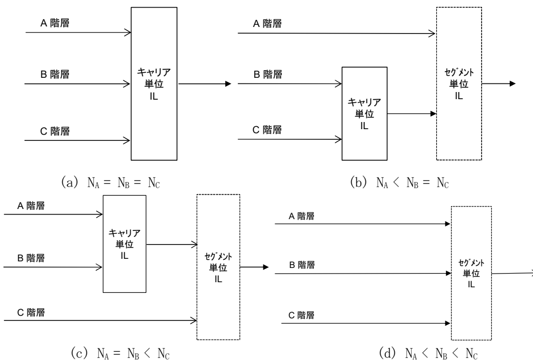
図 3.2.1.6.2.9.3-4 階層間インターリーブの入力が 3 階層
