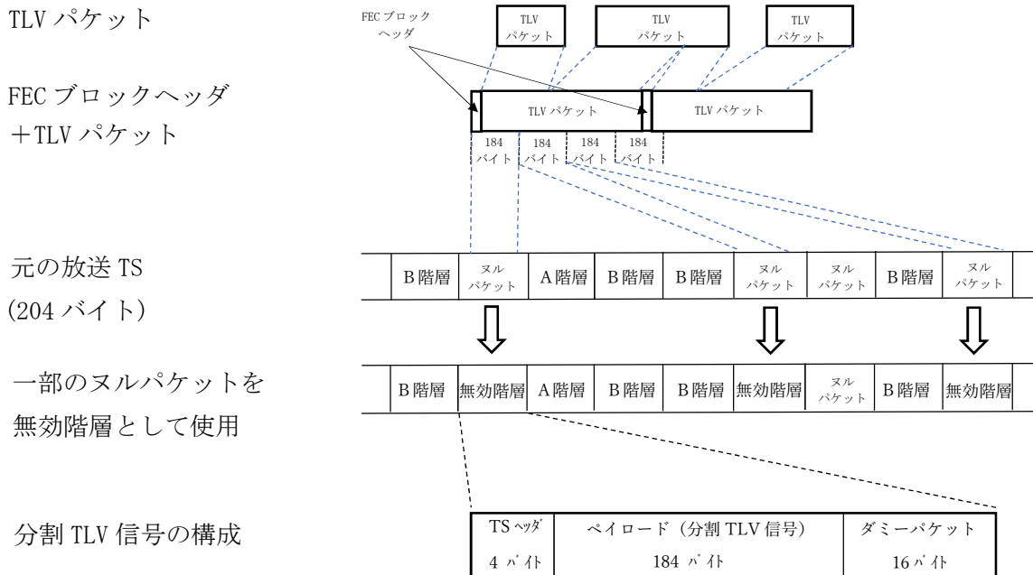
図 3.2.2.2.1-3 放送 TS への TLV 信号重畳法
