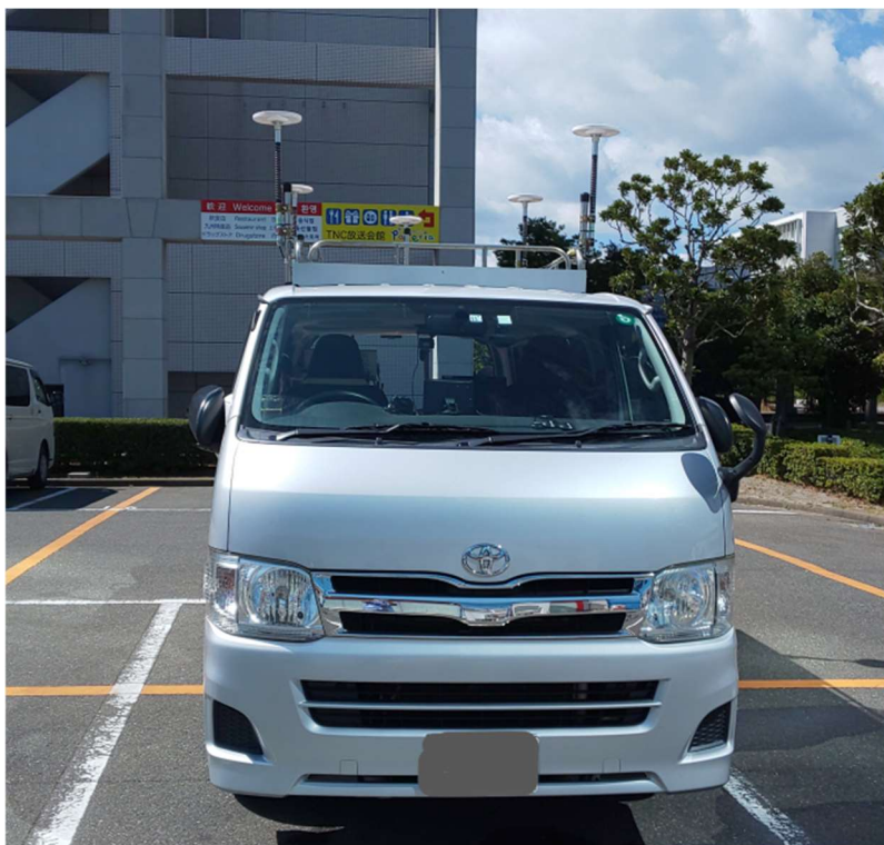
図 5. 4-1 正面から見た測定車 屋根の上にアンテナ 5 基を設置 4 基は ISDB-T 受信機用 / 1 基は LDM 復調器用
