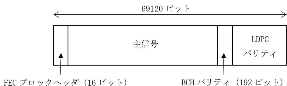
図 3.2.2.4.2.1-1 FEC ブロックの構成
