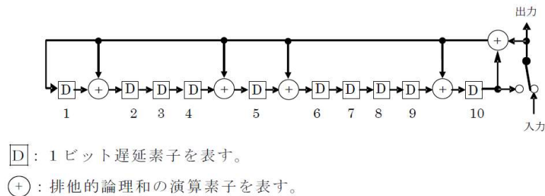
図 3.2.2.11.7.6-1 CRC の生成回路
