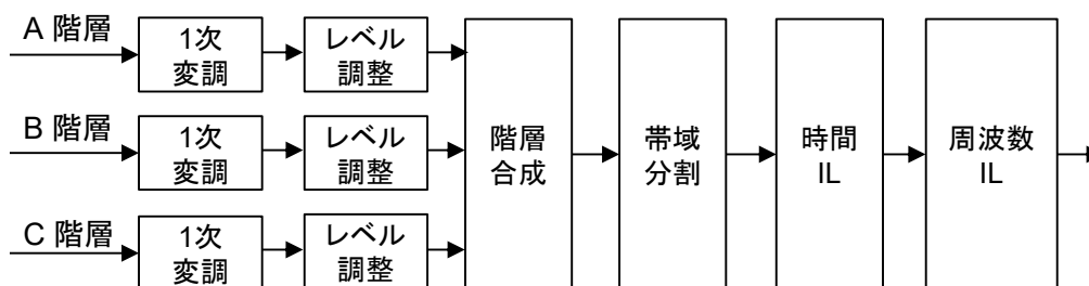
図 3.2.1.6.2.1-1 OFDM データセグメントの構成
