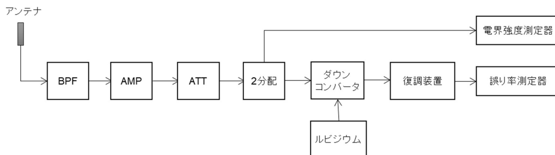
図 4-2 受信系統図 (移動受信環境における測定)
