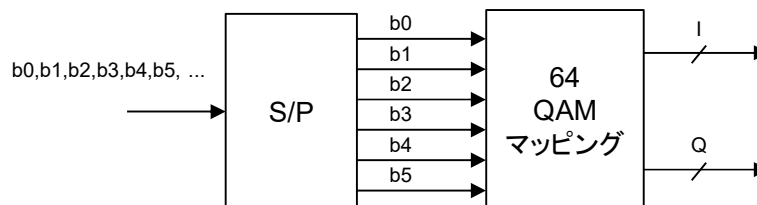
(d) 64 QAM
