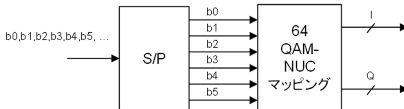
(e) 64QAM-NUC
