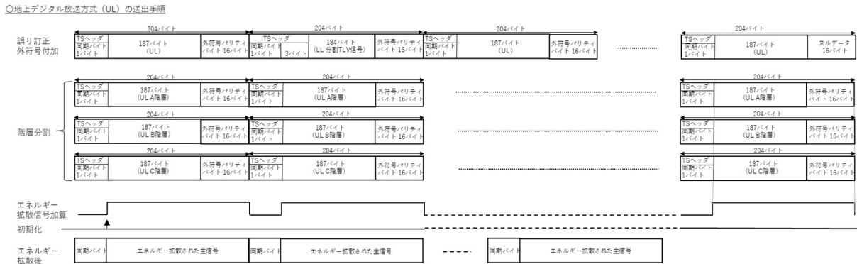
図 3.2.2.3-1 伝送主信号の構成及び送出手順 (LDM 放送時の UL)
