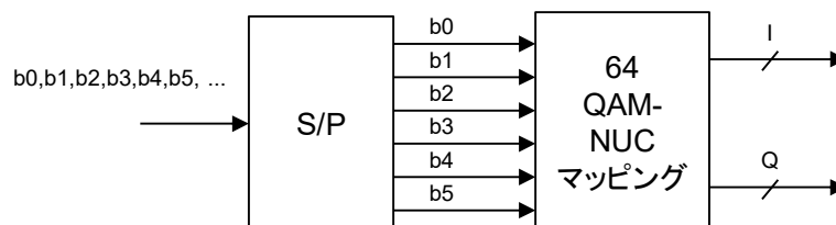
(e) 64 QAM-NUC
