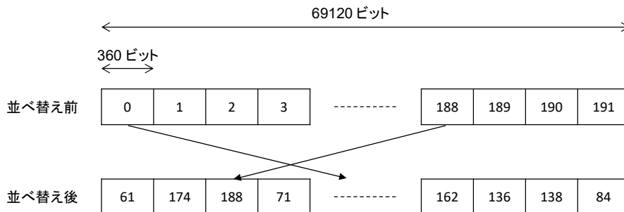
図 3.2.1.6.1.5.1-1 グループワイズインターリーブ (QPSK, 符号化率 2/16 の例)
