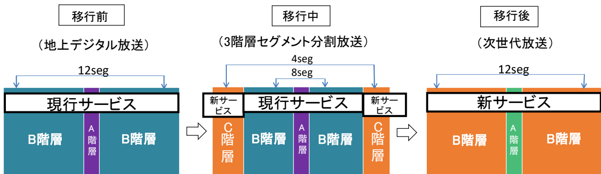
図 2.2-2 セグメント分割 SISO 方式の伝送構造（移行中から移行後）
