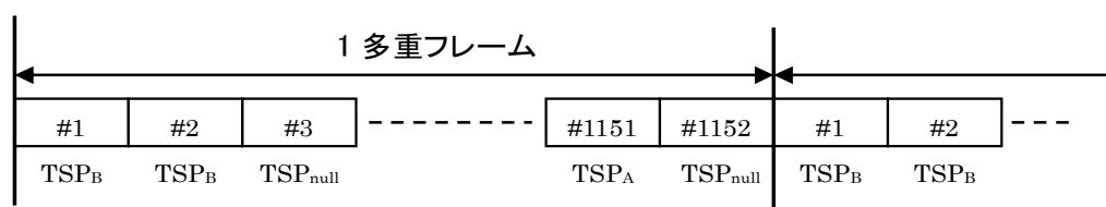
図 3.2.2.2.1-1 再多重されたトランスポートストリームの例 （モード 1、ガードインターバル 1/8 の場合）
