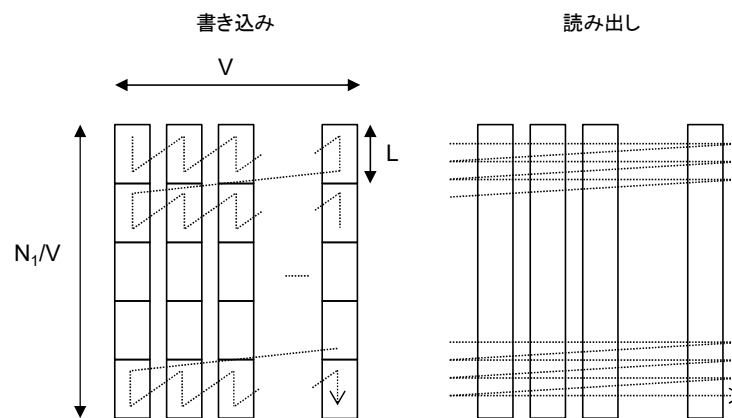
図 3.2.1.6.1.5.2-1 ブロックインターリーブ
