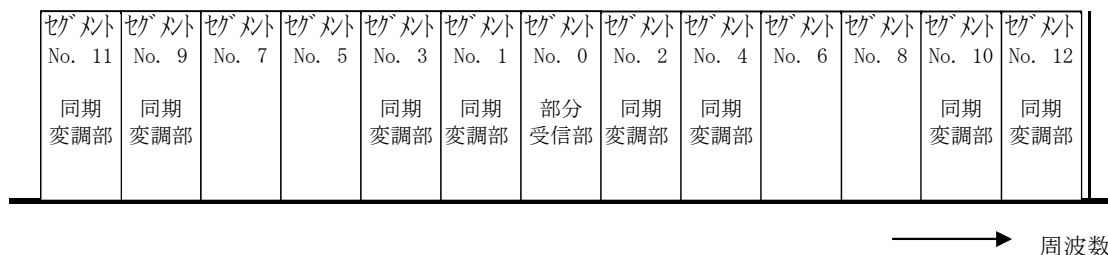
図 3.2.2.8-1 伝送スペクトル上の OFDM セグメント番号と使用例
