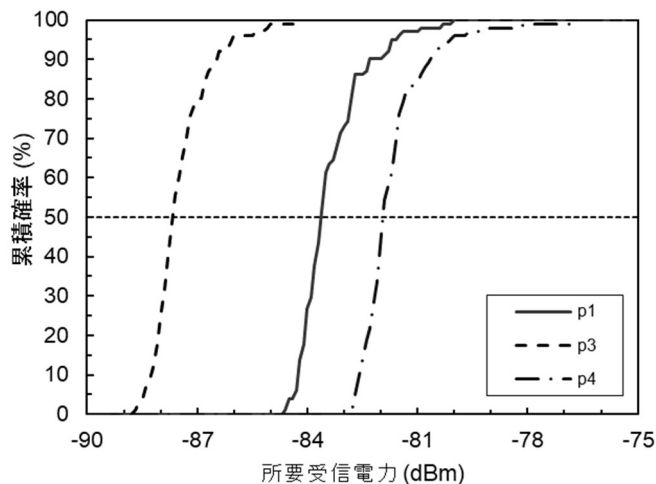
図 2-5 所要受信電力の累積確率
