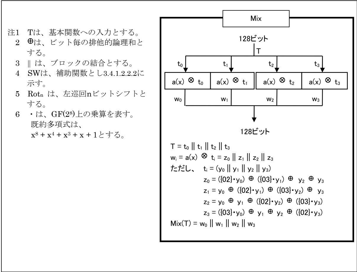
図 3. 4. 1. 2. 2. 1-2 AES 暗号の基本関数 (鍵長 192 ビットの場合)
