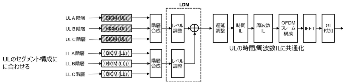
図 2.1-1 時間/周波数 IL の共通化
