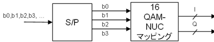
(c) 16QAM-NUC
