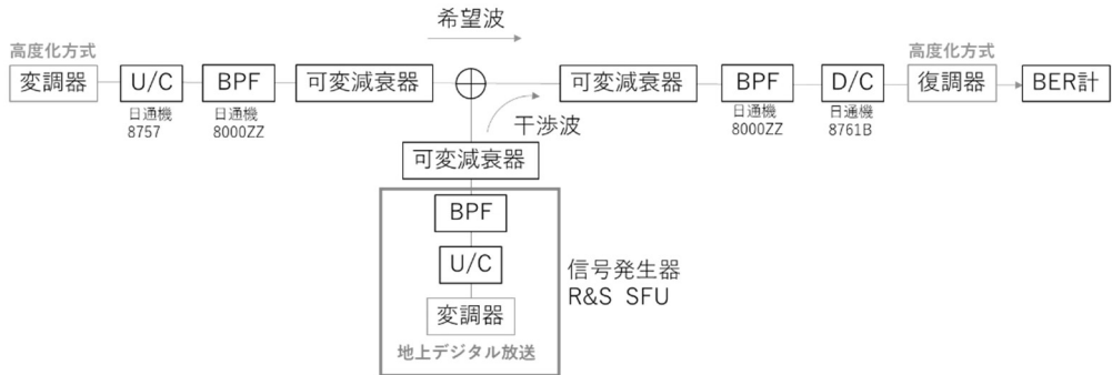
図 3-1 測定系統図
