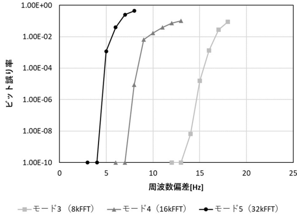
図 3-5 周波数偏差に対する BER 特性 モードによる比較 (1024QAM 符号化率 12/16 C/N=30 dB)
