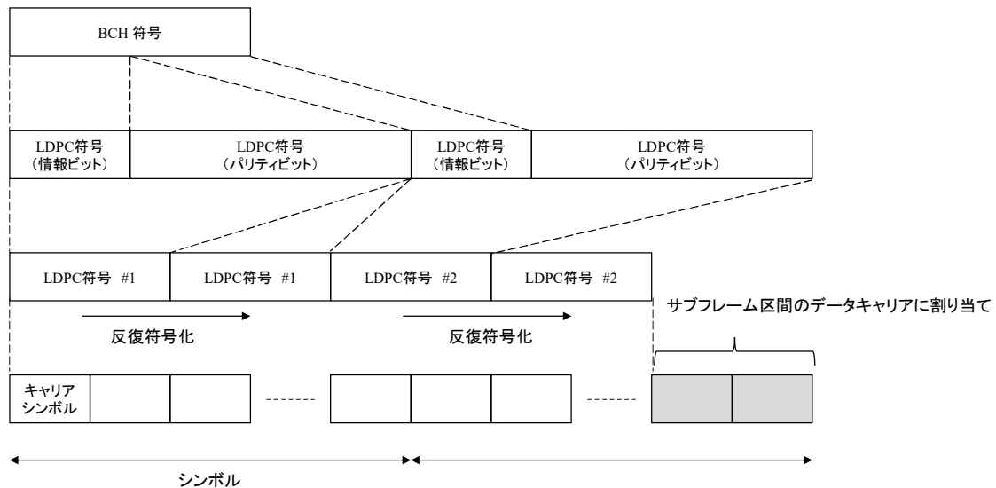
図 3.2.1.5.5.3-1 反復符号化
