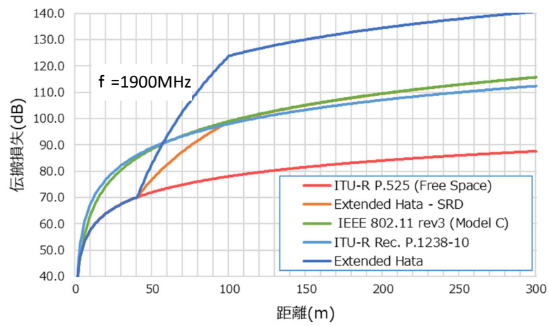
参図 1 - 1 伝搬モデルごとの距離／伝搬損特性
