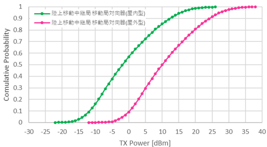
参図 2-22 陸上移動中継局（移動局対向器 屋内型／屋外型）の送信電力分布
