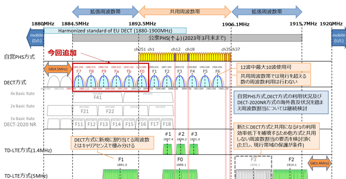
図 1. 2-18 1.9GHz 帯全体の基本周波数配置案
