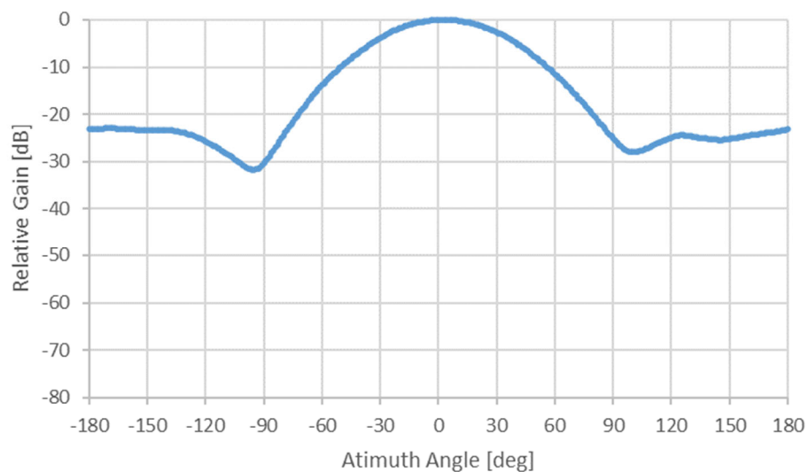
参図 2-14 小電力レピータ（基地局対向器）のアンテナ指向特性（水平）
