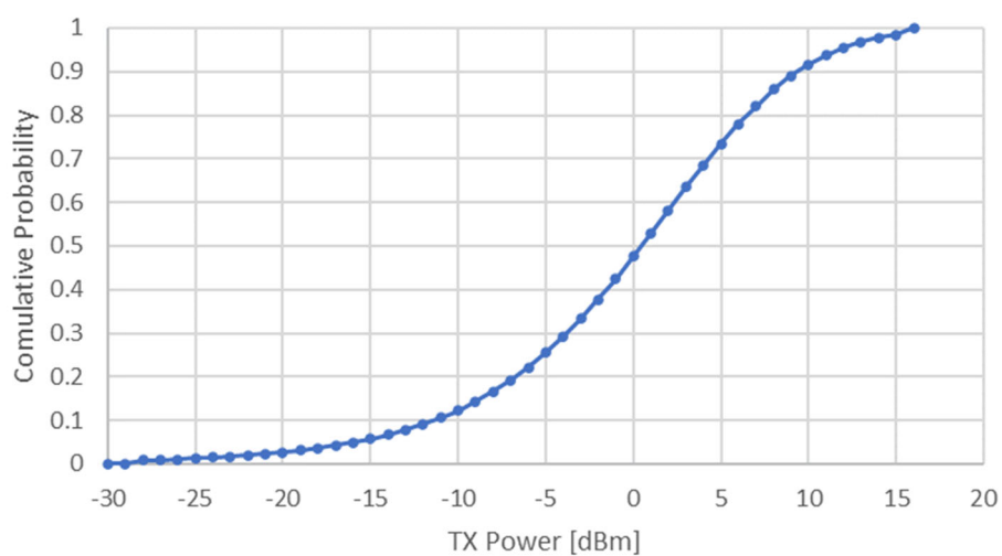
参図 2-23 小電力レピータ（基地局対向器）の送信電力分布
