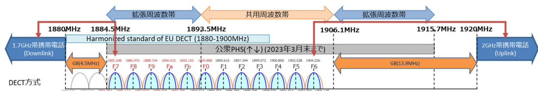
図 2. 2-7 DECT 方式と隣接する携帯電話との周波数位置関係
