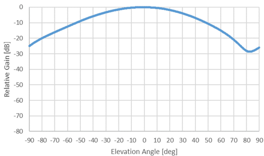
参図 2-15 小電力レピータ（基地局対向器）のアンテナ指向特性（垂直）
