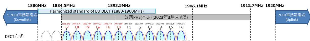
図4. 2 - 1 DECT方式の周波数
