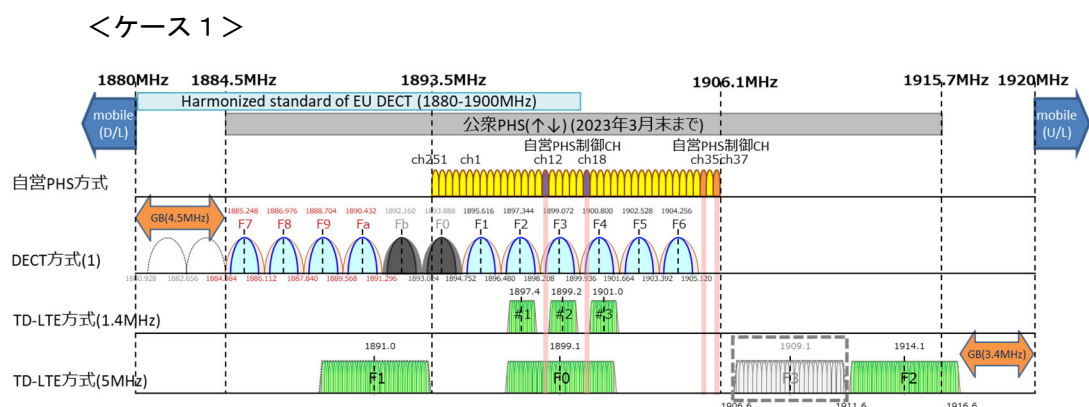
図 2. 2-1 DECT 方式(1)の周波数配置
