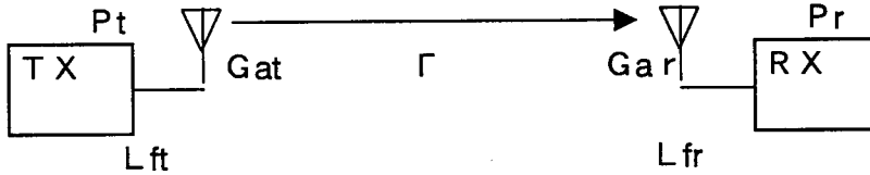
図 1.4 伝搬モデル
