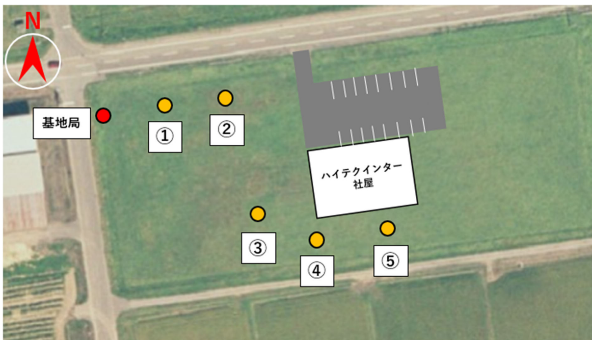
図 3.4-4 上空の測定ポイント
