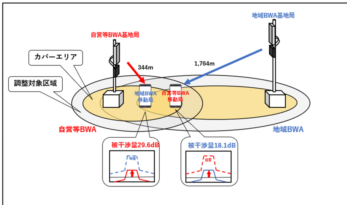
図 5.4-1 基地局－移動局間の干渉イメージ
