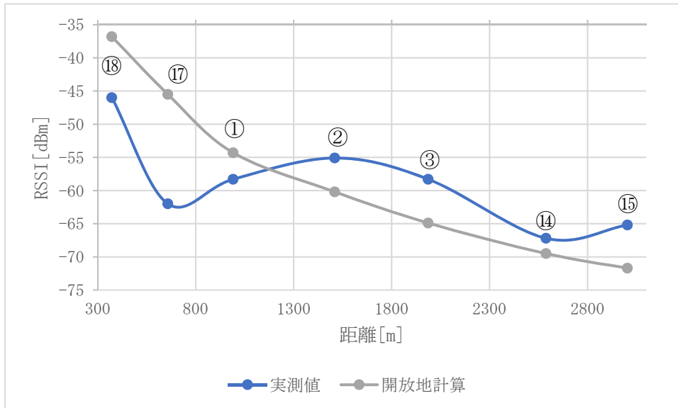
図 3.1-3 圃場の RSSI
