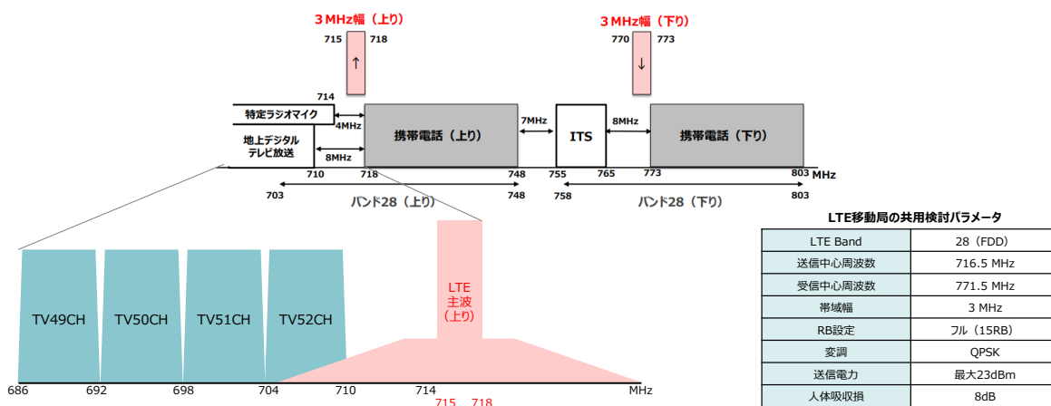
図 2. 3. 4. 1-2 実証実験概要
