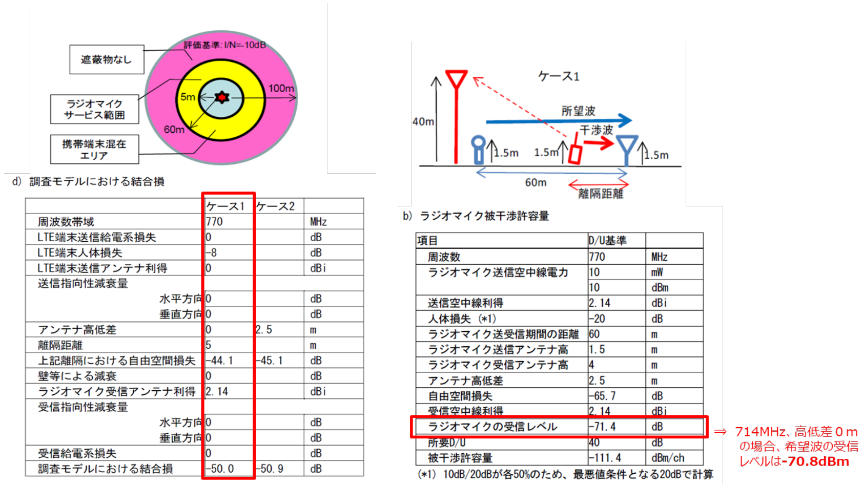
図2.4.4.1-7 検討モデル
