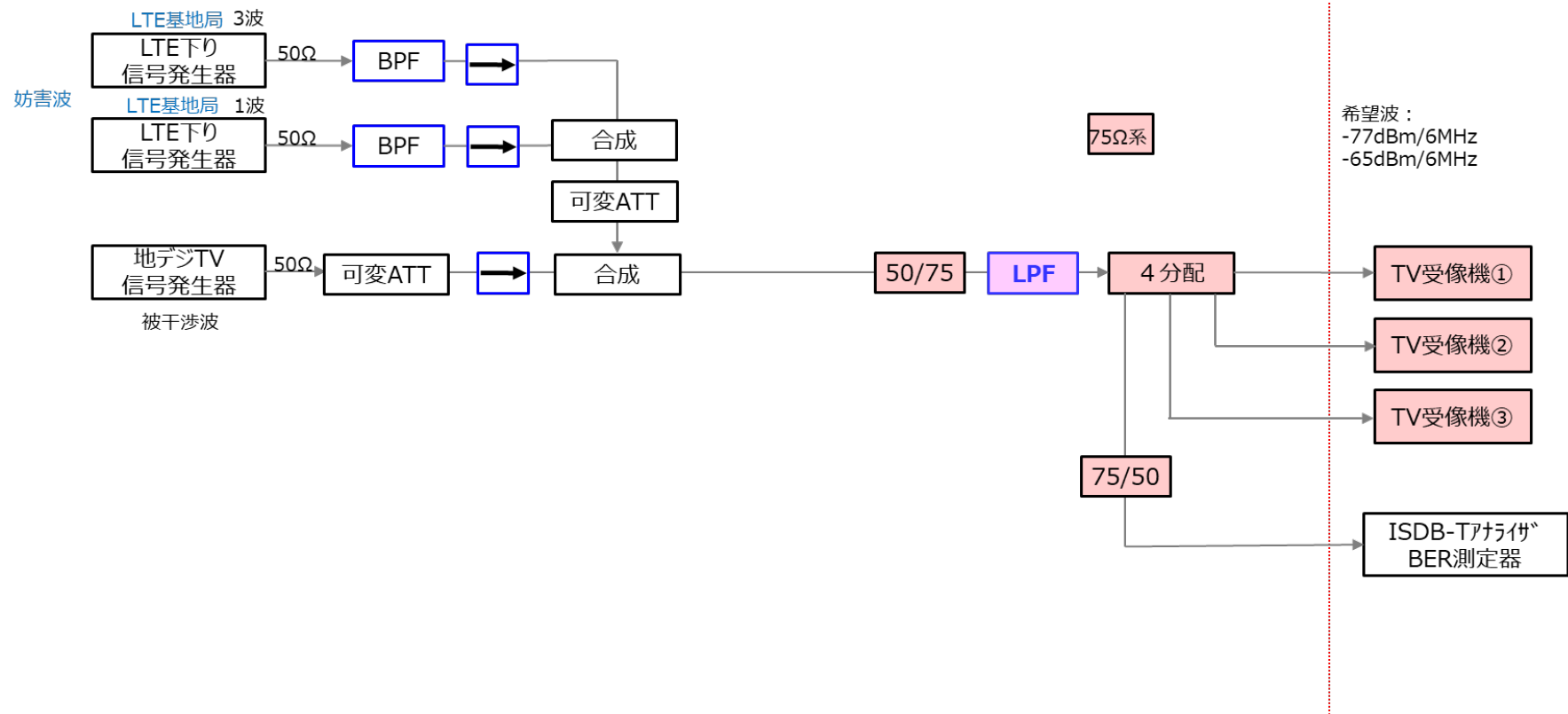
(d) TV-4の実験系 (フィルタ)
