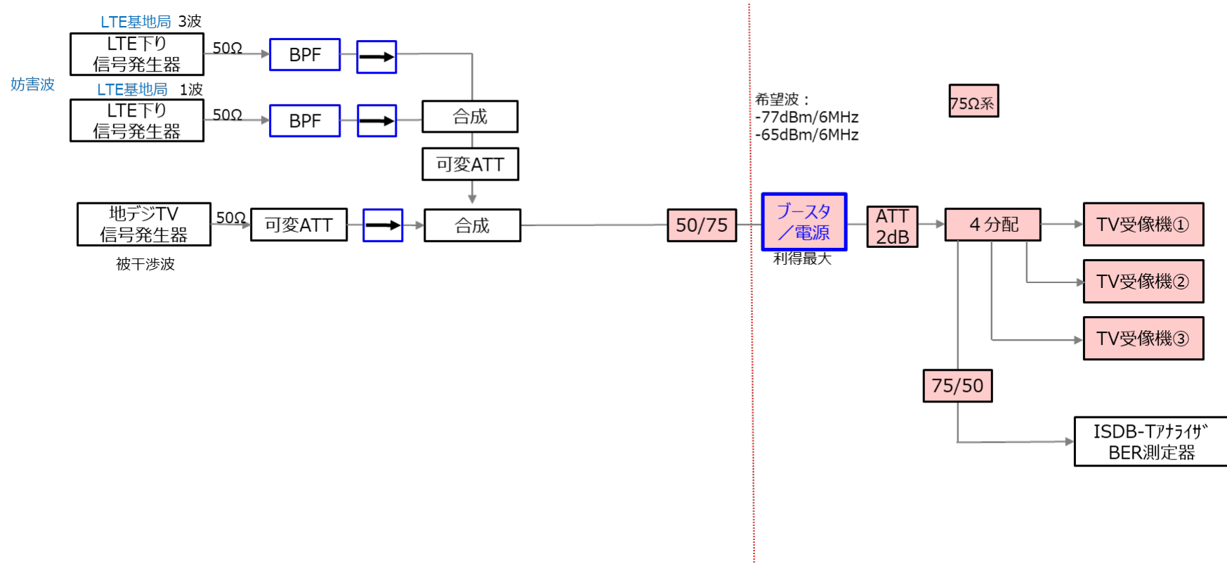
(e) TV-4の実験系（ブースタ）
