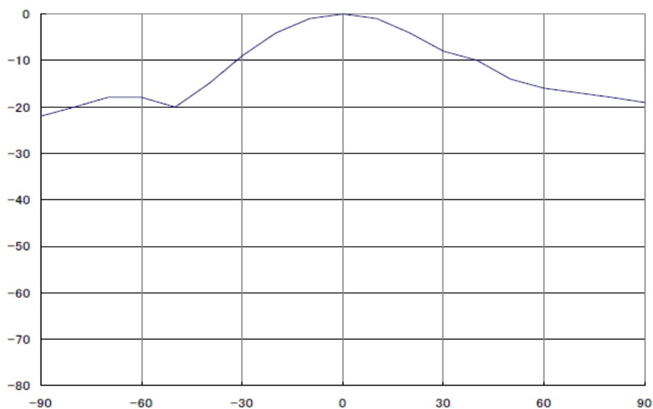
図 2. 2. 3 - 6 狭帯域 LTE-Advanced 陸上移動中継局（屋内エリア用） 基地局対向器アンテナ指向特性（垂直） （「携帯電話等高度化委員会報告」（平成 24 年 2 月 17 日）図 2. 2. 3 - 6 を引用）
