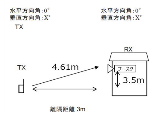
検討モデル案④ 家庭TV 簡易ANTブースタ有(飽和無)(5mH)
