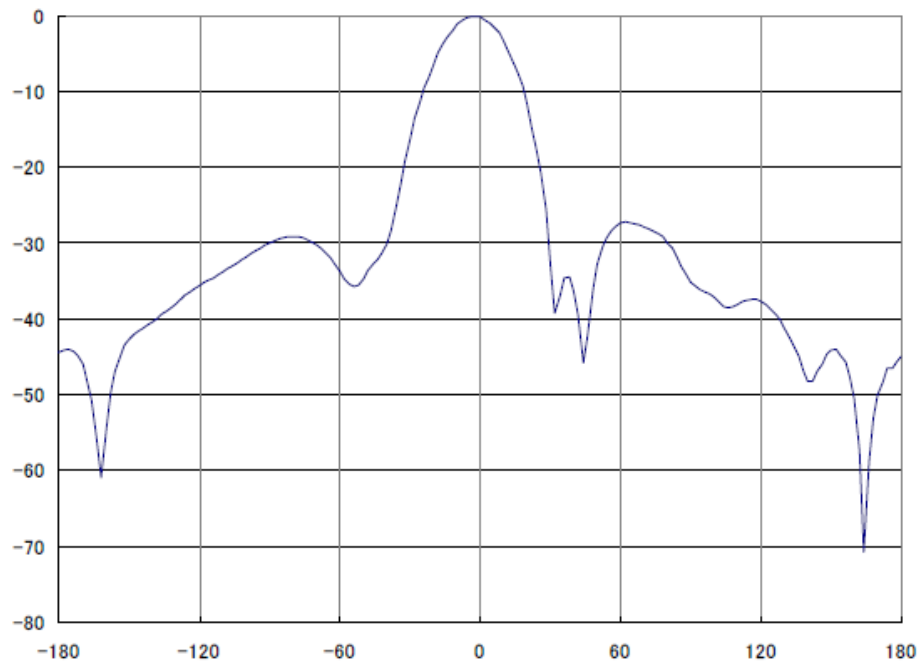
図 2. 2. 3 - 3 狭帯域 LTE-Advanced 陸上移動中継局（屋外エリア用） 基地局対向器アンテナ指向特性（水平）
