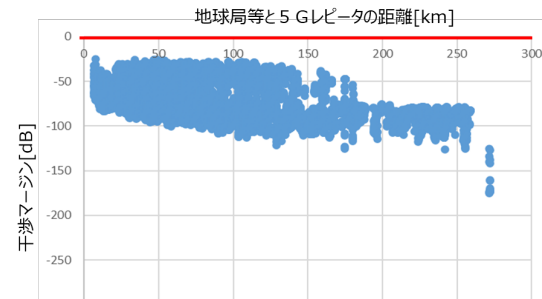
図3.3.1.4-18 下りの干渉マージン(短時間) (横浜、8台/局、11dBm/MHz、全て屋内設置)
