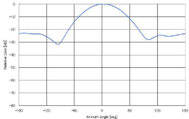
図3. 2. 3-1 基地局対向器のアンテナの指向特性(水平)
