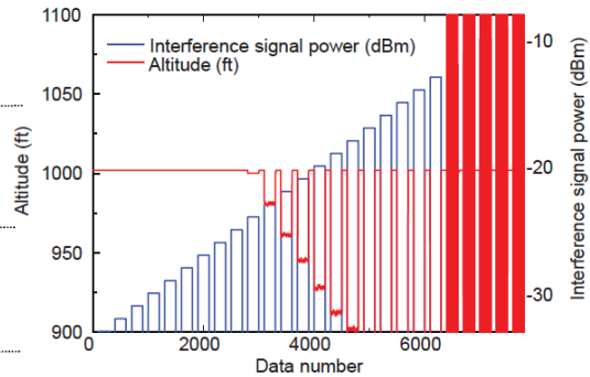
測定結果例 帯域外干渉測定・高度1,000 ft 干渉発生しきい値-23 dBm(高度MEおよび高度CDF)、12 dBm(NCD)
