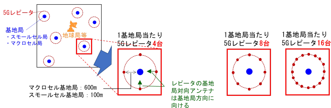
図 3. 3. 1. 2-1 5Gレピータから地球局等への干渉計算モデル
