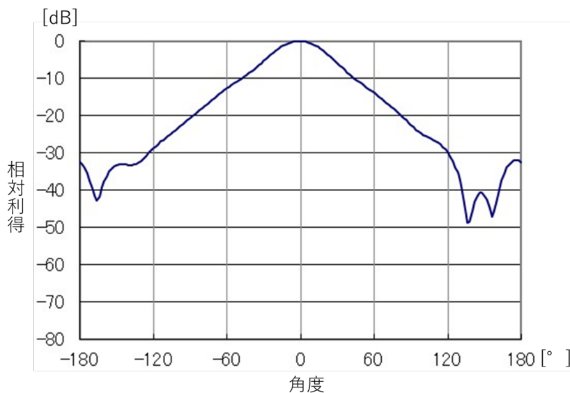
(a) 屋外エリア用（水平面）
