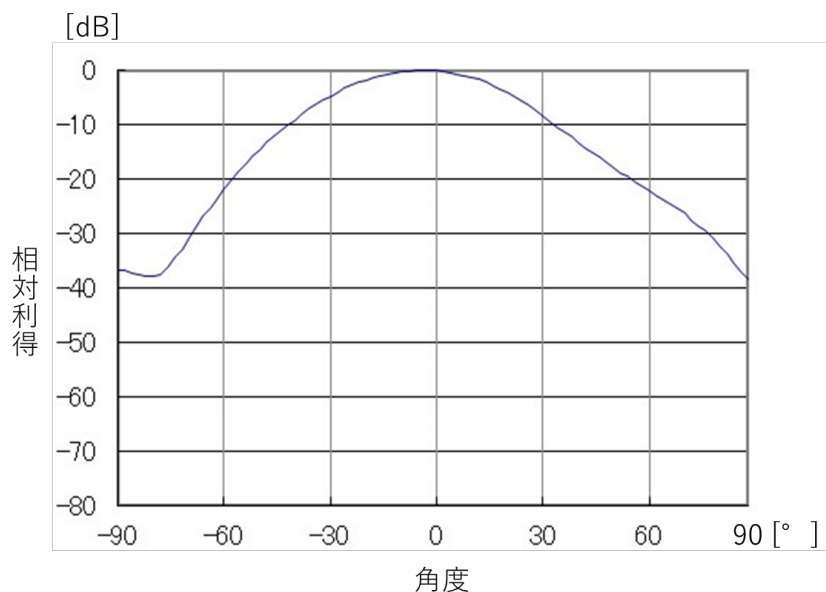
(b) 屋外エリア用（垂直面）
