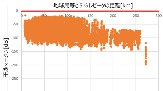
図3.3.1.4-17 上りの干渉マージン(短時間) (横浜、8台/局、11dBm/MHz、全て屋内設置)
