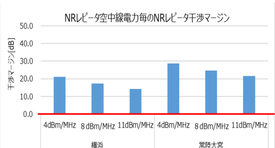
図 3. 3. 1. 4-5 送信電力ごとの干渉マージン(単体)
