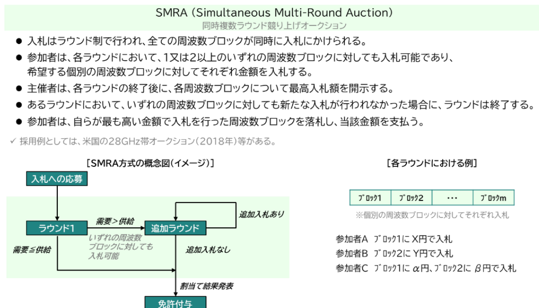
図表 5 - 1 SMRA（同時複数ラウンド競り上げオークション）概要
