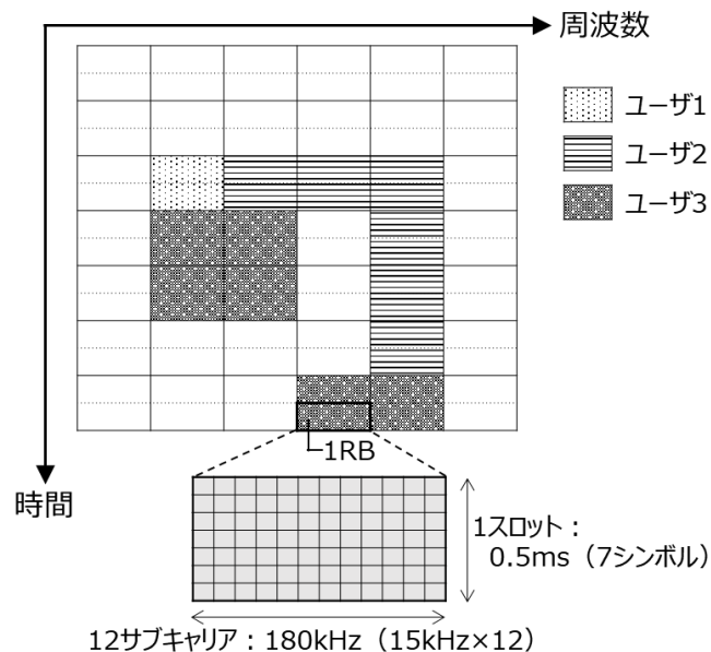
図 1. 2. 1. 2-1 LTE システムにおけるリソースブロック割当のイメージ
