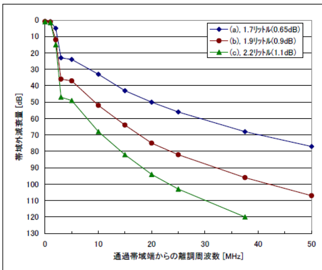
図2. 2. 1－3 狭帯域 LTE-Advanced 基地局/陸上移動中継局の送受信フィルタ特性 （「携帯電話等高度化委員会報告」（平成24年2月17日）図2. 2. 1－3を引用）
