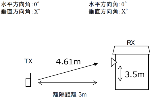
検討モデル案 ③ 家庭TV 簡易ANT ブースタ無 (5mH)
