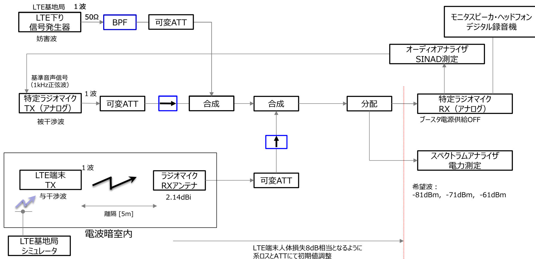
(a) RM-1の実験系 (アナログラジオマイク (ブースタ無))
