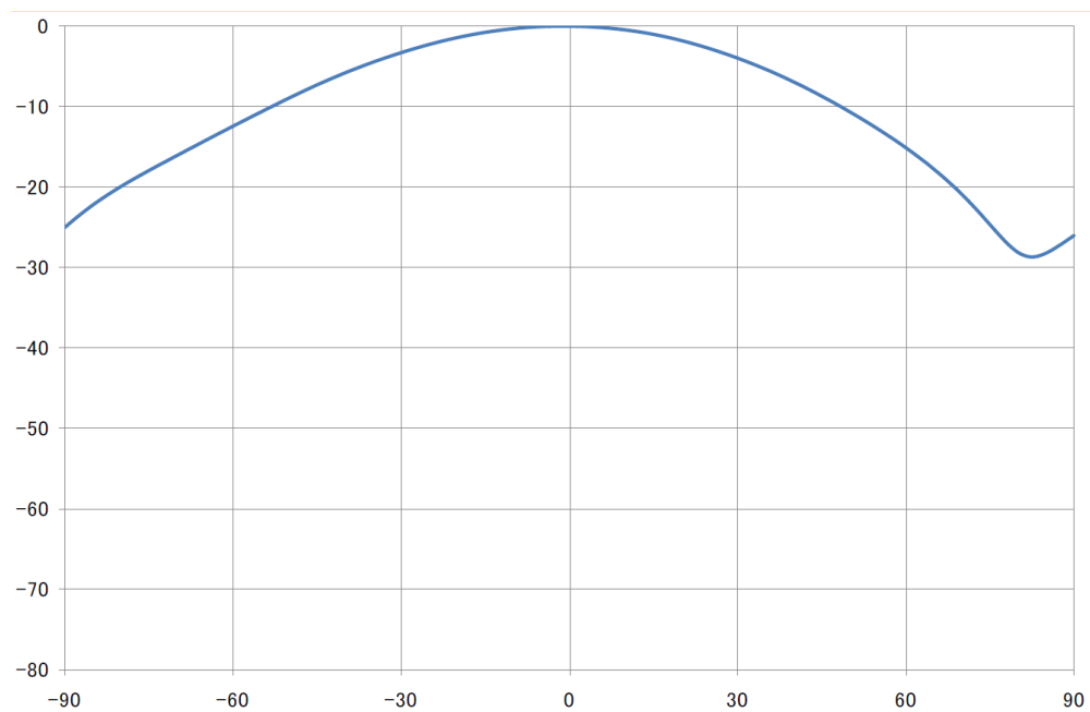
図2. 2. 4－2 狭帯域LTE-Advanced 小電力レピータ基地局対向器アンテナ指向特性（垂直） （「携帯電話等高度化委員会報告」（平成24年2月17日）図2. 2. 4－2を引用）
