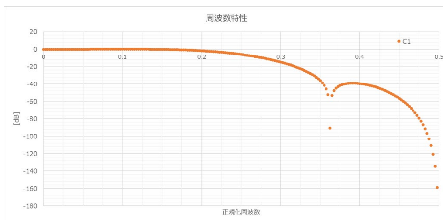
図 8-5 1/2 縮小フィルタの周波数特性
