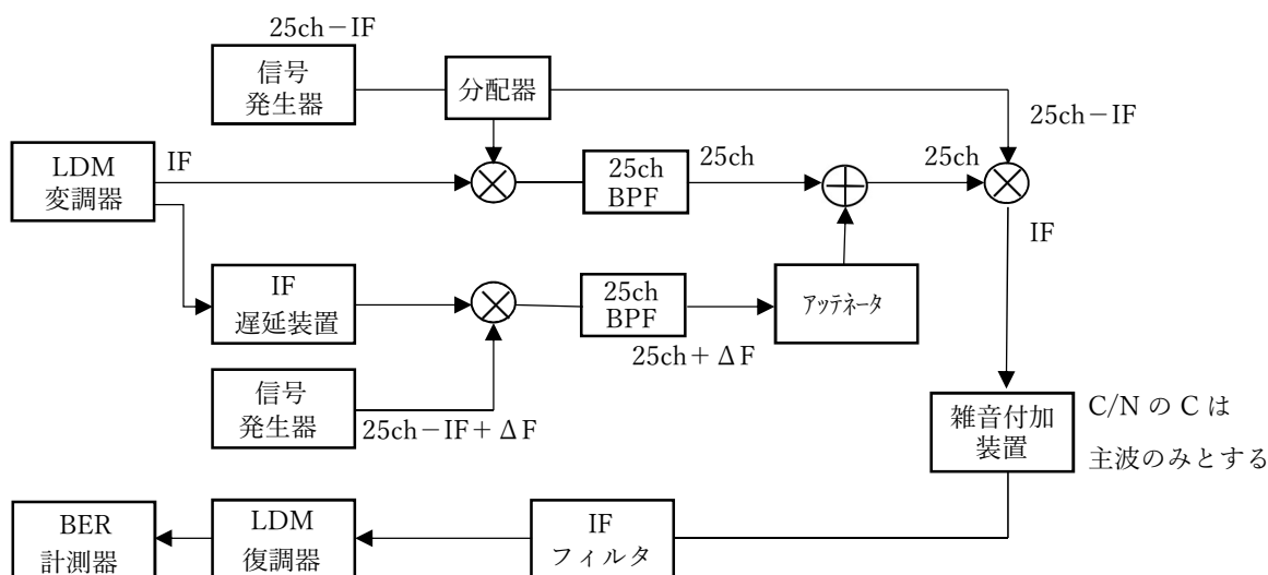
図 3-1 試験系統
