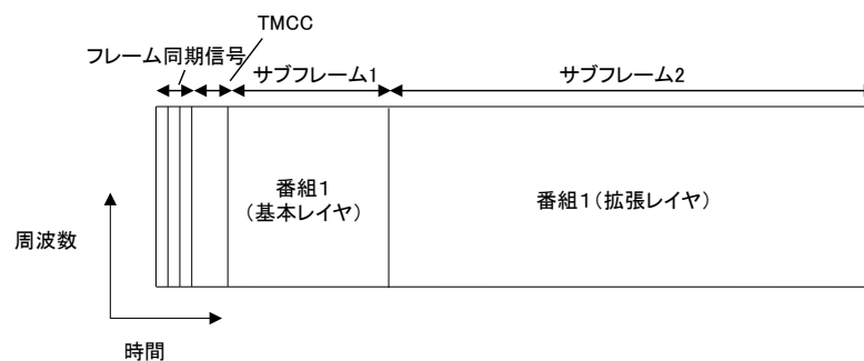
図 4.1-7 情報源符号化が階層符号化の構成例 2
