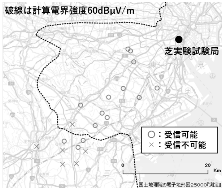
図 6-1 受信可否の結果
