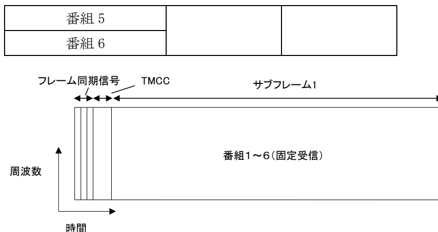
図 4.1-10 6 番組の構成例
