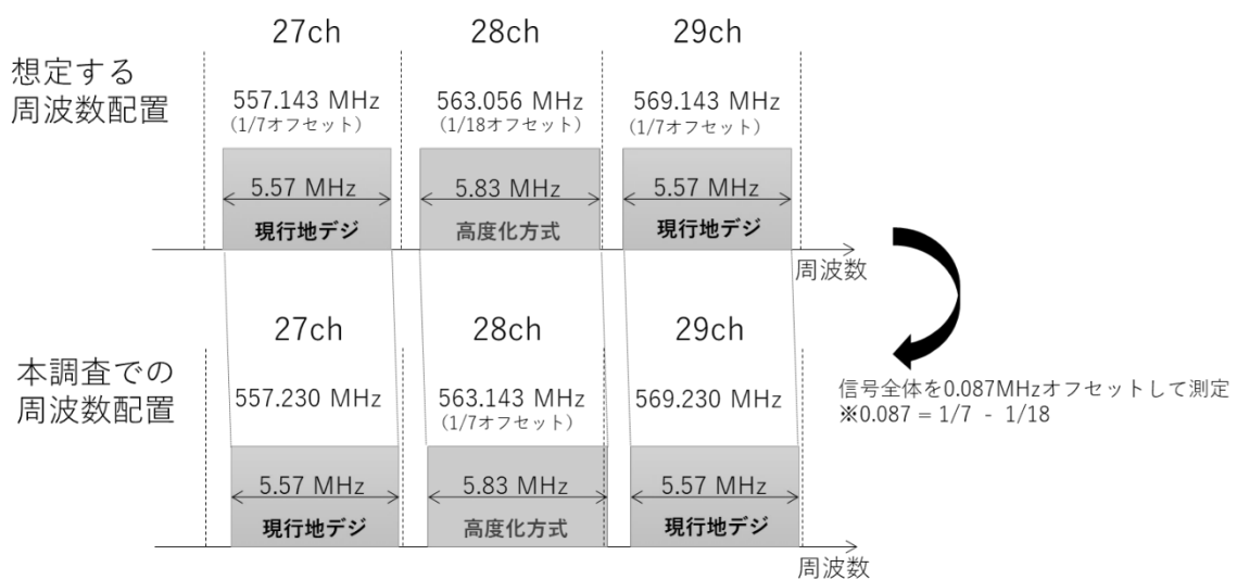
図 3-2 周波数配置
