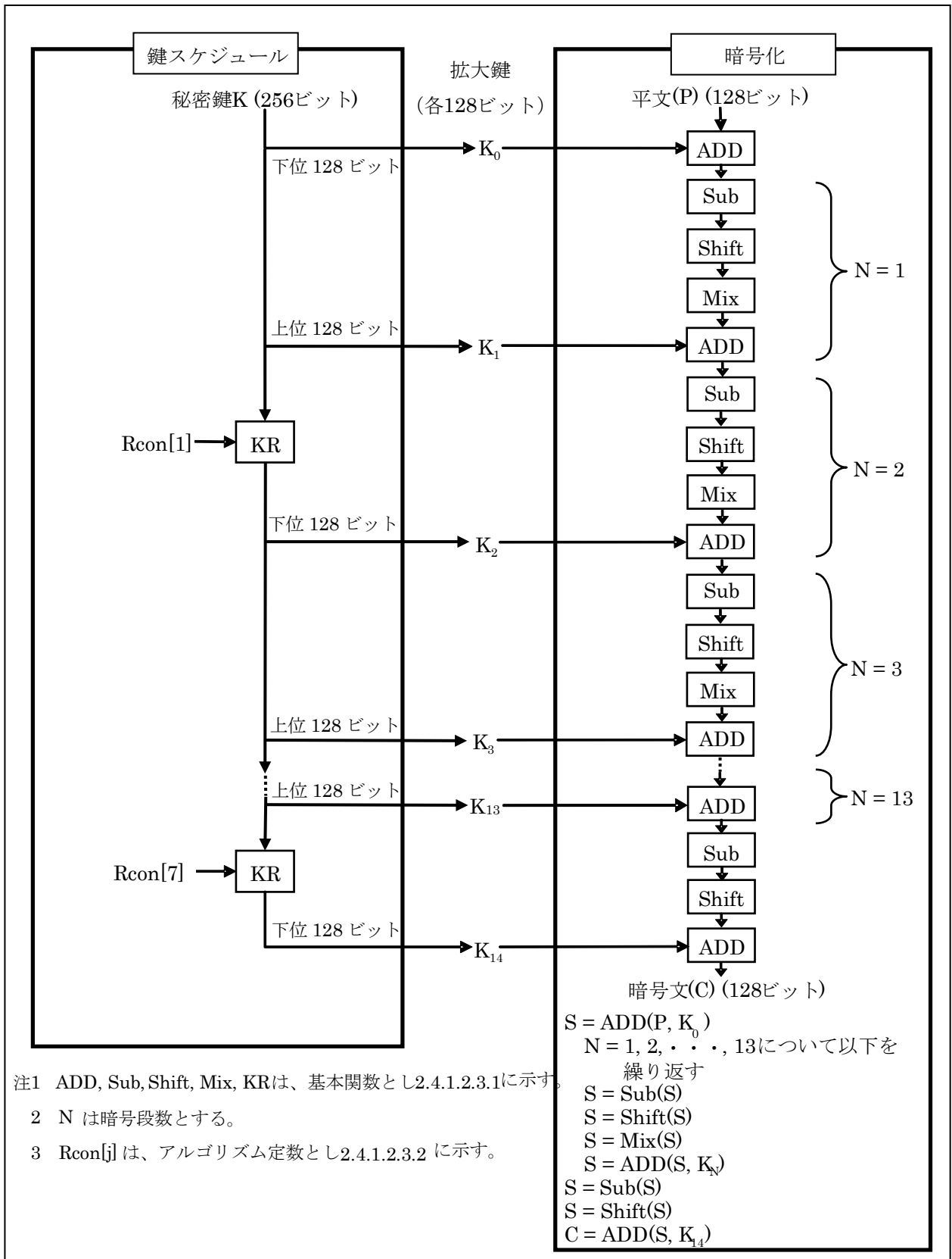
図 2.4.1.2.3-1 AES 暗号のアルゴリズム (鍵長 256 ビットの場合)
