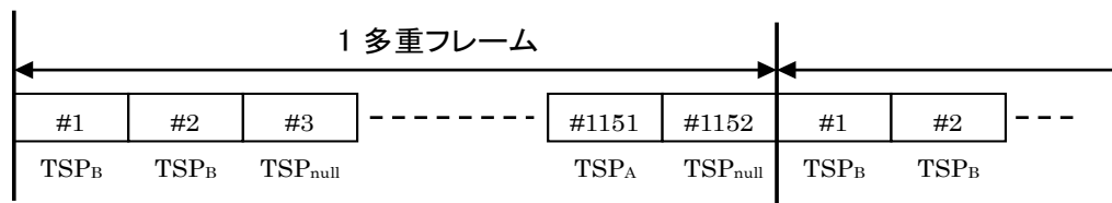
図 2.2.2.2.1-1 再多重されたトランスポートストリームの例 （モード 1、ガードインターバル 1/8 の場合）
