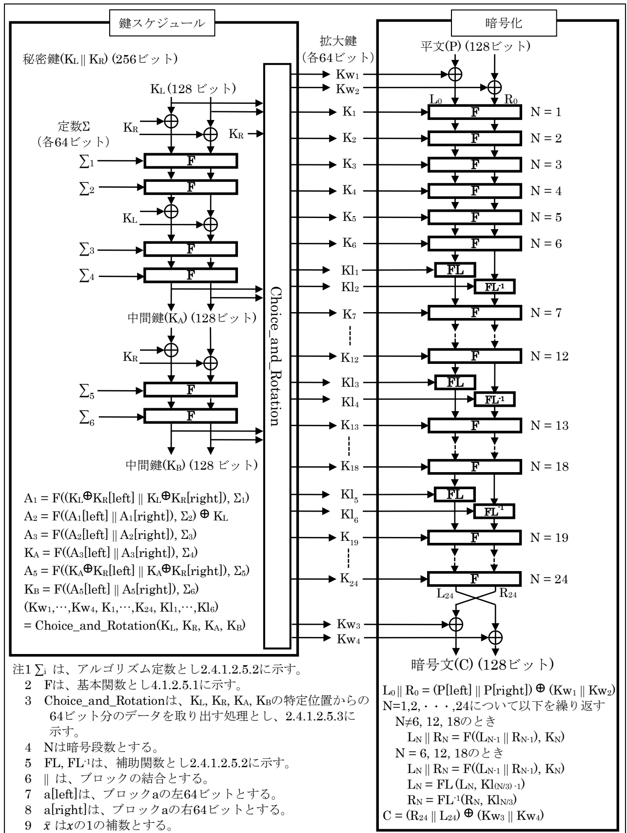
図 2.4.1.2.6-1 Camellia 暗号のアルゴリズム (鍵長 256 ビットの場合)
