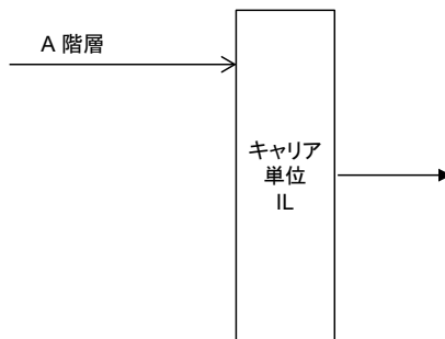
図 2. 2. 1. 6. 2. 9. 3-2 階層間インターリーブの入力が 1 階層
