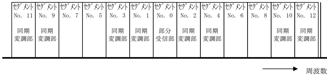
図 2.2.2.8-1 伝送スペクトル上の OFDM セグメント番号と使用例
