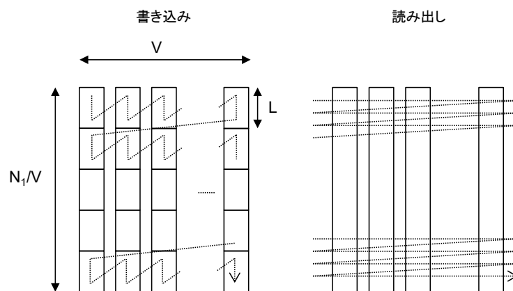
図 2.2.1.6.1.5.2-1 ブロックインターリーブ
