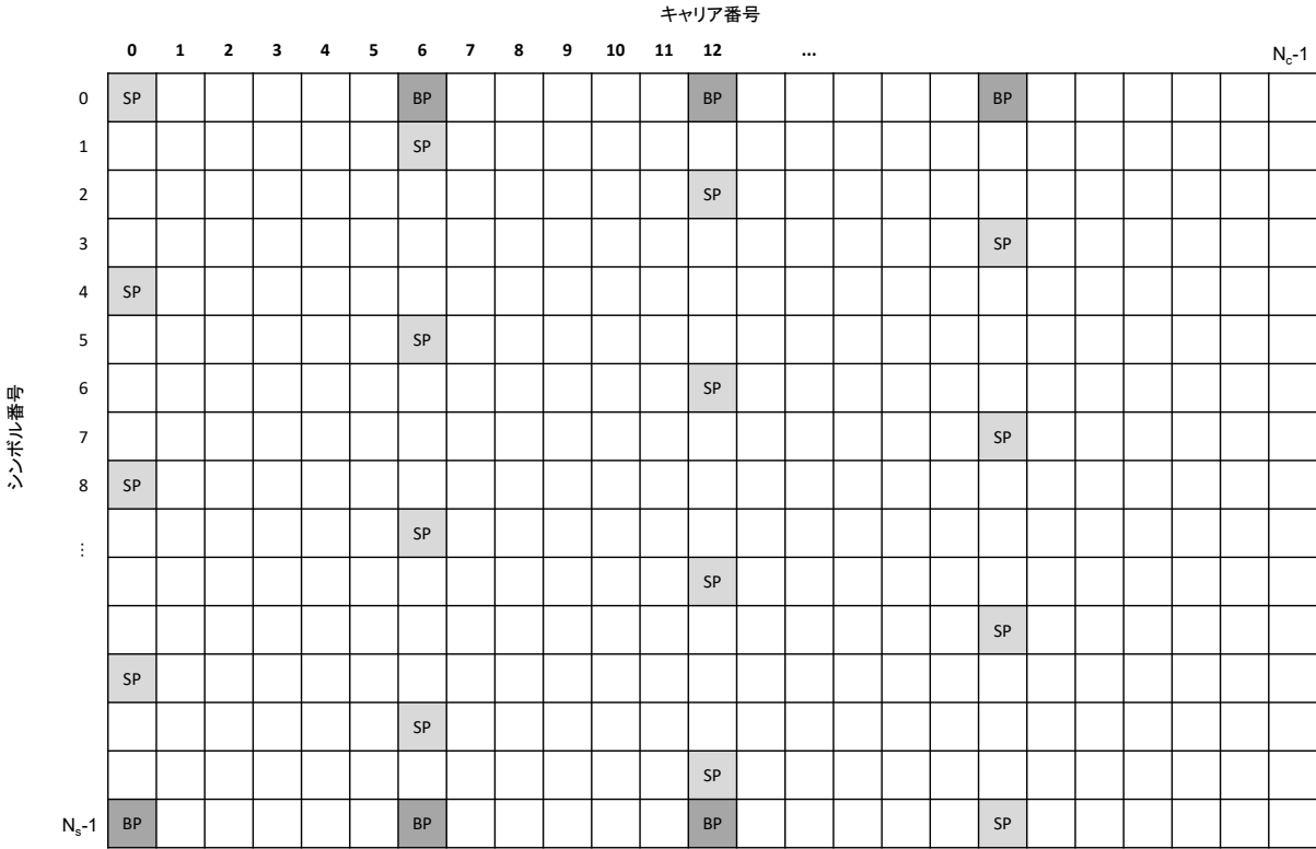
図 2.2.1.6.3.3.4-1 BP 配置の例 ( D_x=6 , D_y=4 )
