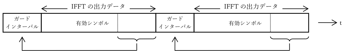
図 2.2.2.8.2-1 ガードインターバルの付加
