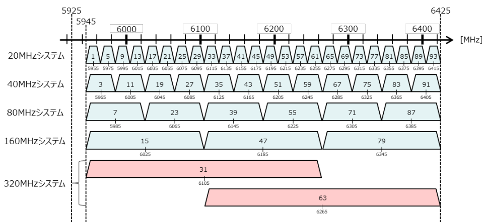
図 2.3-1 新たな 320MHz 幅チャネルの配置
