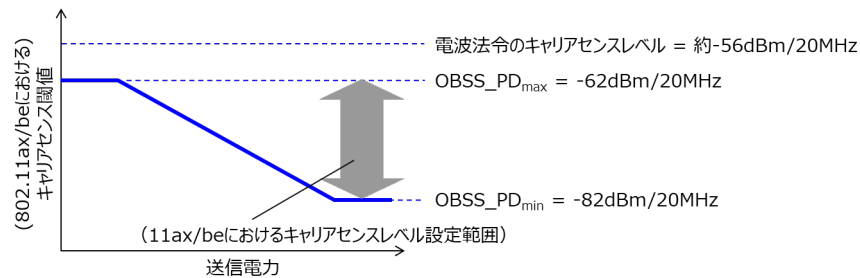
図 2.3-2 IEEE 802.11ax/be におけるキャリアセンスレベルの閾値
