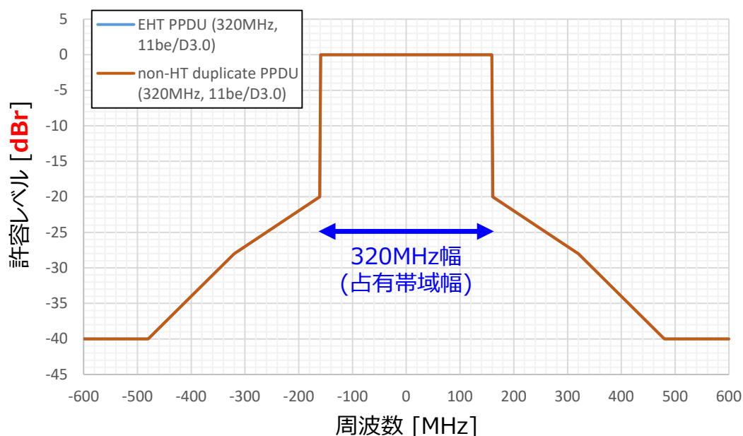
(a) IEEE 802.11be における 2 種類の 320MHz 幅チャネルのスペクトルマスク
