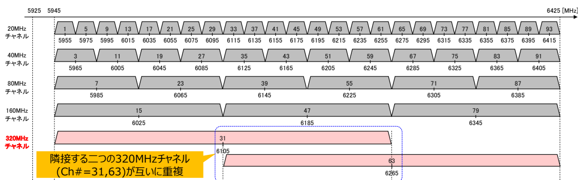
図 2. 5-1 6GHz 帯無線 LAN システムの 320MHz 幅チャネルの配置
