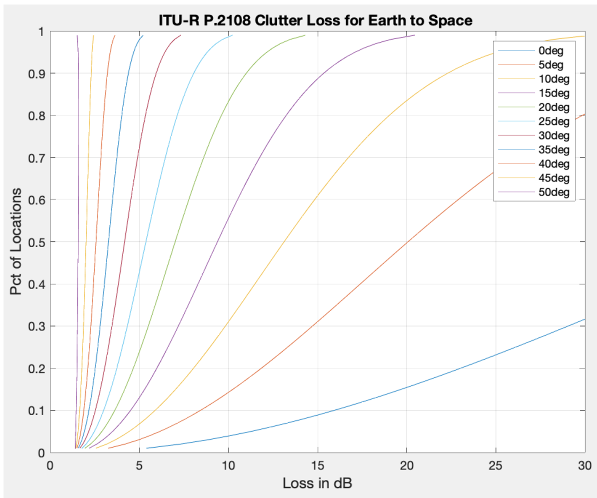
図 4.4-4 ITU-R 勧告 P. 2108 によるクラッタ損失
