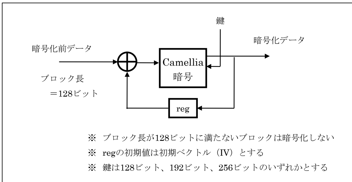
図 2.4.1.3.4-1 Camellia を用いたスクランブル手順 (CBC モード)
