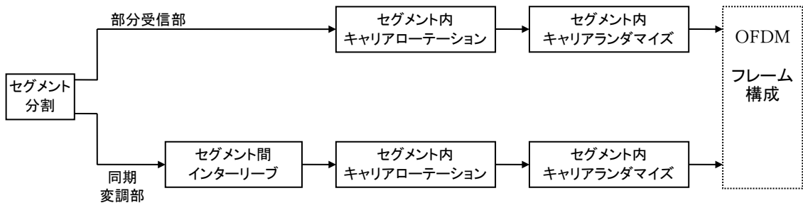
図 2.2.2.3.10-1 周波数インターリーブの構成
