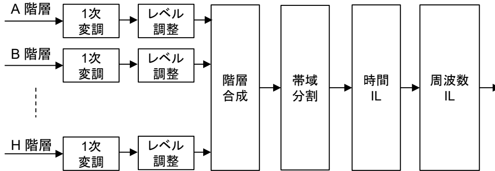
図 2.2.1.6.2.1-1 OFDM データセグメントの構成
