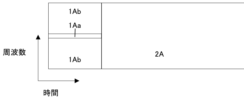
(e) 2サブ階層サブフレームと1階層サブフレームの例
