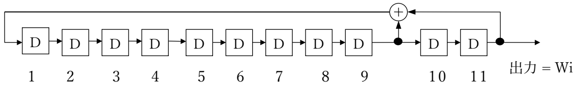
図 2.2.2.7.1-1 PRBS の生成回路
