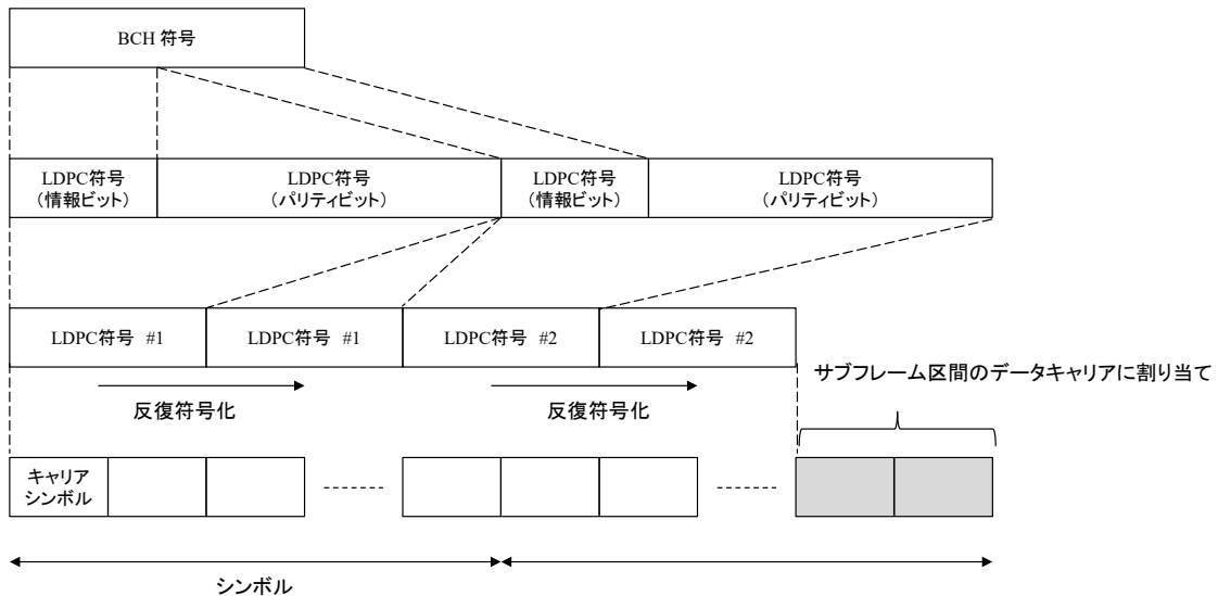
図 2.2.1.5.5.3-1 反復符号化
