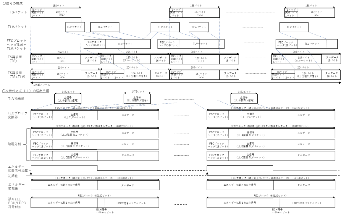
図 2. 2. 4-1 伝送主信号の構成及び送出手順 (LDM 放送時の LL)
