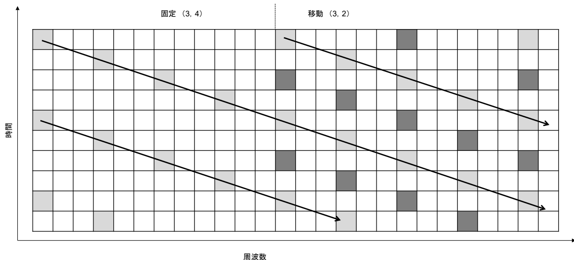
図 2.2.1.6.3.3.3-1 SP 配置の例
