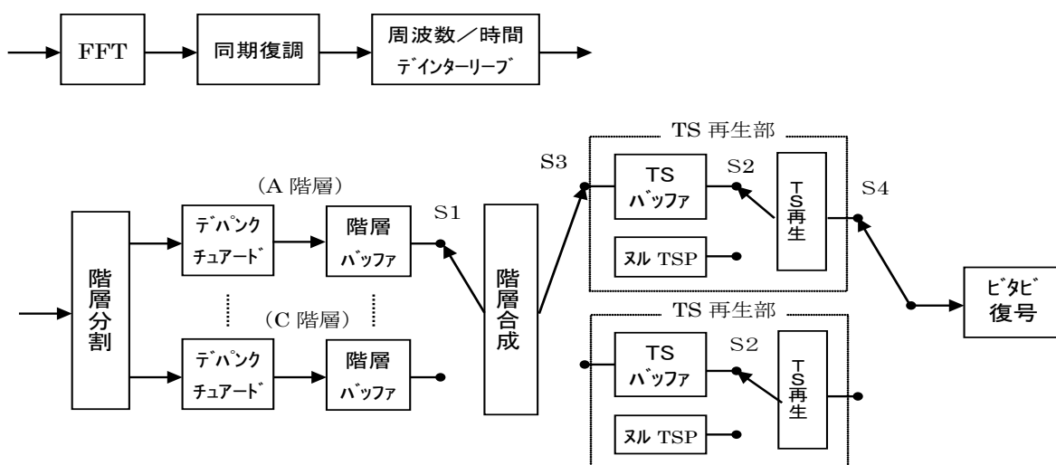
図 2.2.2.2.1-2 多重フレームパターン構成用モデル受信機
