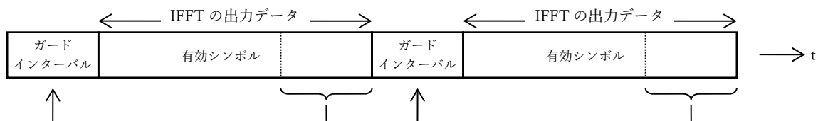
図 2.2.2.8.2-1 ガードインターバルの付加
