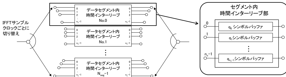
図 2.2.1.6.2.8.1-1 時間インターリーブ
