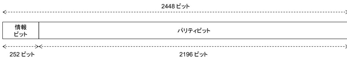
(b) 符号 2 (2448, 252)
