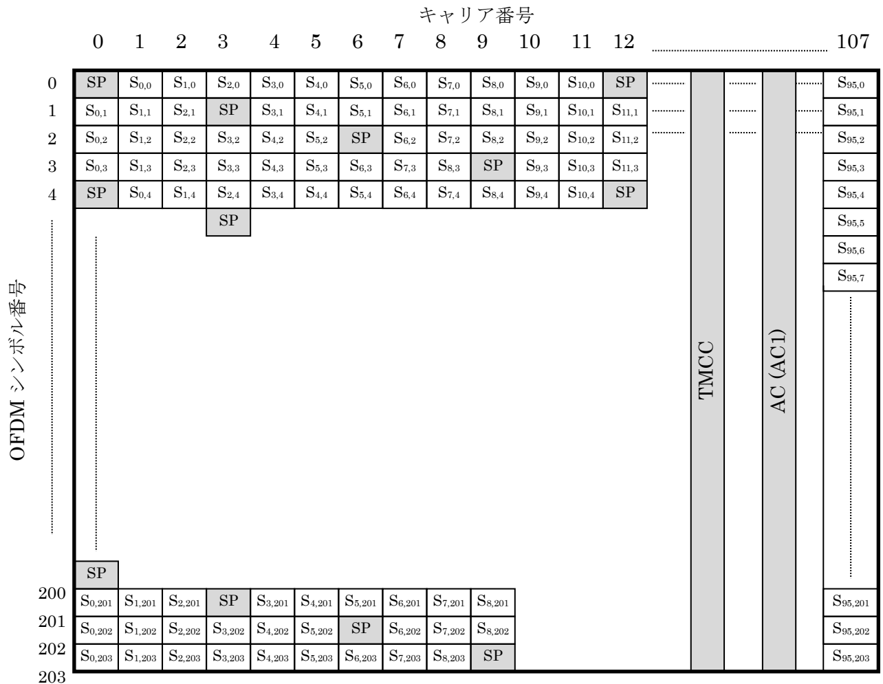
図 2.2.2.6-1 同期変調部の OFDM セグメント構成
