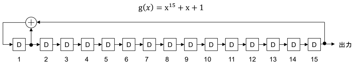
図 2. 2. 1. 6. 3. 3-2 キャリア PRBS 生成回路
