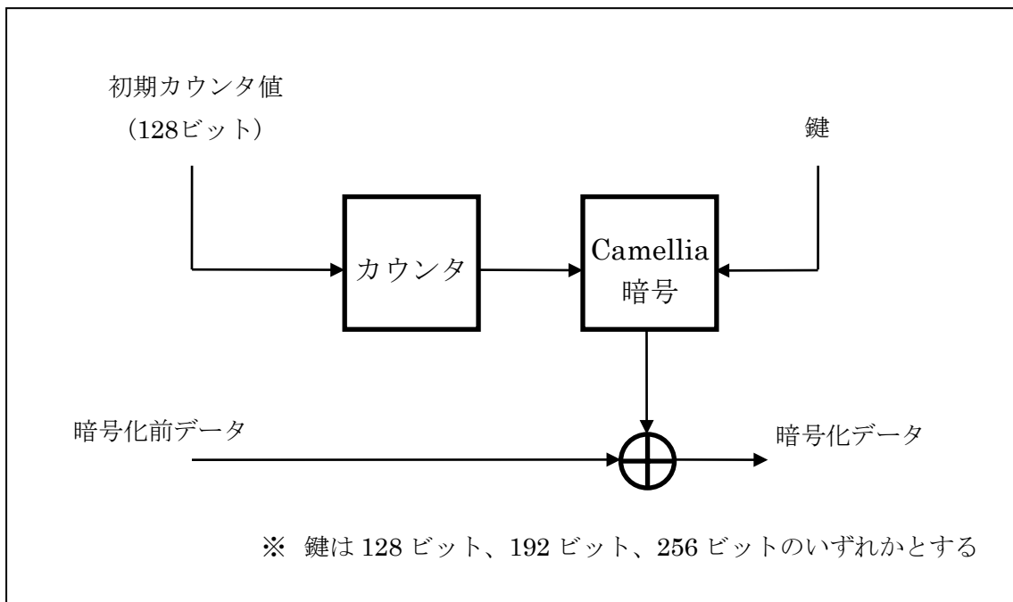
図 2.4.1.3.3-1 Camellia を用いたスクランブル手順 (CTR モード)
