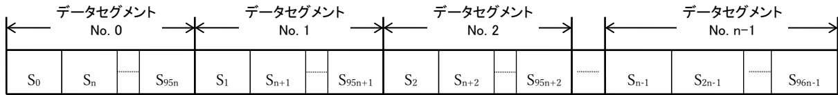
(a) モード1のセグメント間インターリーブ
