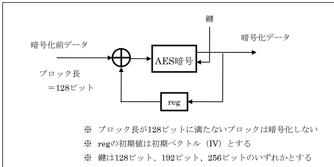
図 2.4.1.3.2-1 AES を用いたスクランブル手順 (CBCモード)
