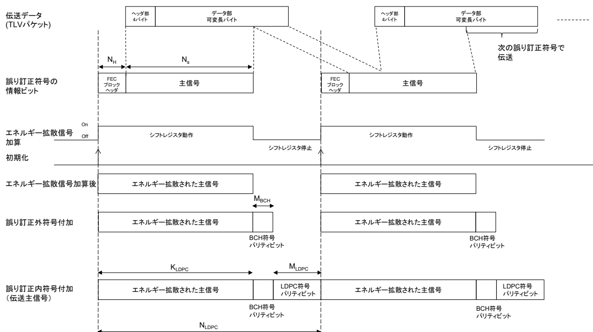
図 2.2.1.6.1-1 伝送主信号の構成
