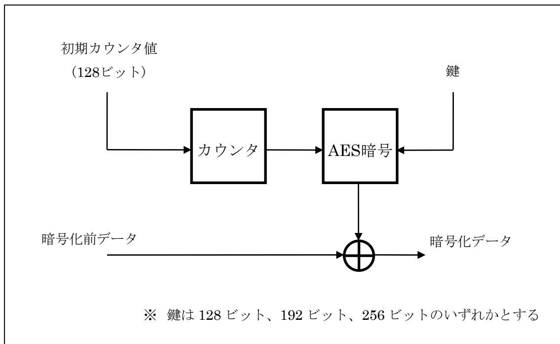
図 2.4.1.3.1-1 AES を用いたスクランブル手順 (CTRモード)
