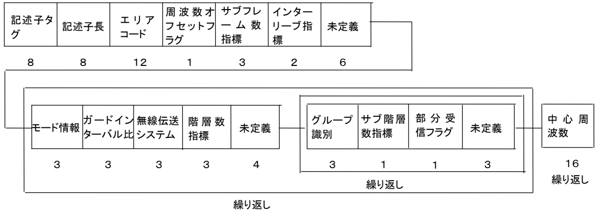
図 2.3.3-1 第2世代地上配信システム記述子の構成
