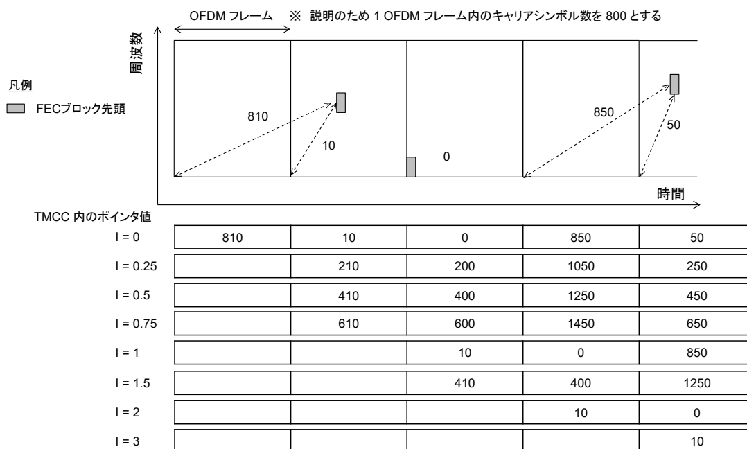
図 2.1.6.1.2.4-1 FEC ブロックポインタの遅延の例
