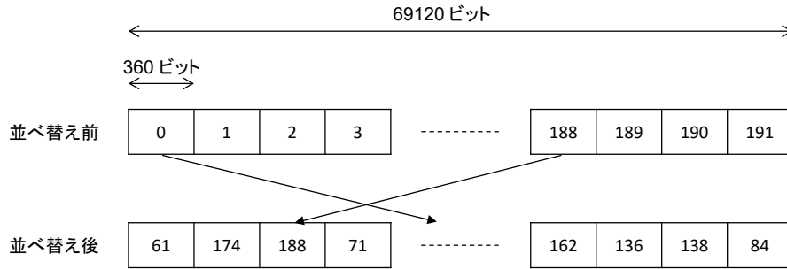
図 2. 2. 1. 6. 1. 5. 1-1 グループワイズインターリーブ (QPSK, 符号化率 2/16 の例)
