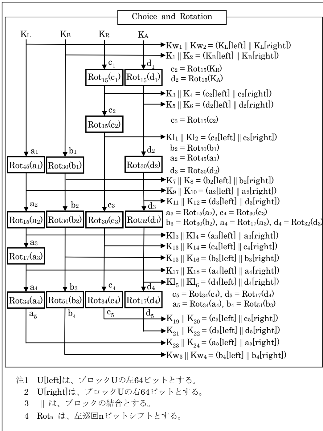
図 2.4.1.2.5.3-1 Camellia 暗号の Choice_and_Rotation
