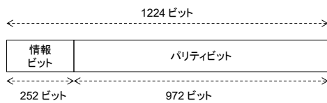
(a) 符号 1 (1224, 252)
