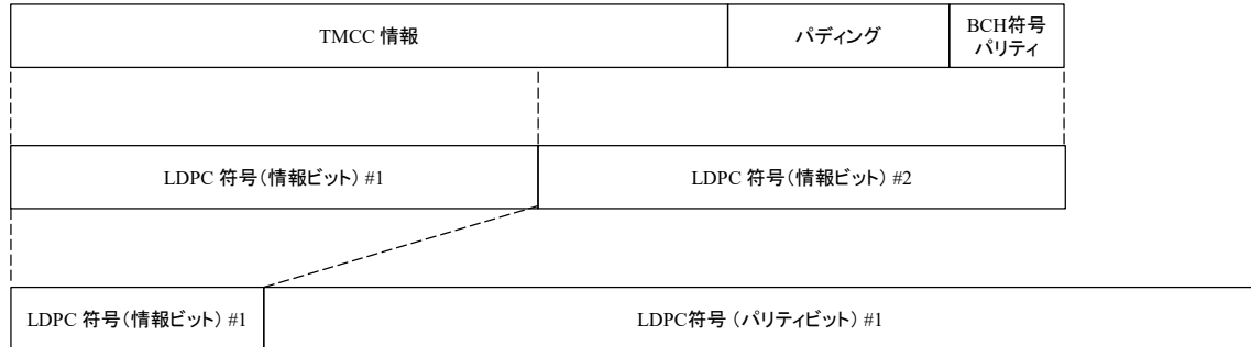
図 2.2.1.5.2-1 伝送制御情報の誤り訂正符号化
