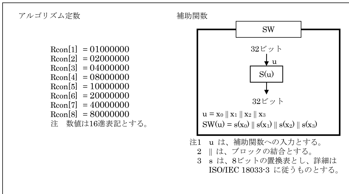
図 2. 4. 1. 2. 2. 2-1 AES 暗号のアルゴリズム定数と補助関数 (鍵長 192 ビットの場合)
