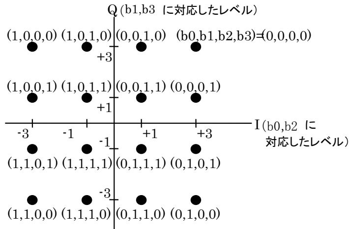
図2. 2. 2. 3. 7. 3. 2-2 16QAMの位相図
