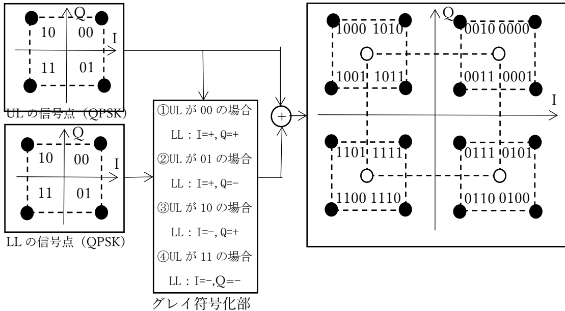
図 2.2.2.4.12-1 変調器のグレイ符号化処理フロー
