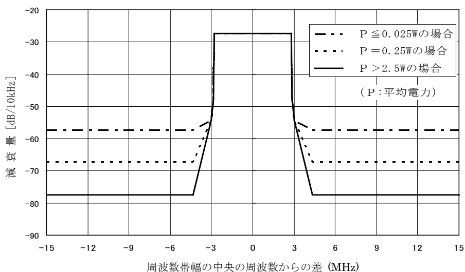
図 2.1.2.5-1 LDM 放送、次世代放送の送信スペクトルマスク
