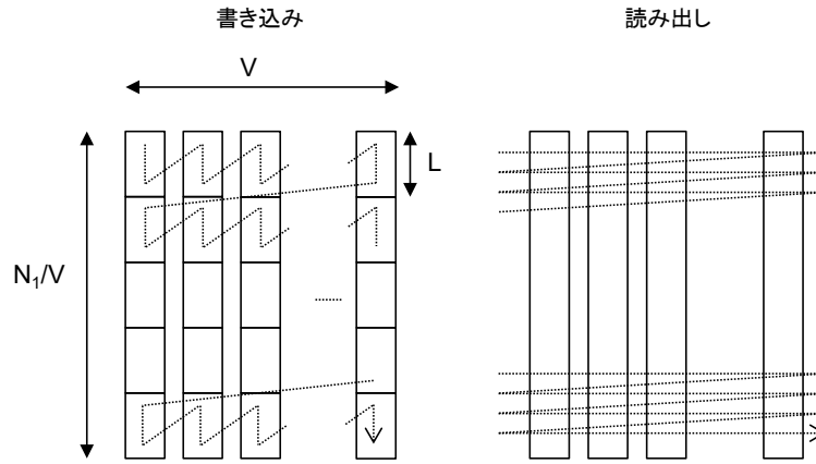
図 2.2.2.4.7.2-1 ブロックインターリーブ
