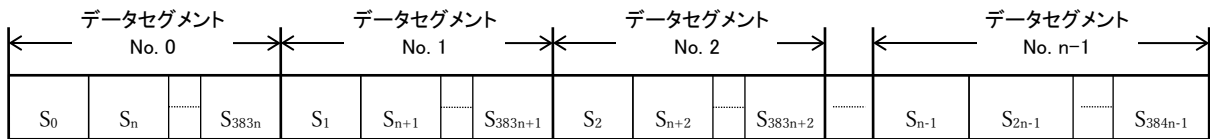
(c) モード3のセグメント間インターリーブ
