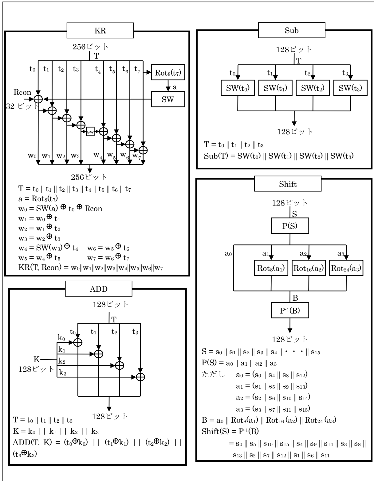
図 2.4.1.2.3.1-1 AES 暗号の基本関数 (鍵長 256 ビットの場合)
