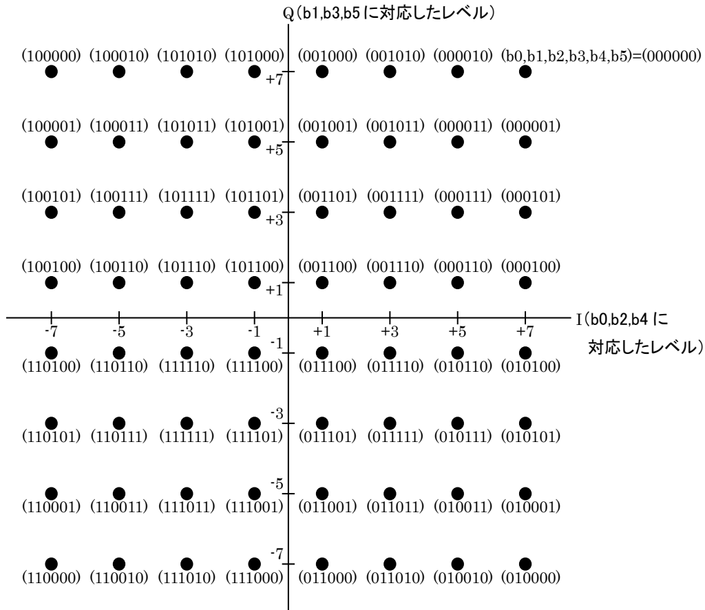
図2.2.2.3.7.3.3-2 64QAM の位相図
