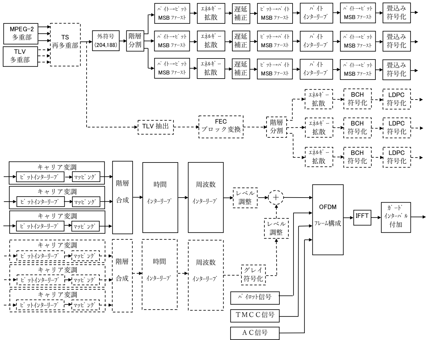
図 2.2.2.1-1 LDM 放送の伝送路符号化部系統 (点線部分が次世代方式 (LL) で追加される)
