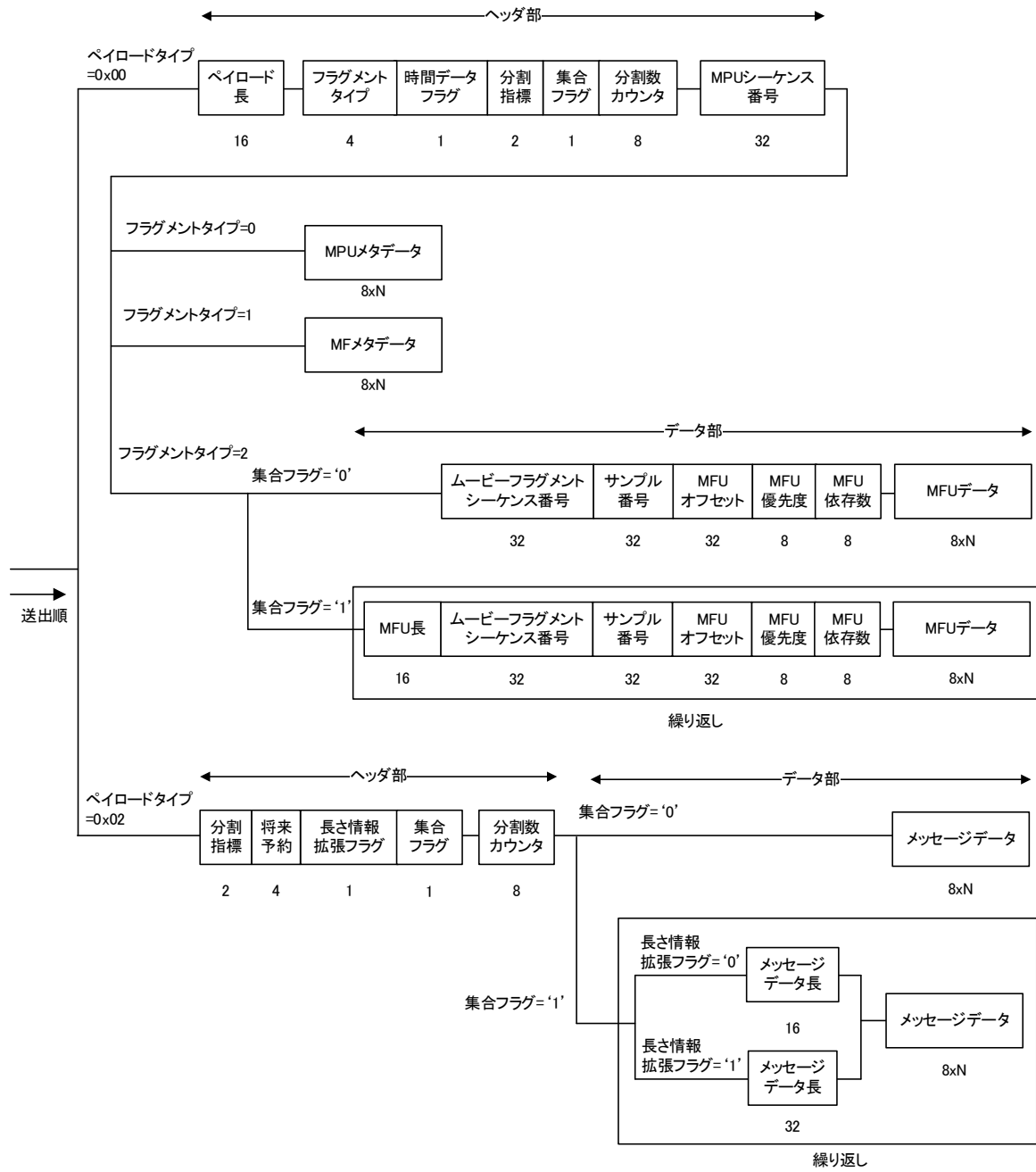
図 2.3.2-1 MMTP ペイロードの構成
