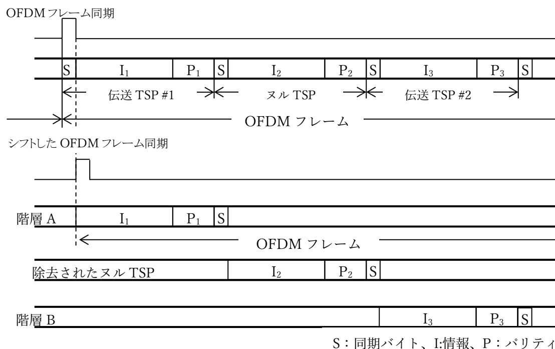
図 2.2.2.3.2-1 階層分割部の動作例
