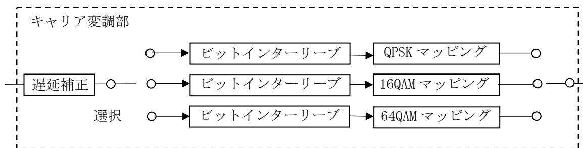
図2.2.2.3.7.1-1 キャリア変調部の構成
