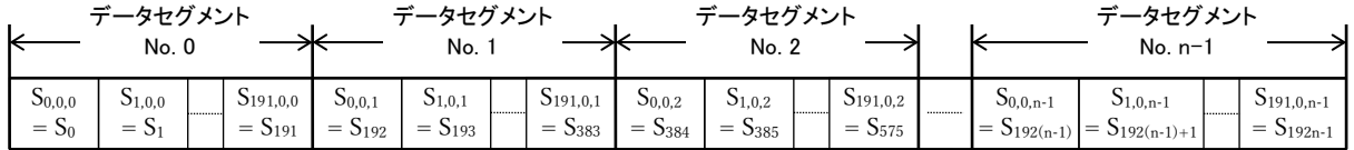
(a) モード1のセグメント間インターリーブ
