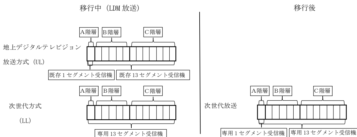
図 2.2.2-1 高度化放送導入方式の階層伝送及び部分受信
