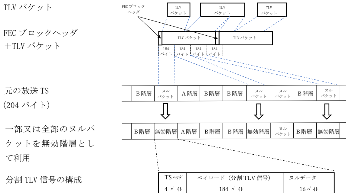
図 2.2.2.2.1-3 放送 TS への TLV 信号重畳法
