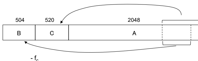
図 2.2.1.4.4.2-1 BCA 構造
