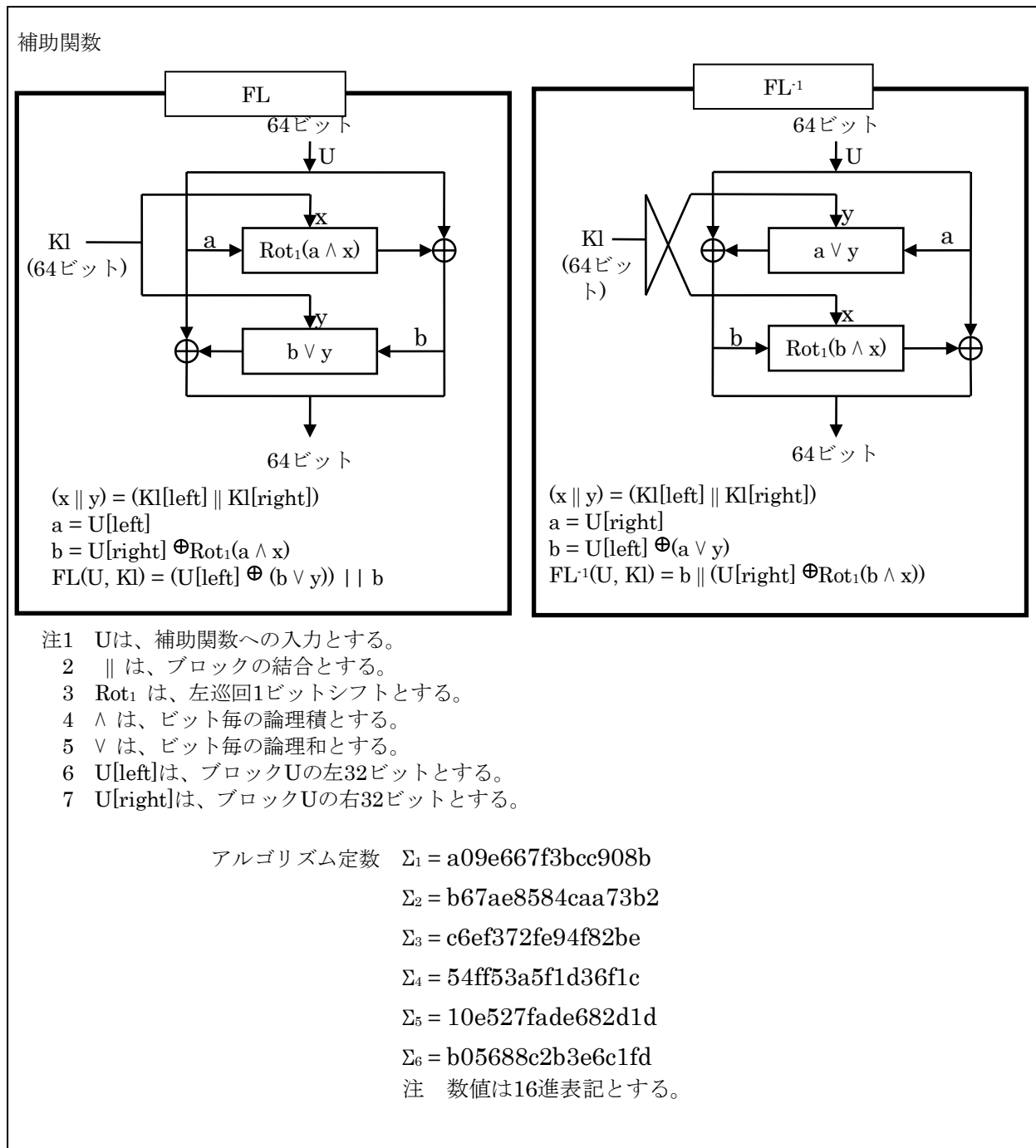
図 2.4.1.2.5.2-1 Camellia 暗号の補助関数とアルゴリズム定数
