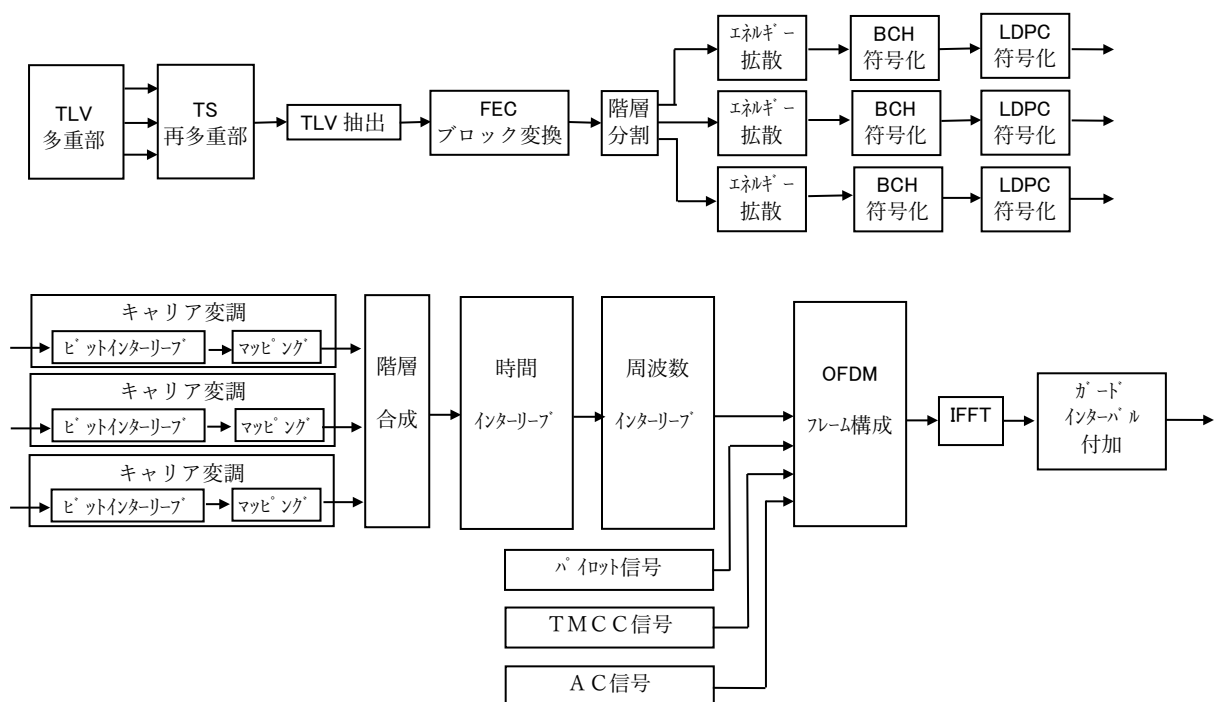
図 2.2.2.1-2 次世代放送の伝送路符号化部系統
