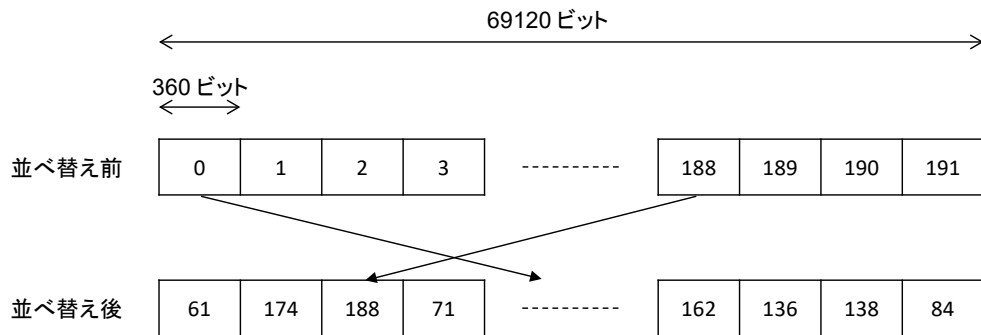
図 2.2.2.4.7.1-1 グループワイズインターリーブ (QPSK, 符号化率 2/16 の例)
