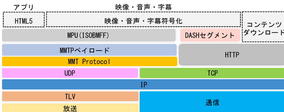
図 2.3.1-1 MMT・TLV方式のレイヤモデル
