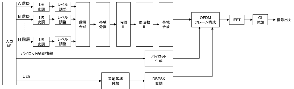
図 2.2.1.2.1-1 OFDM 変調部の構成
