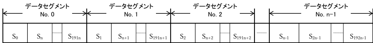
(b) モード2のセグメント間インターリーブ
