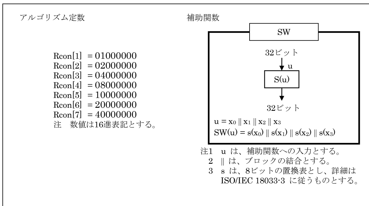
図 2. 4. 1. 2. 3. 2-1 AES 暗号のアルゴリズム定数と補助関数 (鍵長 256 ビットの場合)
