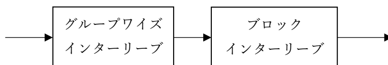
図 2.2.2.4.7-1 ビットインターリーブの構造
