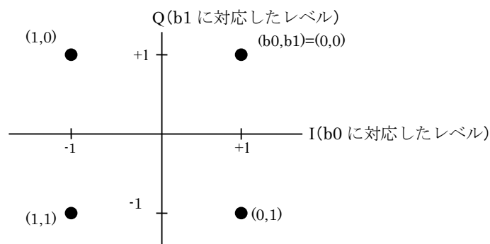
図2.2.2.3.7.3.1-2 QPSK位相図
