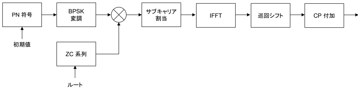
図 2.2.1.4.1-1 フレーム同期信号生成部の構成
