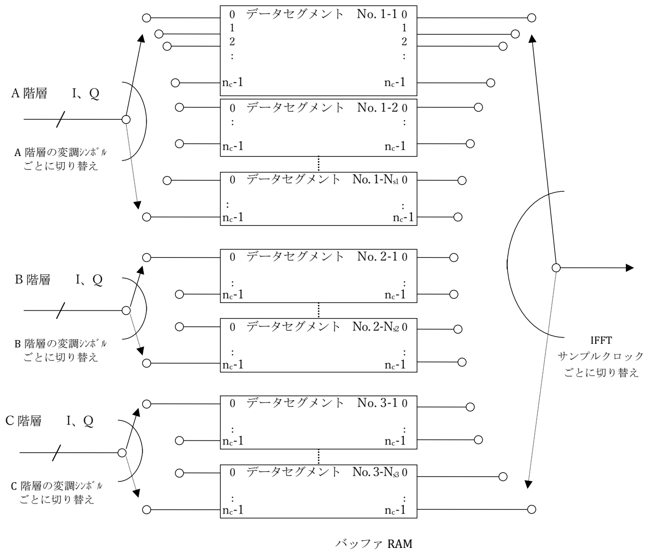
図2.2.2.3.8-1 階層合成の構成
