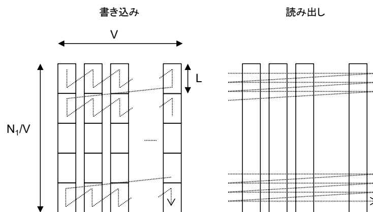
図 2.2.1.6.1.5.2-1 ブロックインターリーブ
