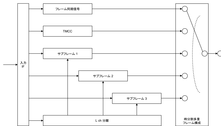
図 2.2.1.2-2 地上放送高度化方式のフレーム構成部 (サブフレームが3つの場合)
