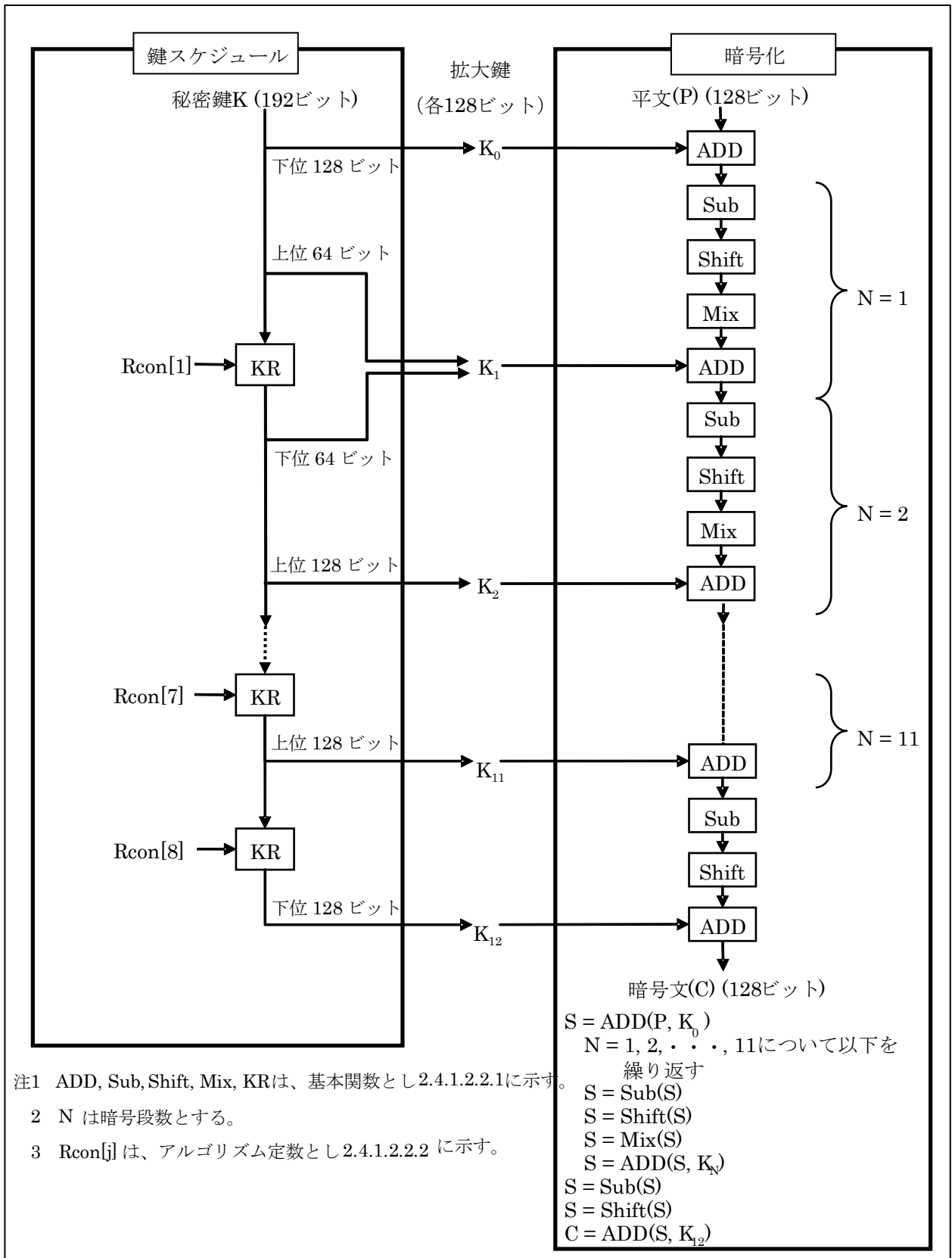
図 2.4.1.2.2-1 AES 暗号のアルゴリズム (鍵長 192 ビットの場合)
