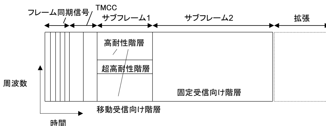
図 2.2.1.1.2-1 地上放送高度化方式のフレーム構成例
