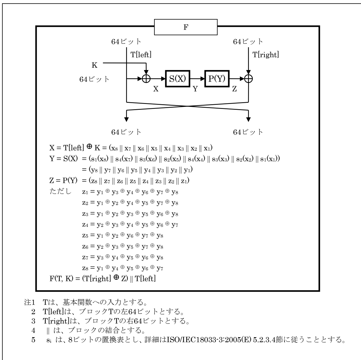
図 2.4.1.2.5.1-1 Camellia 暗号の基本関数
