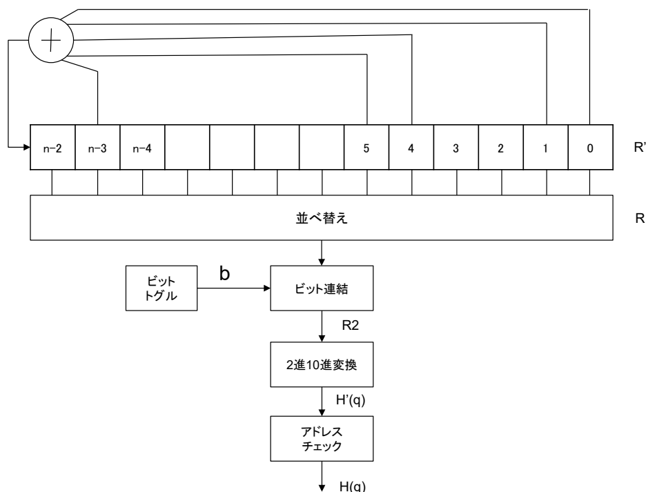
図 2.2.1.6.2.9.4.2-1 アドレス生成回路
