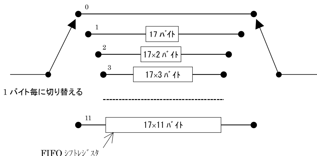
図 2.2.2.3.5-1 バイトインターリーブ
