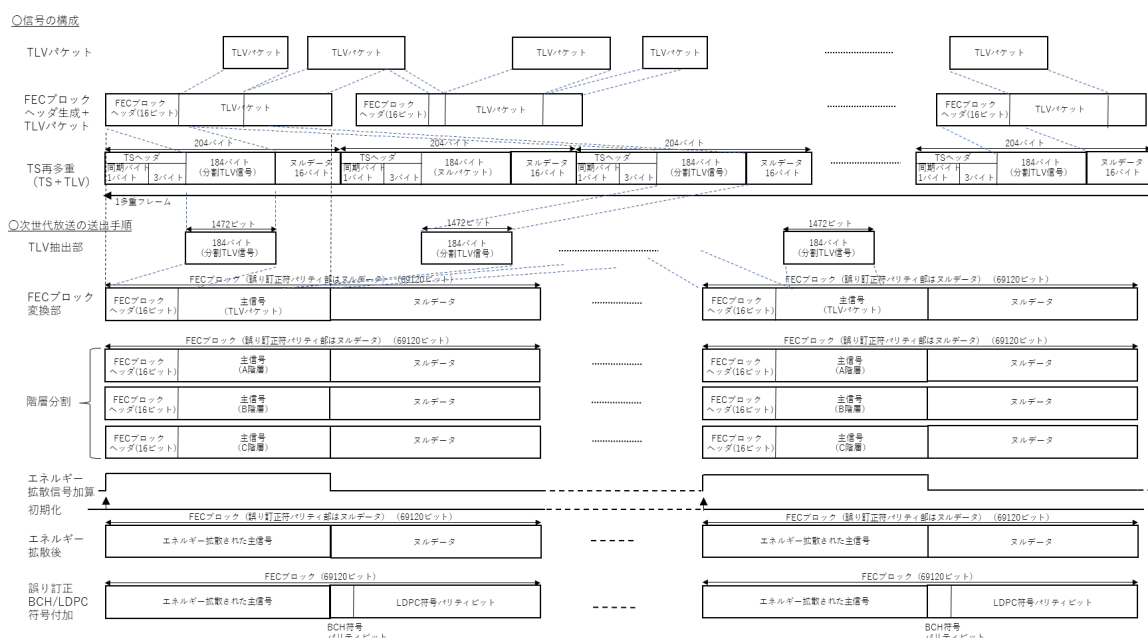
図 2.2.2.4-2 伝送主信号の構成及び送出手順 (次世代放送時)
