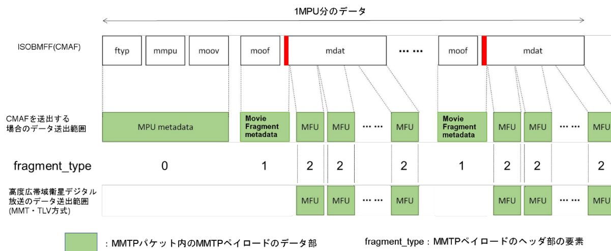
図 2. 3. 2-2 4K8K 衛星放送 (MMT・TLV 方式) と CMAF を送出する場合のデータ送出範囲の違い
