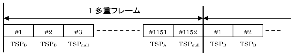
図 2.2.2.2.1-1 再多重されたトランスポートストリームの場合 (モード 1、ガードインターバル 1/8 の場合)
