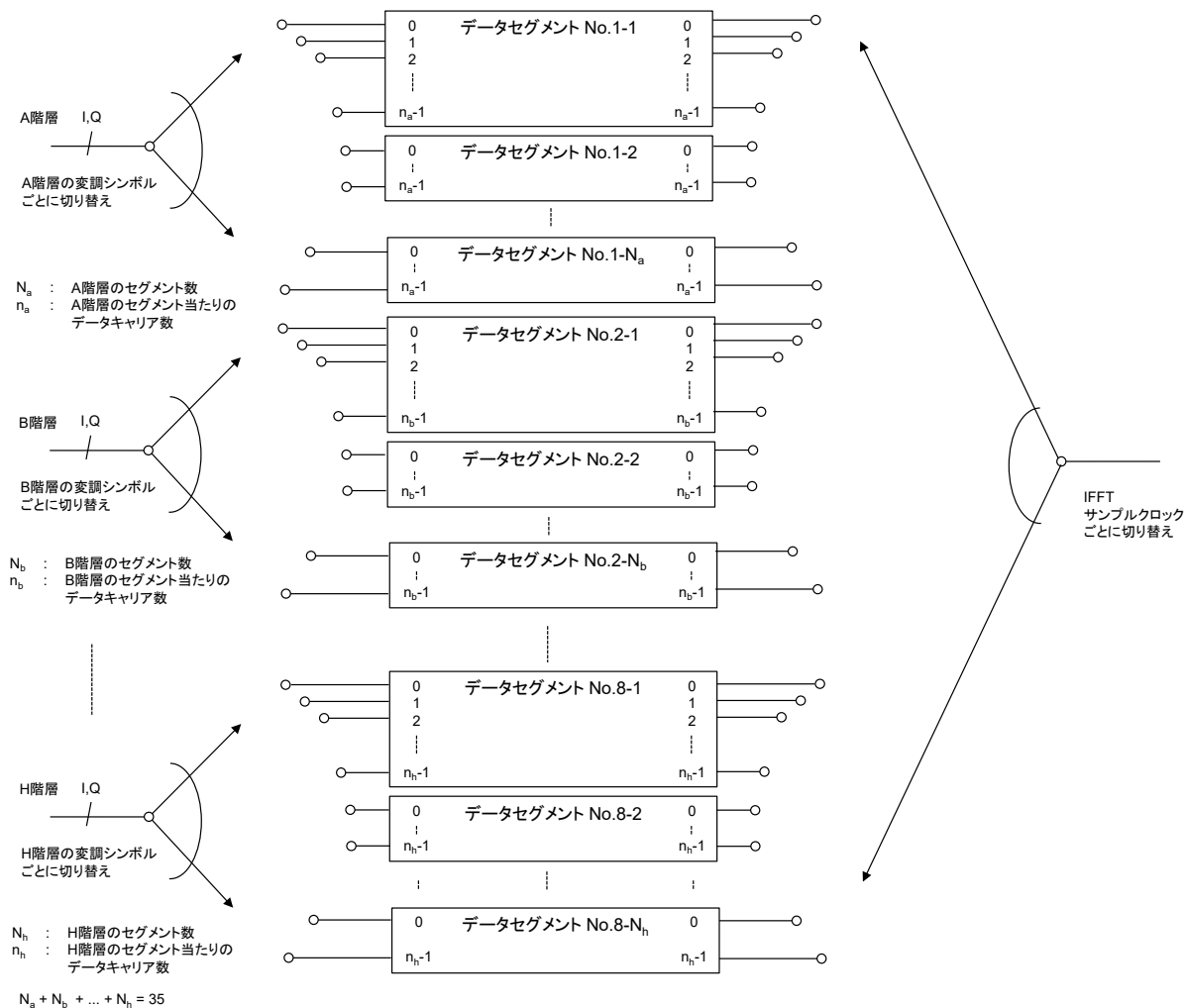
図 2.2.1.6.2.6-1 階層合成の信号処理手順
