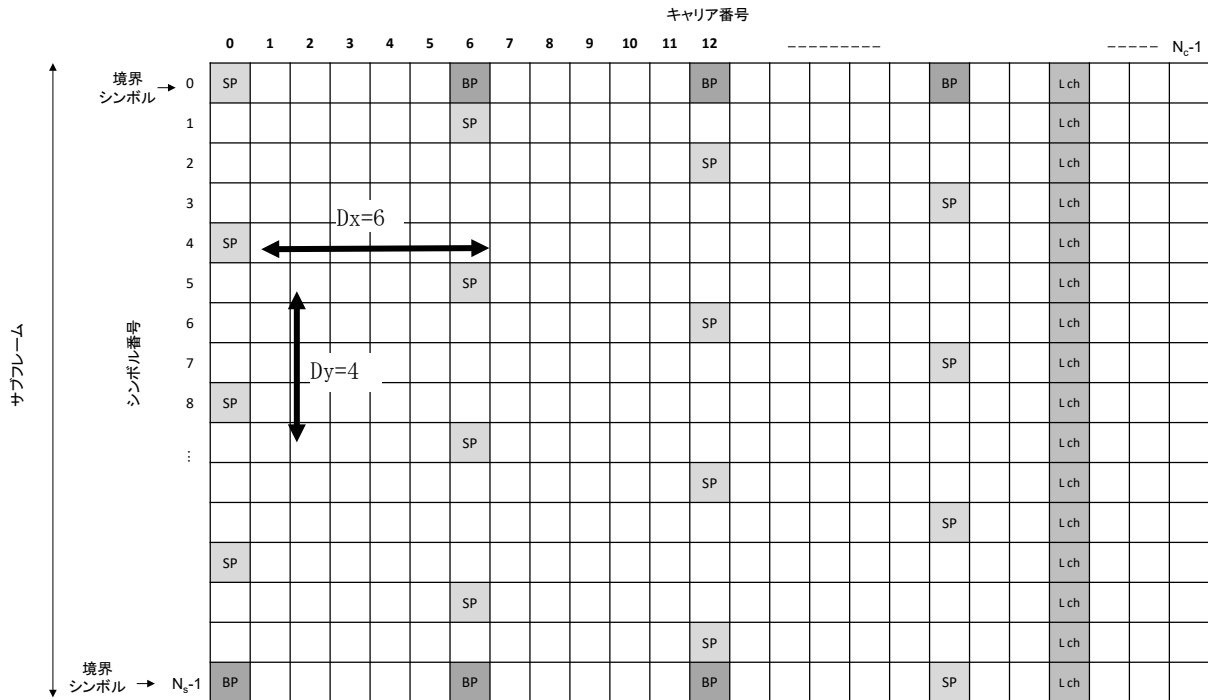
図 2. 2. 1. 6. 3. 2-1 サブフレーム区間の OFDM セグメント構成
