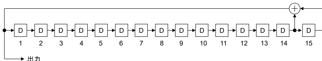
図 2.2.1.6.1.3-1 PRBS 生成回路
