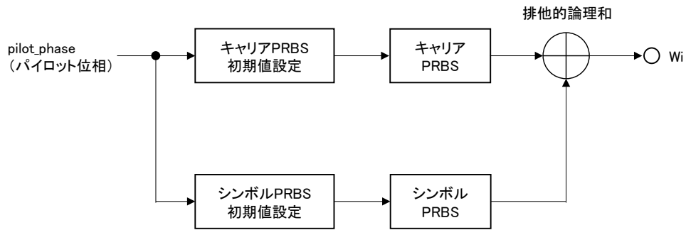
図 2. 2. 1. 6. 3. 3-1 Wi 生成回路
