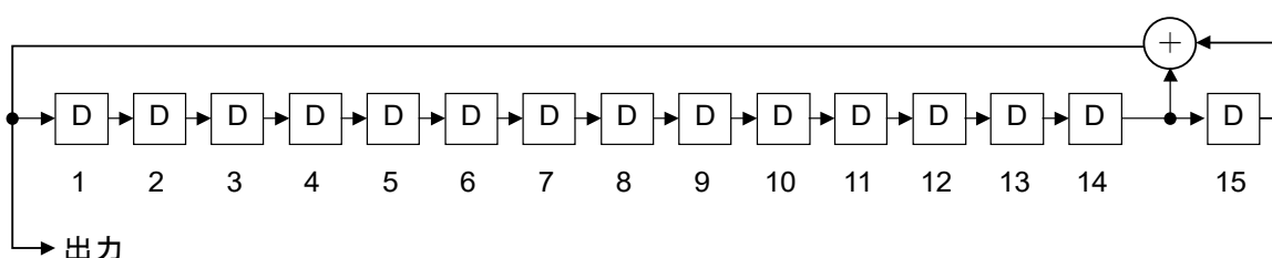
図2.2.2.3.3-1 PRBSの生成多項式と回路
