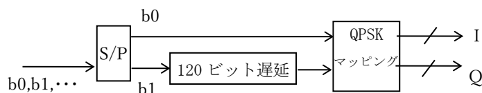
図2.2.2.3.7.3.1-1 QPSK変調系統図
