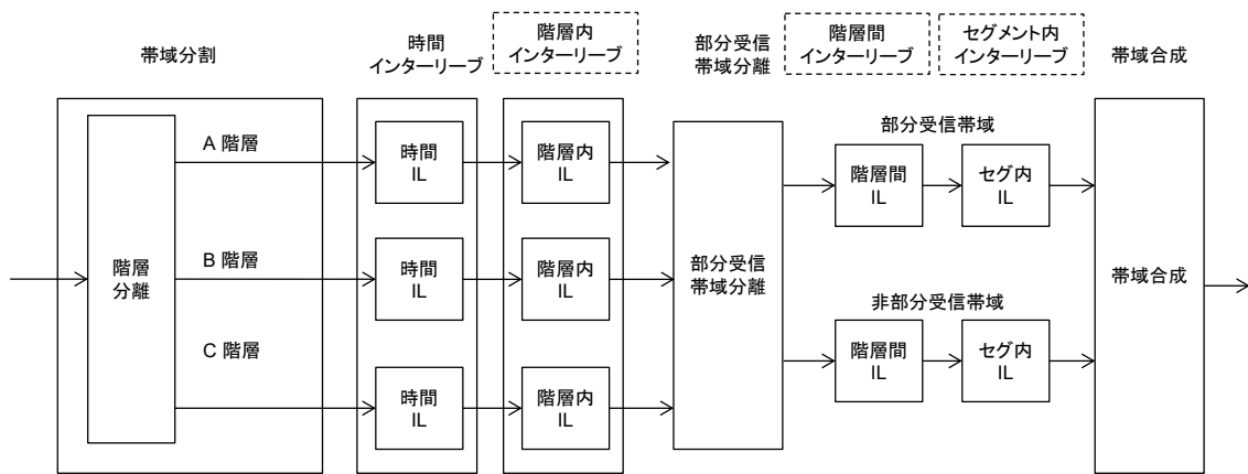
図 2.2.1.6.2.9-1 周波数インターリーブ
