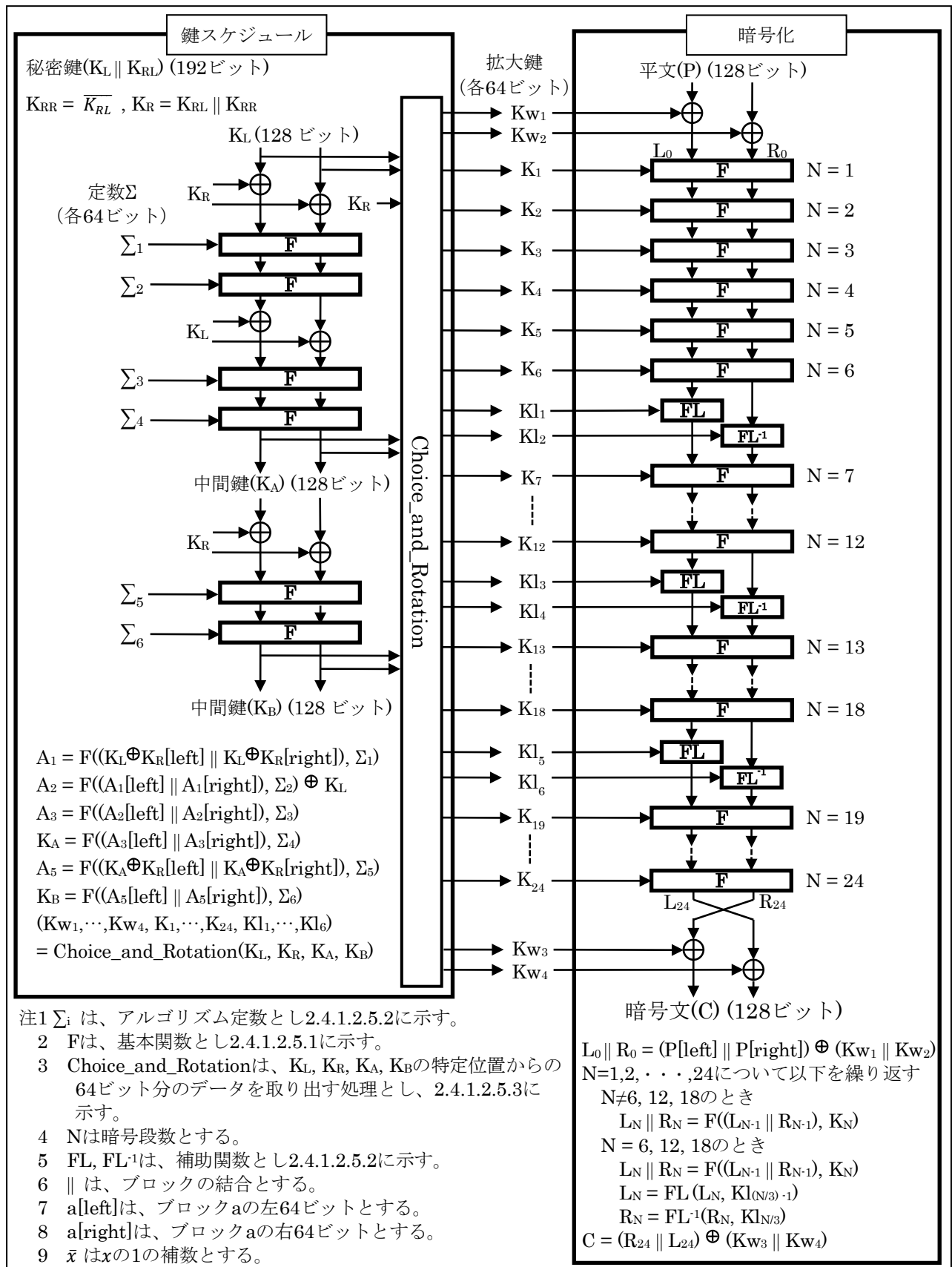
図 2.4.1.2.5-1 Camellia 暗号のアルゴリズム (鍵長 192 ビットの場合)
