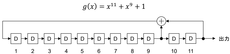
図 2. 2. 1. 6. 3. 3-3 シンボル PRBS 生成回路
