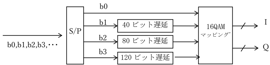
図2. 2. 2. 3. 7. 3. 2-1 16QAM変調系統図
