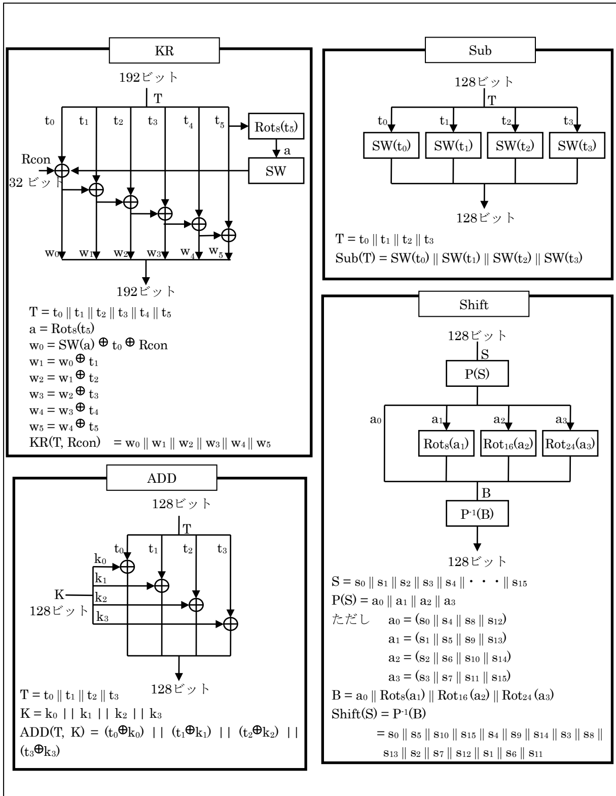
図 2.4.1.2.2.1-1 AES 暗号の基本関数 (鍵長 192 ビットの場合)
