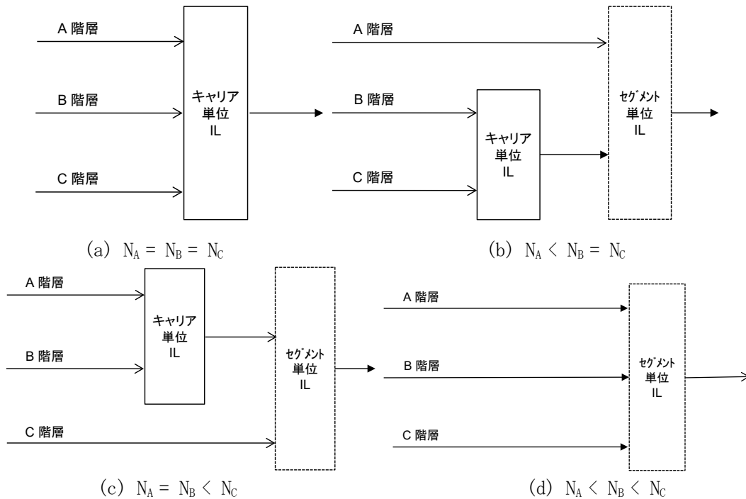
図 2.2.1.6.2.9.3-4 階層間インターリーブの入力が3階層
