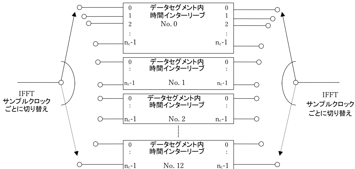
図 2.2.2.3.9-1 時間インターリーブの構成
