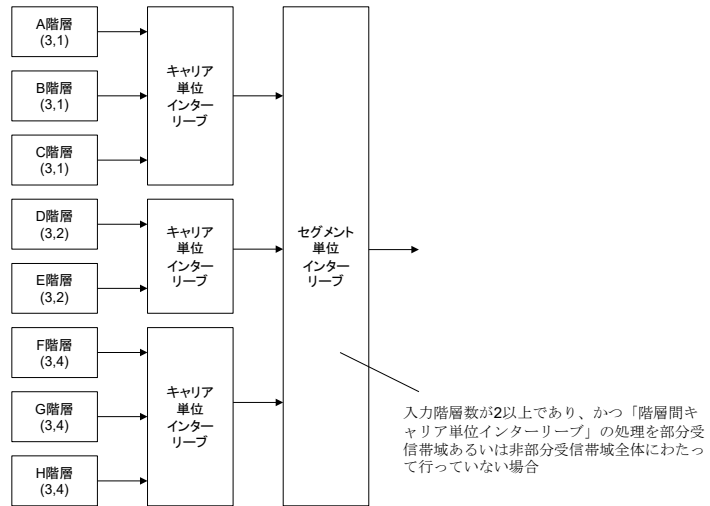
図 2. 2. 1. 6. 2. 9. 3-1 階層間インターリーブ
