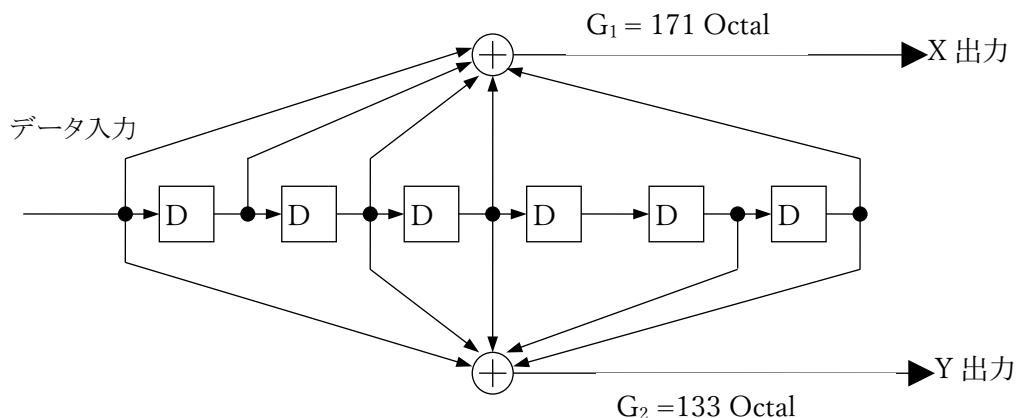
図2.2.2.3.6-1 拘束長k=7、符号化率1/2の畳込み符号の符号化回路
