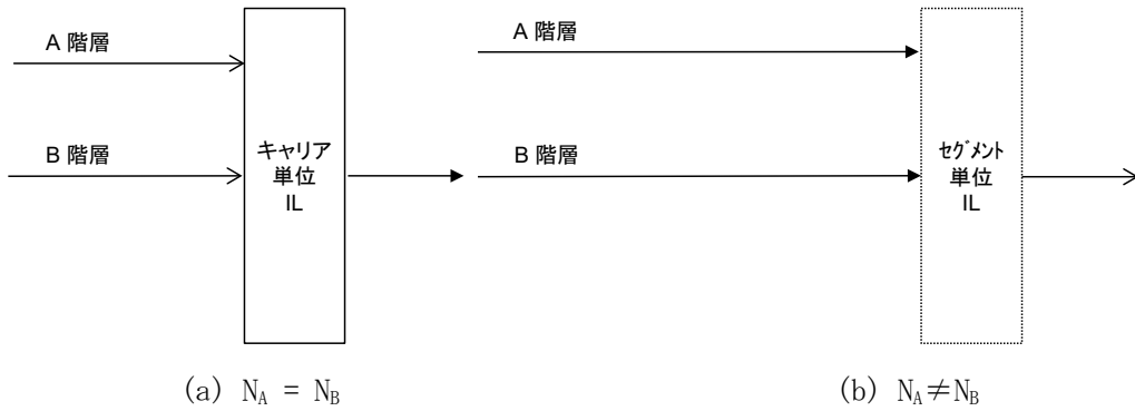
図 2. 2. 1. 6. 2. 9. 3-3 階層間インターリーブの入力が 2 階層
