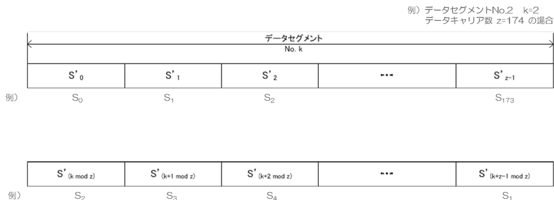
図 2.2.1.6.2.9.4.1-1 セグメント内キャリアローテーション
