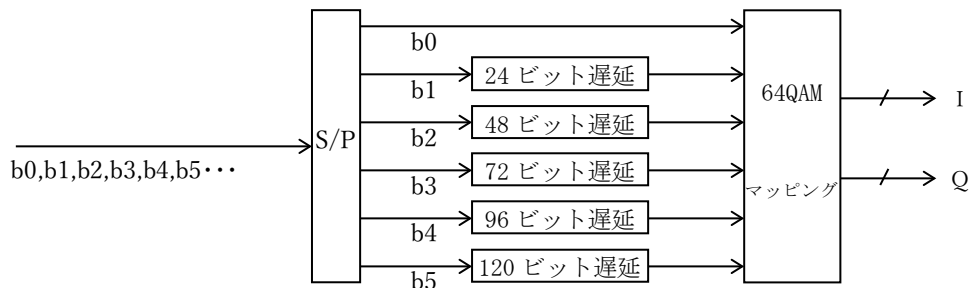
図2. 2. 2. 3. 7. 3. 3-1 64QAM変調系統図
