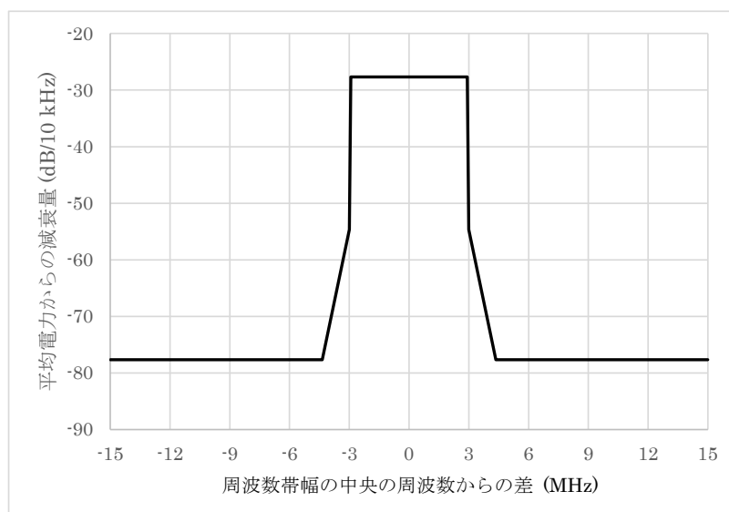
図 2.1.1.5-1 地上放送高度化方式の送信スペクトルマスク
