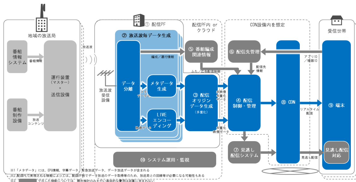
図2-5 B案の全体構成・アーキテクチャ
