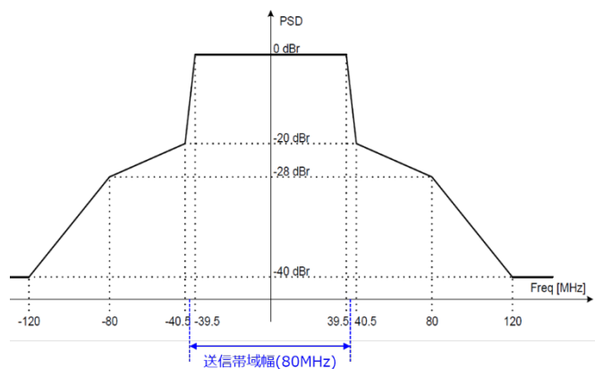
(a) puncturing ブロックがない場合の 80MHz 幅スペクトルマスク
