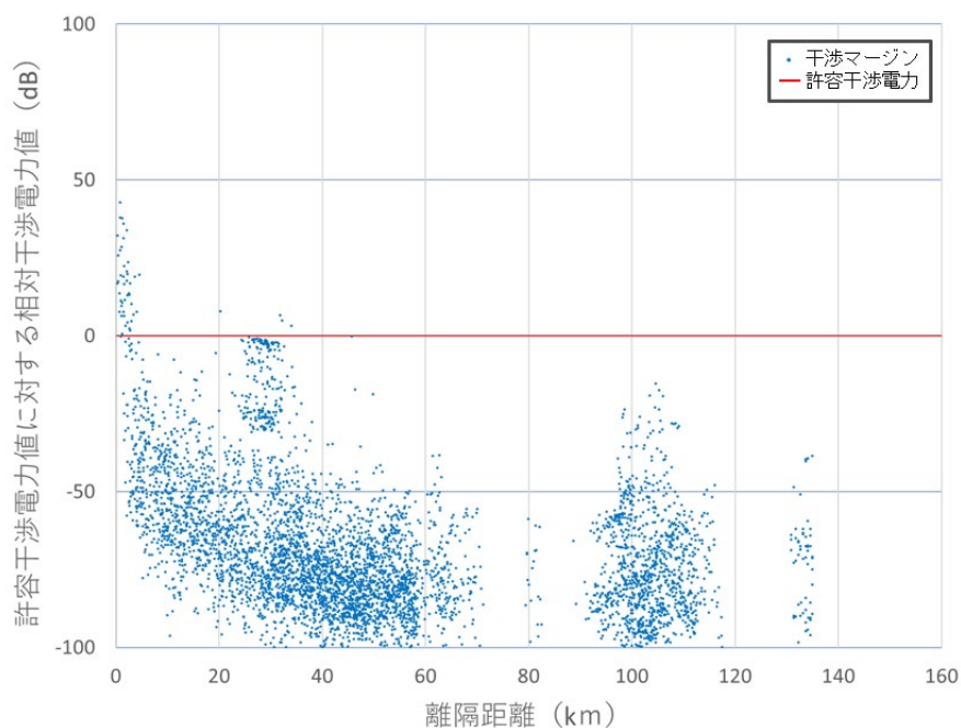
図 2. 3-2 5Gスモールセル基地局（最大パターン）から無線航行衛星システムの地球局（奄美大島・対静止衛星）への干渉影響
