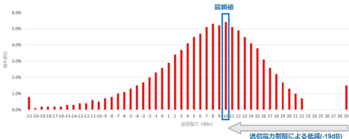
図2.3-6 検討に用いた陸上移動局(最大電力 29dBm)の電力分布
