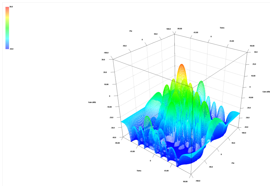
図参 1-5 手法 2 で用いたマクロセル基地局の空中線指向特性（瞬時パターン）
