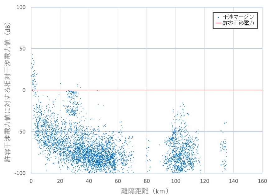
図 2. 3-3 5Gスモールセル基地局（最大パターン）から無線航行衛星システムの地球局（奄美大島・対非静止衛星）への干渉影響
