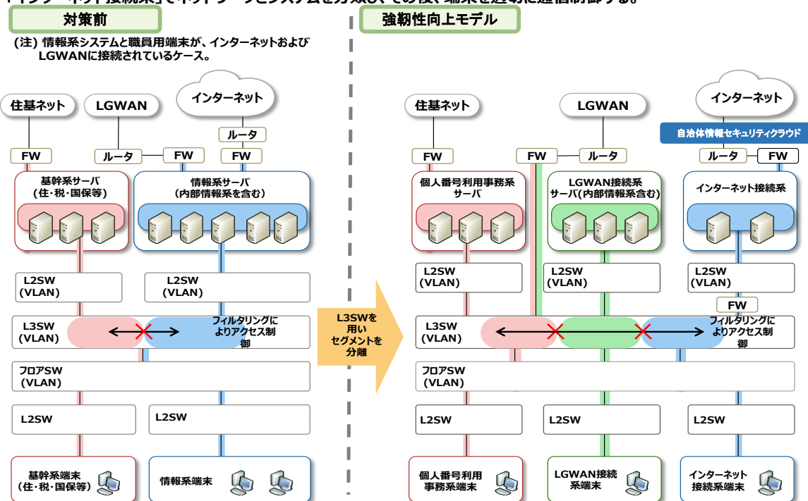
図表 22 強靭性向上モデルにおけるネットワーク再構成のイメージ
