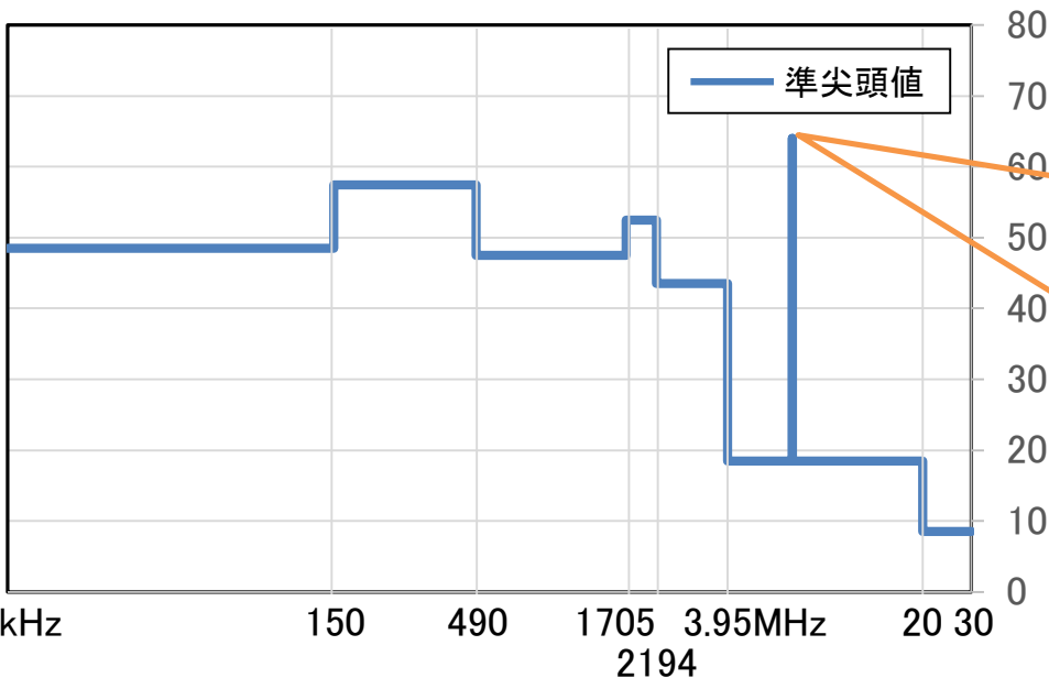
放射妨害波の磁界強度 (dB \mu A/m)
