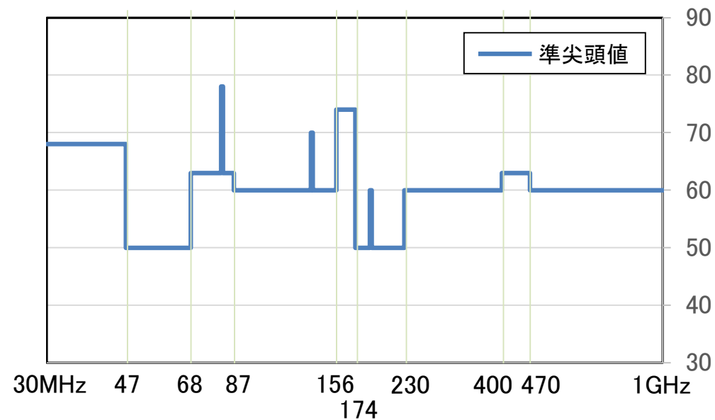
放射妨害波の電界強度 (dB \mu V/m)
