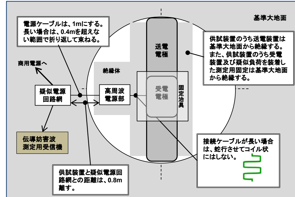
伝導妨害波の測定方法
