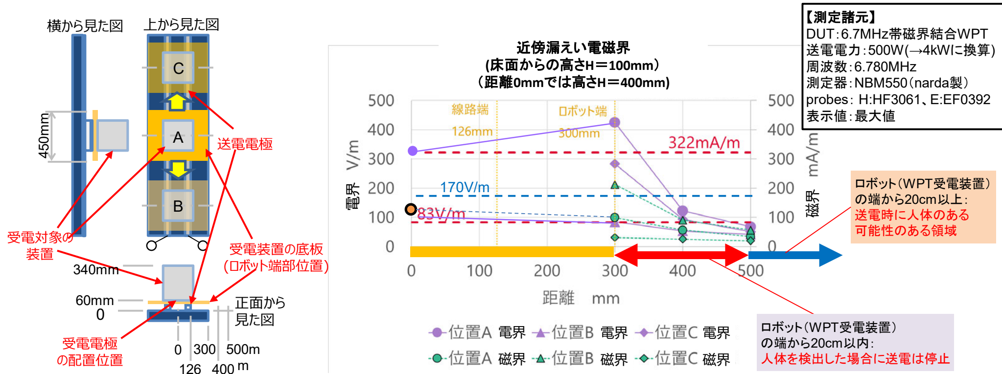
適合性確認のために行った測定装置
