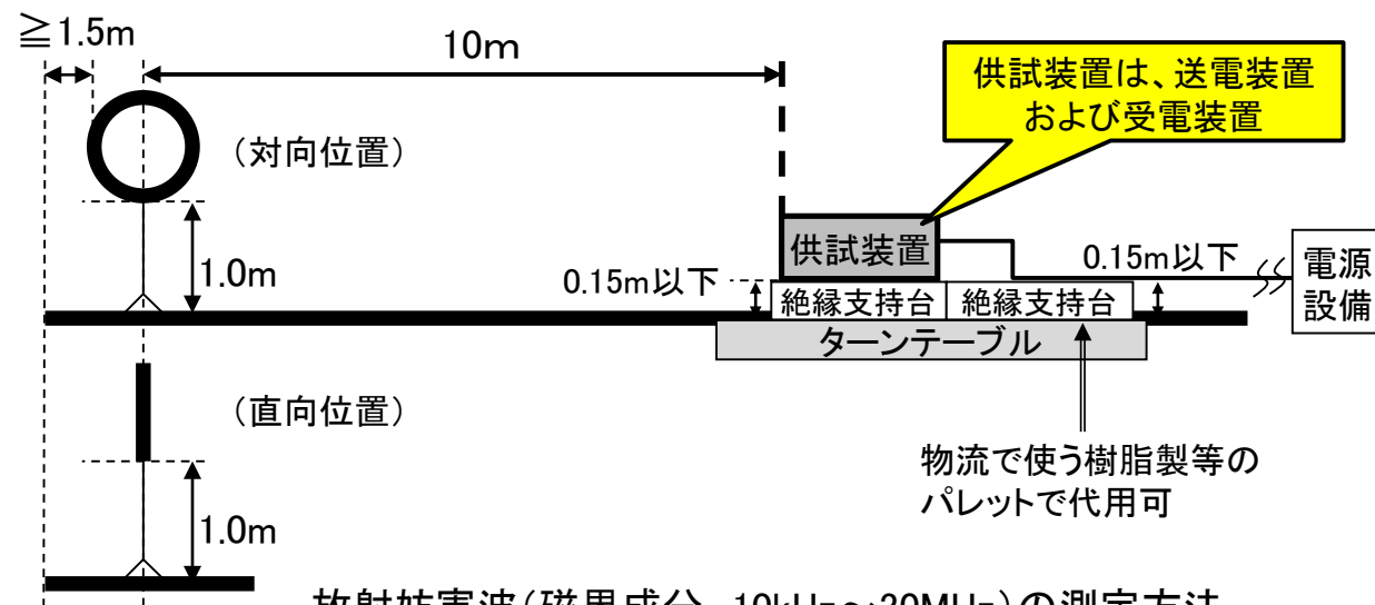
放射妨害波(磁界成分、10kHz~30MHz)の測定方法
