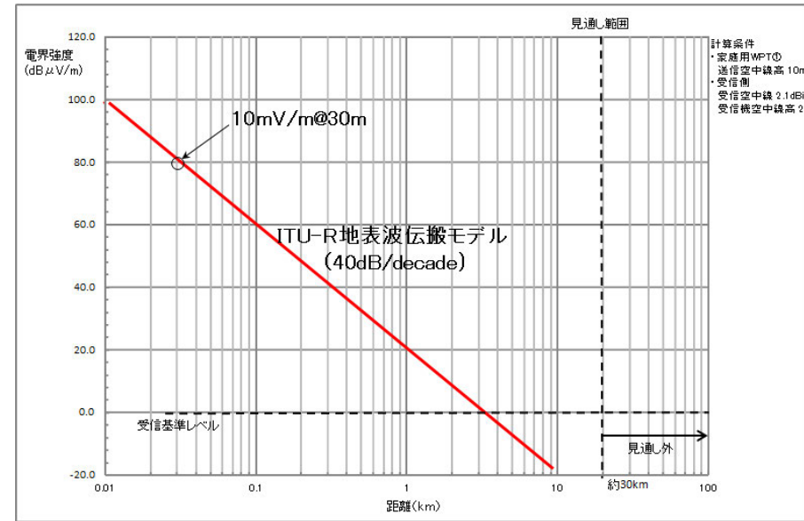
漏えい電界の伝搬特性計算値
