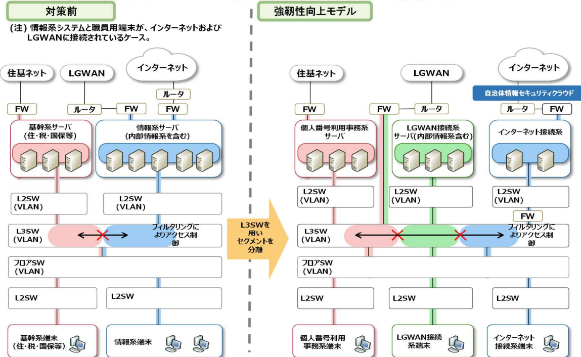
図表 2223 強靱性向上モデルにおけるネットワーク再構成の一つのイメージ
