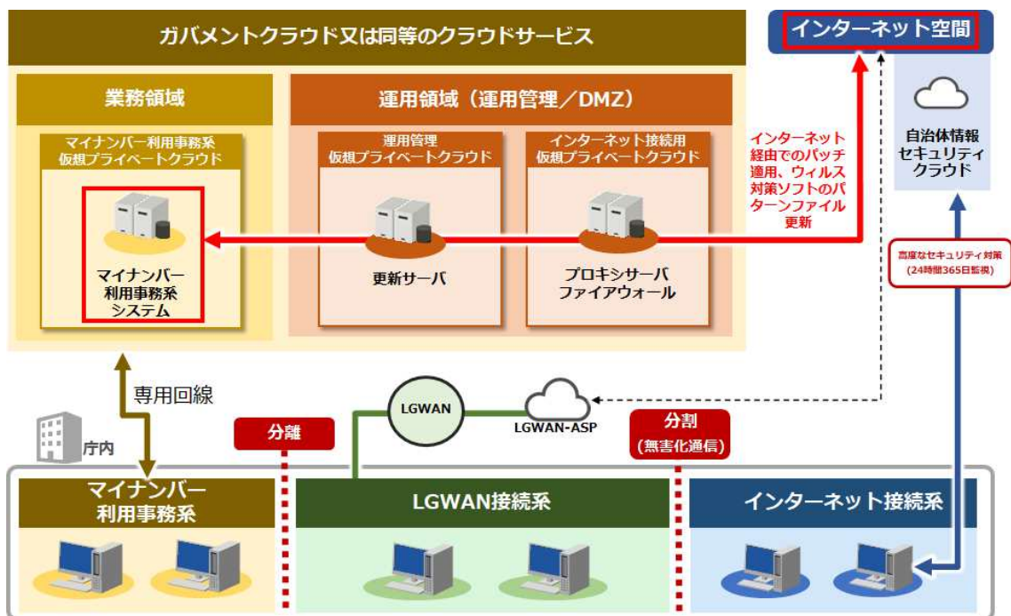
図表 3645 インターネット経由による標準標準拠システム等の修正プログラム適用、ウイルス対策ソフトのパターンファイル更新等のイメージ
