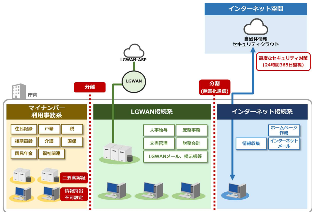
図表 2122 三層の構えによる自治体情報システム例
