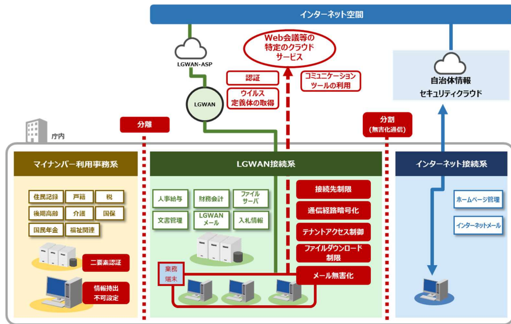
図表 29 α'モデル (コミュニケーションツールを利用するが、ファイルを内部に取り込まない場合) イメージ図
