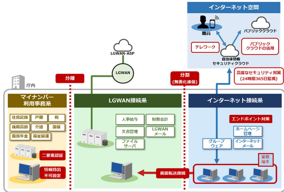
図表 2835 Bモデルイメージ図
