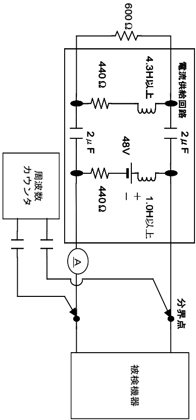
(2) 信号送出時間、ミニムパルス及び周期の測定の場合
