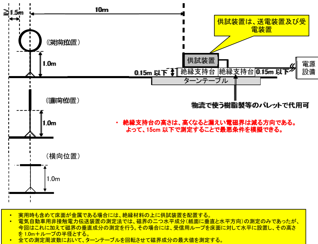
図 4.2-5 放射妨害波（磁界成分、10kHz～30MHz）の測定方法
