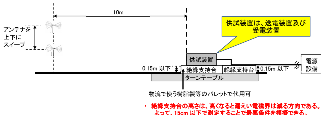
図 3 放射妨害波（電界成分、30MHz～1GHz）の測定方法
