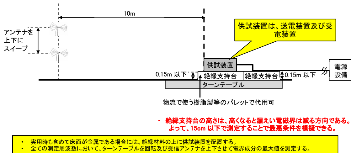
図 4.2-6 放射妨害波（電界成分、30MHz～1GHz）の測定方法
