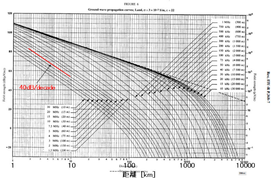
図 3.2-2 ITU-R 勧告 P. 368-7 の地表波の伝搬特性 (大地の定数 導電率: 3mS/m、比誘電率: 22.0)
