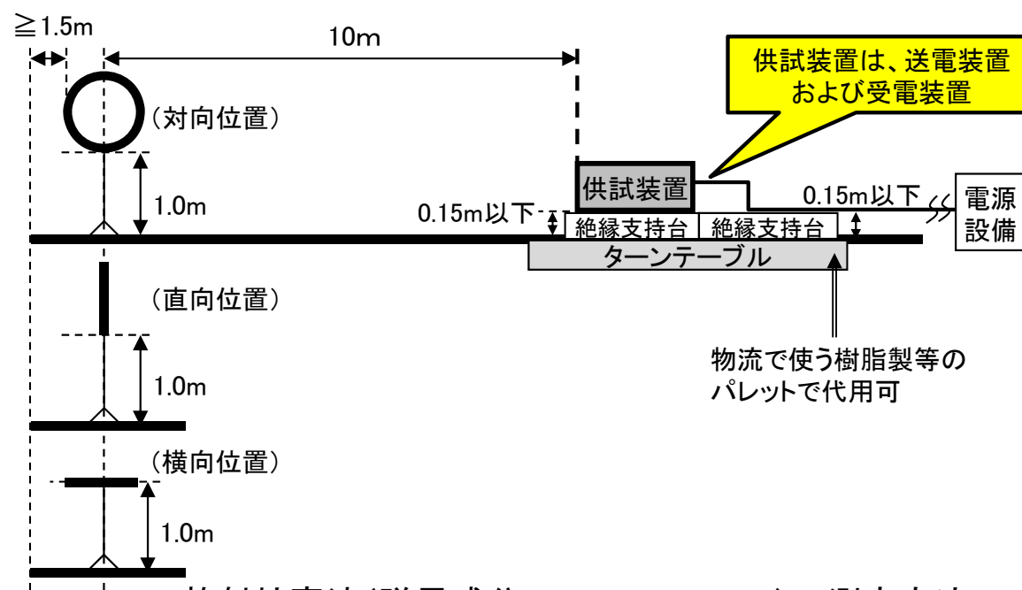
放射妨害波(磁界成分、10kHz~30MHz)の測定方法
