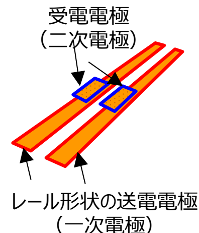
WPTのための送受の電極の構成
