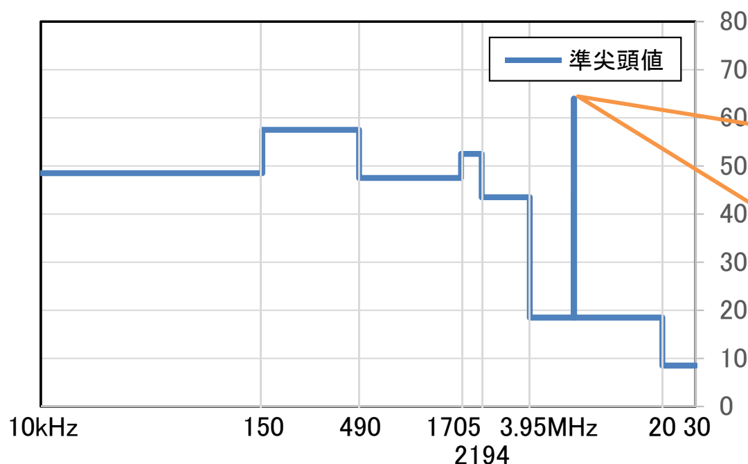
放射妨害波の磁界強度(dB \mu A/m)
