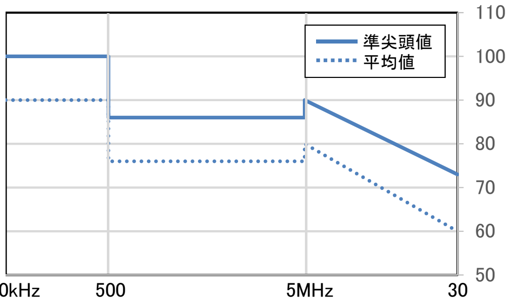
交流電源端子における妨害波電圧(dB \mu V)
