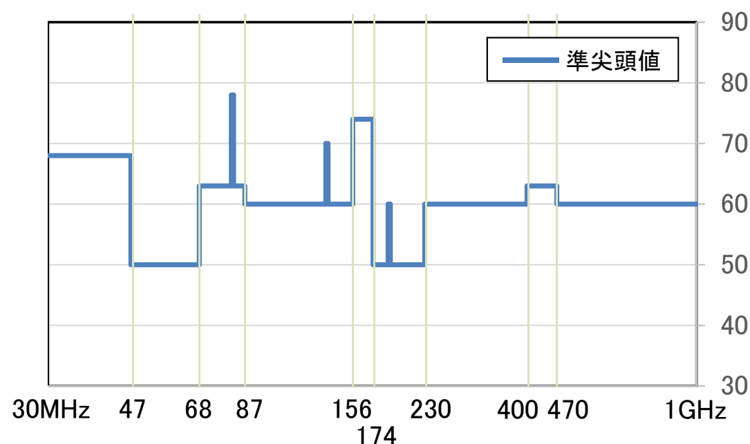
放射妨害波の電界強度(dB \mu V/m)
