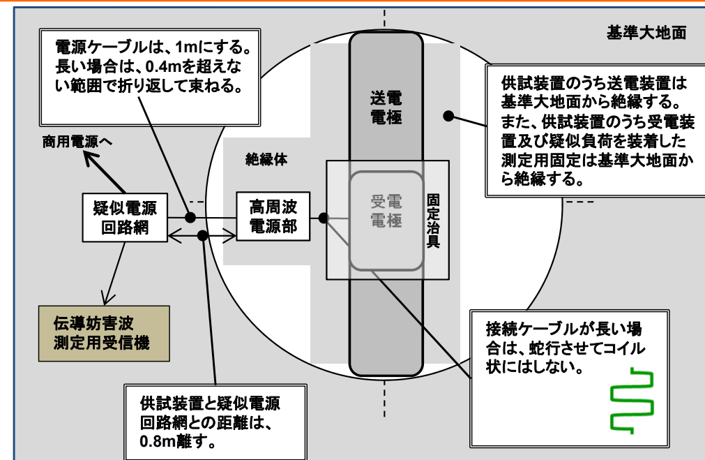
伝導妨害波の測定方法
