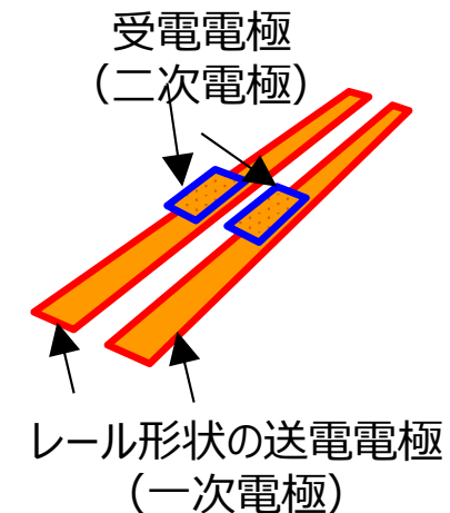
WPTのための送受の電極の構成
