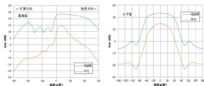
マクロセル基地局空中線指向特性
