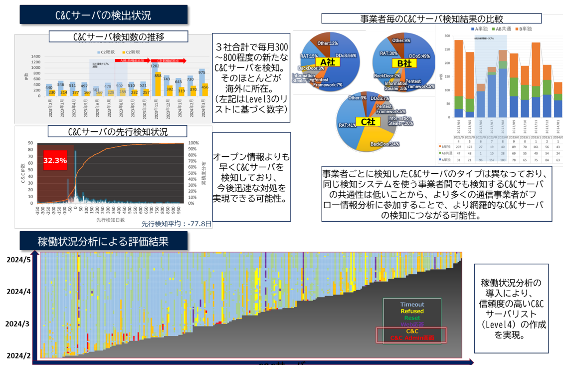
(図 13) フロー情報分析による C&C サーバ検知の成果
