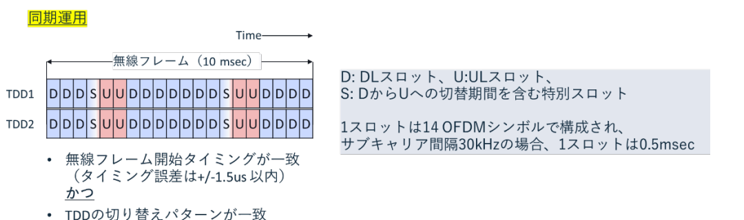
図 2-14 同期運用
