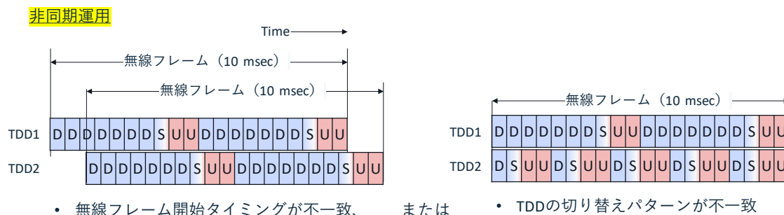
図 2-15 非同期運用
