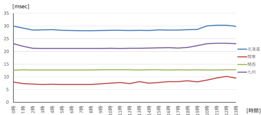
＜図表 2-21＞地方別の遅延(レイテンシー)の推移(IPv4)
