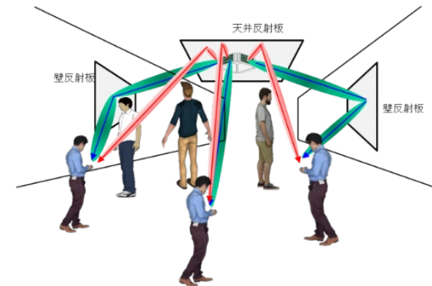
ミリ波・サブテラヘルツ波無線ネットワークの概念
