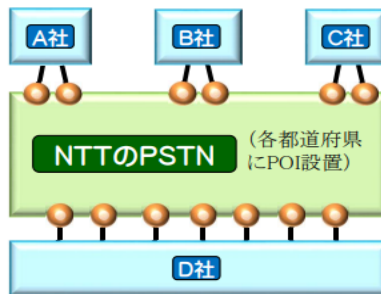
現在の事業者間接続 (イメージ)
