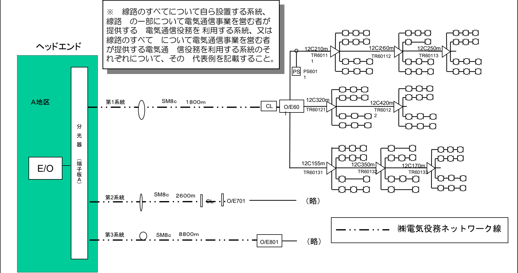
設備系統図(線路の一部について電気通信事業を営む者が提供する電気通信役務を利用する系統の代表例)
