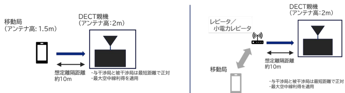
図 2. 6. 2-2 2GHz 帯非静止衛星通信システム（移動局）からデジタルコードレス電話システム（DECT 方式親機）への与干渉の 1 対 1 対向モデル
