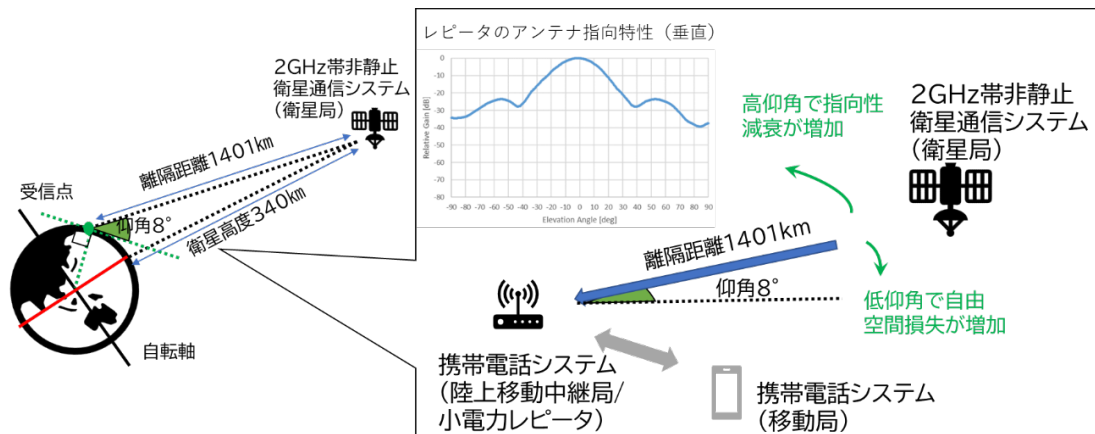
図2.3.2-3 2GHz帯非静止衛星通信システム（衛星局）から移動通信システム（移動局：陸上移動中継局（屋外型））への与干渉の実運用モデル
