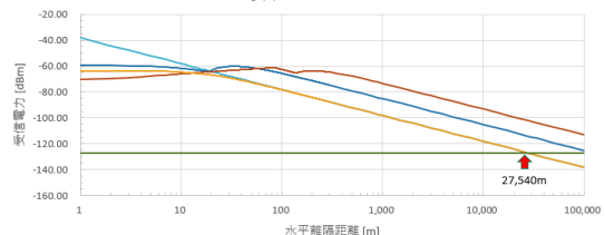
参考図2-8 RKE E.I.R.P.: 0dBm
