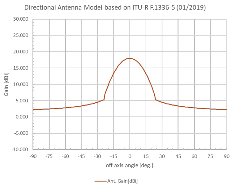
参図 2-36 八木アンテナのアンテナモデル (15 エレ) (Gain: 18dBi, HPBA: 24deg)
