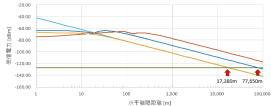
参考図2-4 TPMS E.I.R.P.: 0dBm
