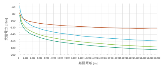
参図2-19 RKE E.I.R.P.: 0dBm
