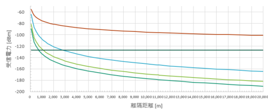
参図2-16 RKE E.I.R.P.: 0dBm
