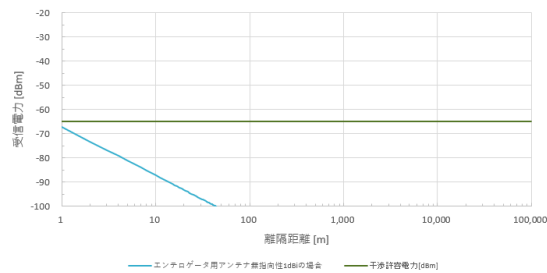
参考図2-30 自由空間損失のみ RKE 帯域外 -36.02dBm/100kHz (-43.01dBm/20kHz)
