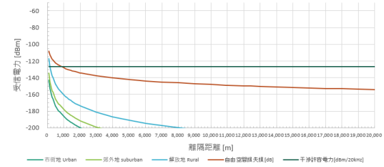
参图2-15 RKE 带域外实力值 -65.0dBm/20kHz
