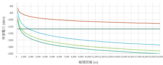
参図2-17 RKE E.I.R.P.: -10dBm
