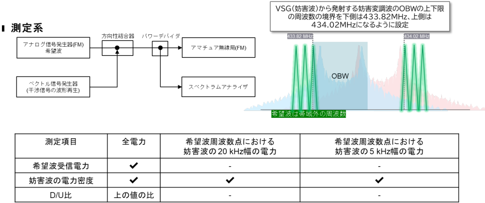
参照 5-10 帯域外における所要 D/U 比の測定に係る測定系等
