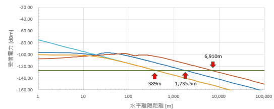
参照2-6 TPMS帯域外 -36.02dBm/100kHz (-43.01dBm/20kHz)
