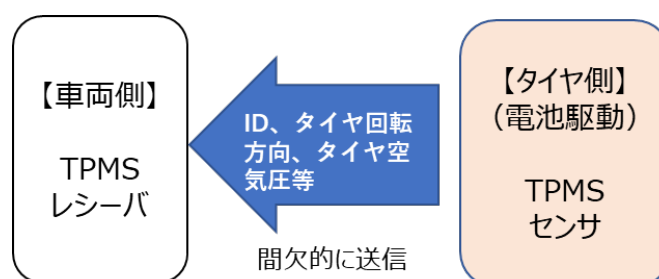
図 2. 1. 2-1 TPMS の通信
