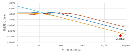
参照2-4 TPMS E.I.R.P.: 0dBm
