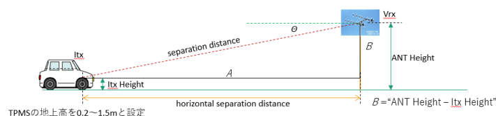
参照2-7 シミュレーションモデル
