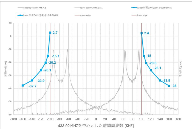
参照 5-11 干渉信号の OBW の境界を BN の境界に配置した場合の帯域外領域において D/U 比を測定した結果（2 値 FSK（RKE1））
