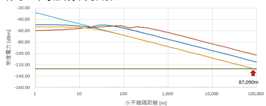
参照2-8 RKE E.I.R.P.: 0dBm
