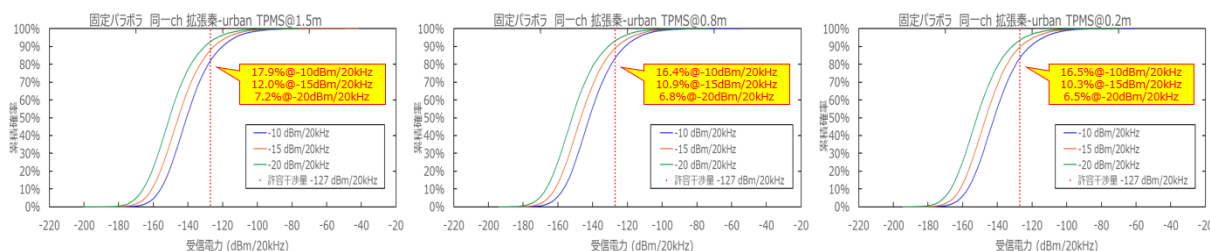
参図 4-5 TPMS からアマチュア局（固定・パラボラ）への干渉発生確率 （同一帯域利用、普及予測パターン2）
