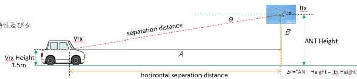
参考図2-32 シミュレーションモデル
