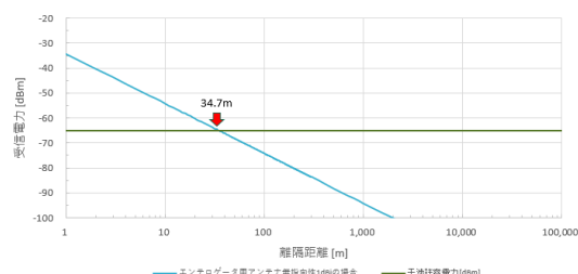
参図2-26 自由空間損失のみ TPMS E.I.R.P.: -10dBm
