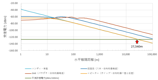
参照2-9 RKE E.I.R.P.: -10dBm
