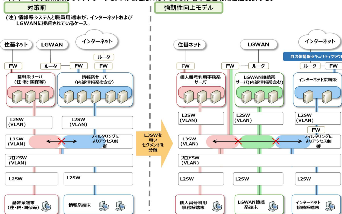
図表 26 強靱性向上モデルにおけるネットワーク再構成のイメージ
