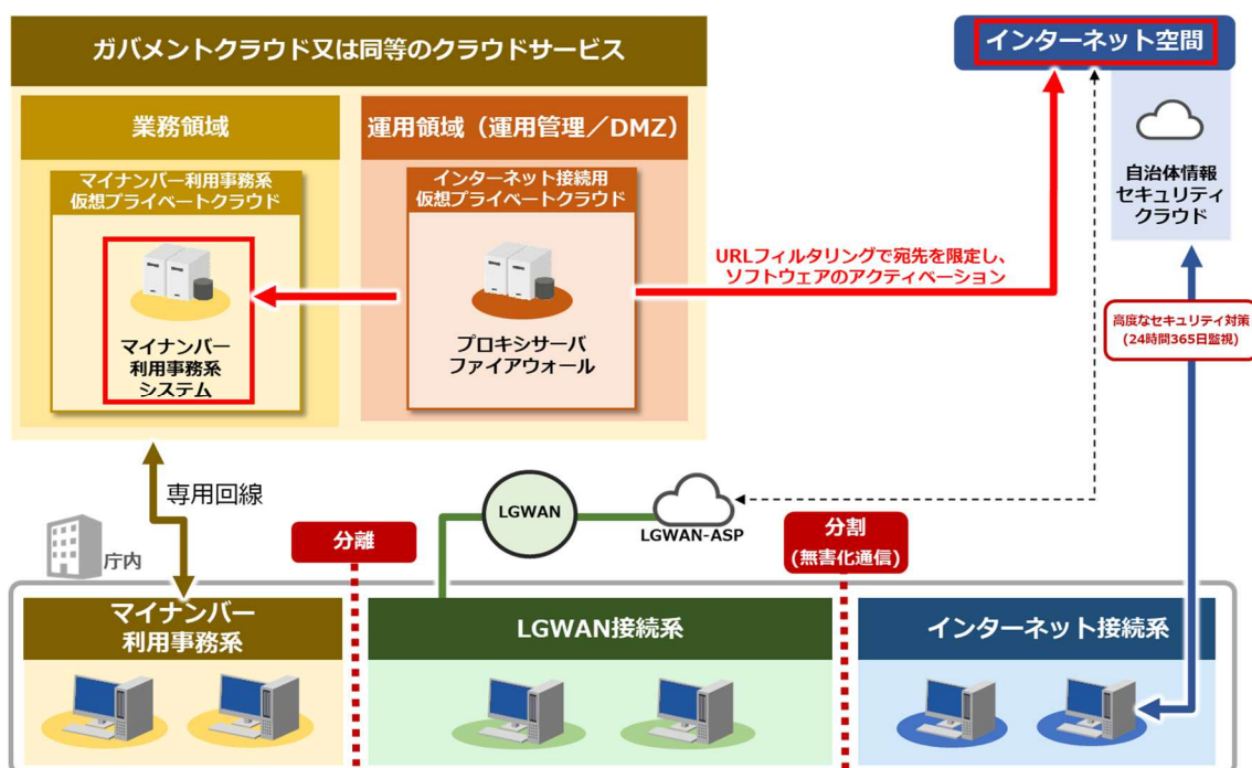
図表 51 インターネット経由での標準準拠システム等のソフトウェアのアクティベーションを実施する場合のイメージ
