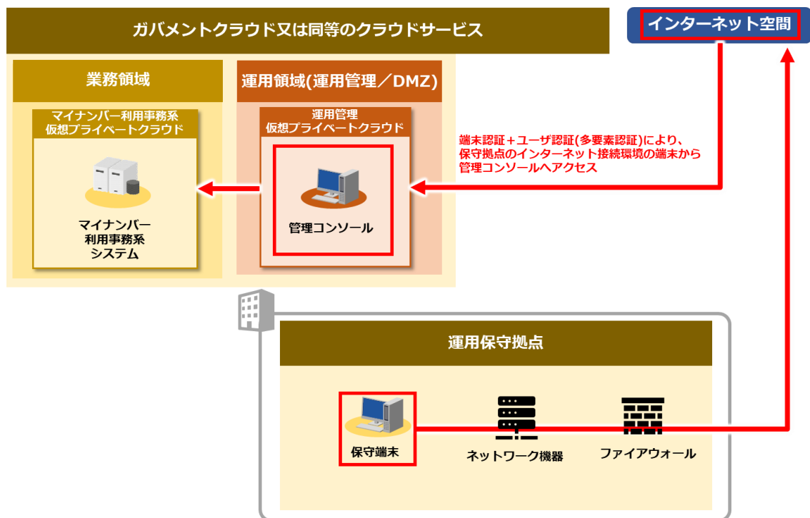
図表 52 インターネット経由での標準準拠システム等の運用保守（管理コンソール接続）を実施する場合の接続イメージ
