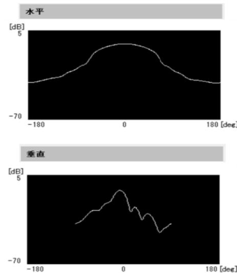
図1 HPUE(PC1)アンテナパターン
