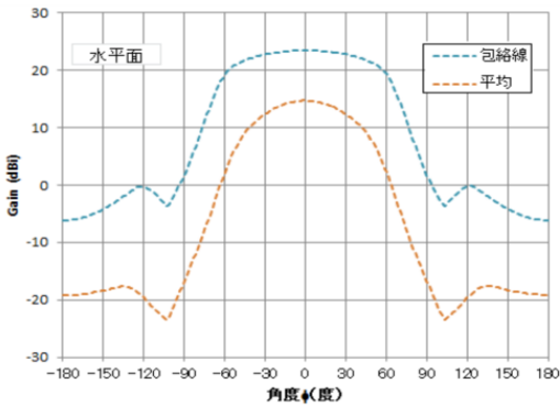
図1 L5G基地局（マクロセル局）のアンテナパターン（左：水平、右：垂直）
