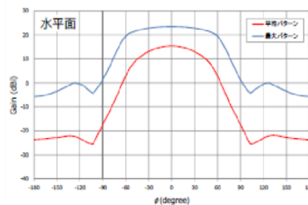
図3 mmW帯NR基地局アンテナパターン(左:水平、右:垂直)
