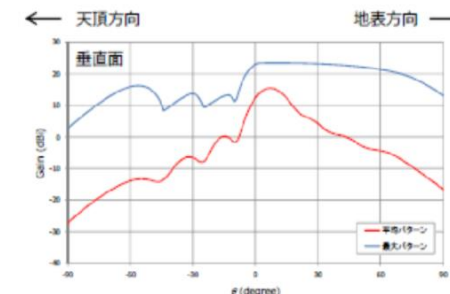
図3 mmW帯NR基地局アンテナパターン(左:水平、右:垂直)
