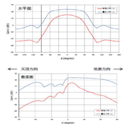
図2 L5G基地局アンテナパターン (上:水平、下:垂直)
