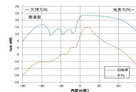
図2 Sub6帯NR基地局のアンテナパターン(左:水平、右:垂直)
