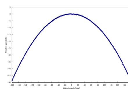
図1 BWA帯、Sub6帯基地局のアンテナパターン(左:水平、右:垂直)
