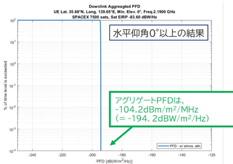
図2. 5. 2-2 アグリゲート PFD の検証の結果（水平仰角 0° 以上）
