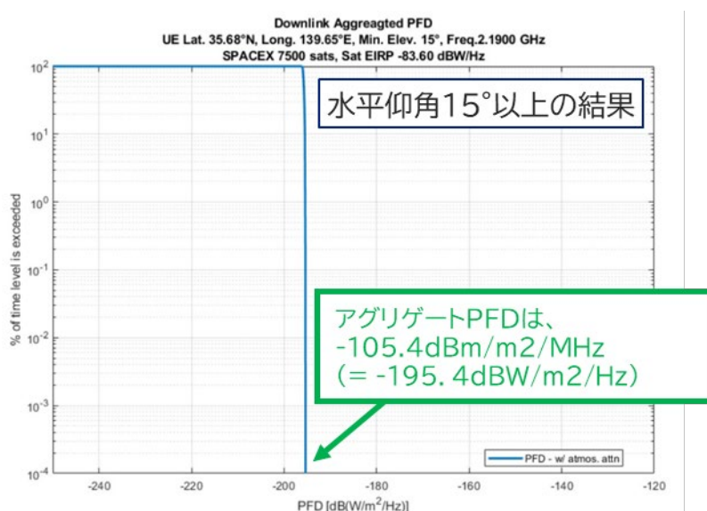
図 2. 5. 2-1 アグリゲート PFD の検証の結果（水平仰角 15° 以上）
