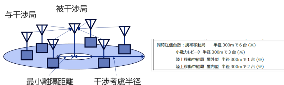
図 2. 6. 2-7 検討モデル
